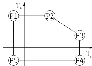
▣ 43 铝外壳, 带涂层; 过程温度范围: -40 ... +150 °C (-40 ... +302 °F)
