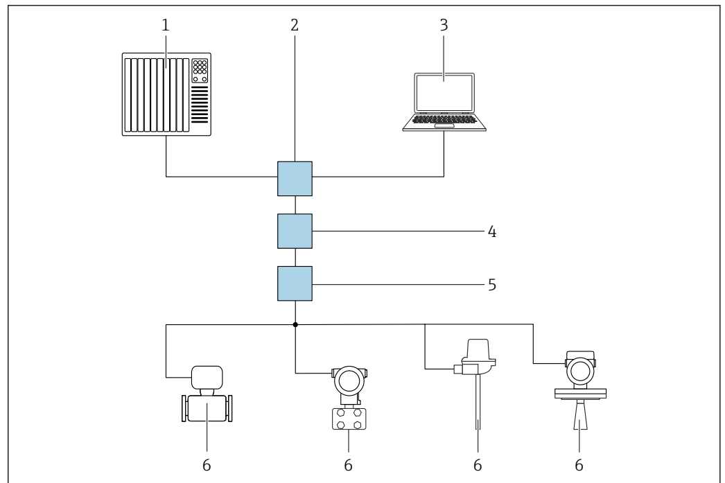
图 18 通过 PROFINET + Ethernet-APL 网络实现远程操作：星形拓扑结构
