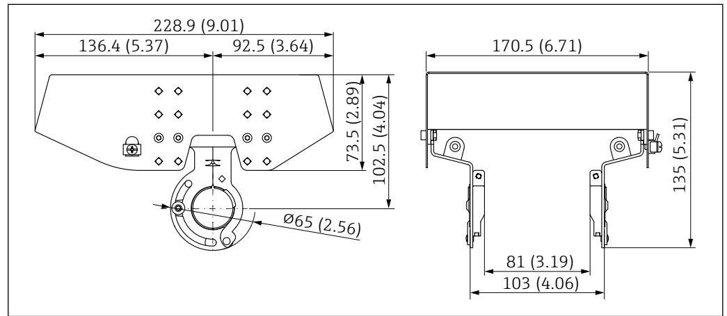
图 27 316L 防护罩 XW112 的外形尺寸示意图。测量单位 mm (in)
