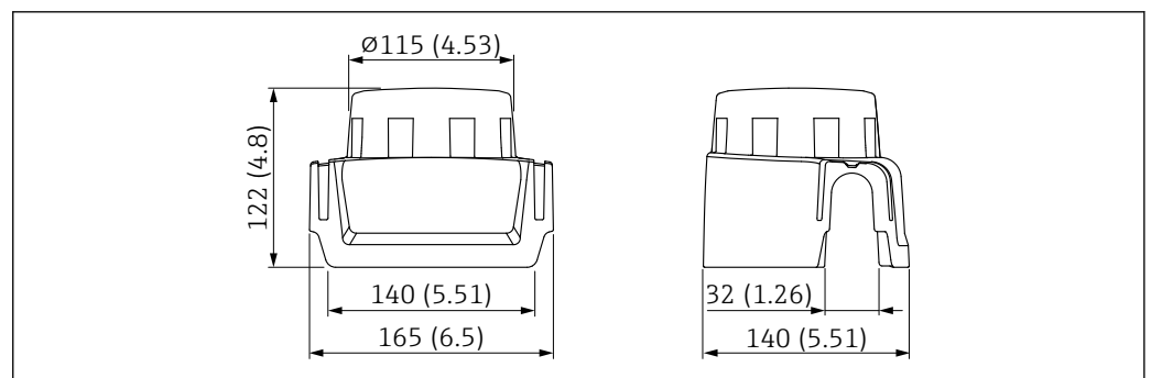
图 28 塑料防护罩 XW111 的外形尺寸示意图。测量单位 mm (in)
