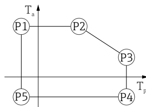
☑ 34 塑料外壳; 过程温度范围: -40 ... +150 °C (-40 ... +302 °F)
