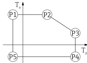
▣ 36 塑料外壳; 过程温度范围: -40 ... +200 °C (-40 ... +392 °F)
