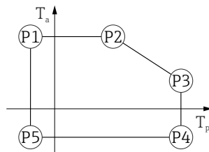
▣ 45 铝外壳, 带涂层; 过程温度: -40 ... +280 °C (-40 ... +536 °F)
