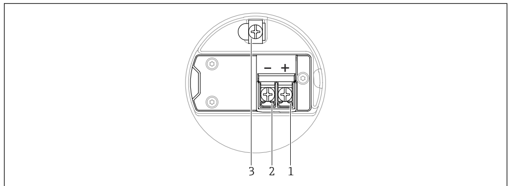
图 8 接线腔中的接线端子和接地端
