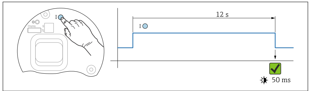
图 26 时序图 - 恢复出厂设置
