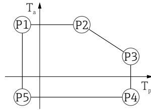
图 47 316L 外壳; 过程温度范围: -40 ... +80 °C (-40 ... +176 °F)
