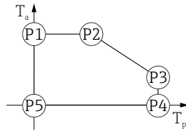
▣ 41 塑料外壳; 过程温度: 0 ... +450 °C (+32 ... +842 °F), 针对 CSA C/US 认证型仪表
