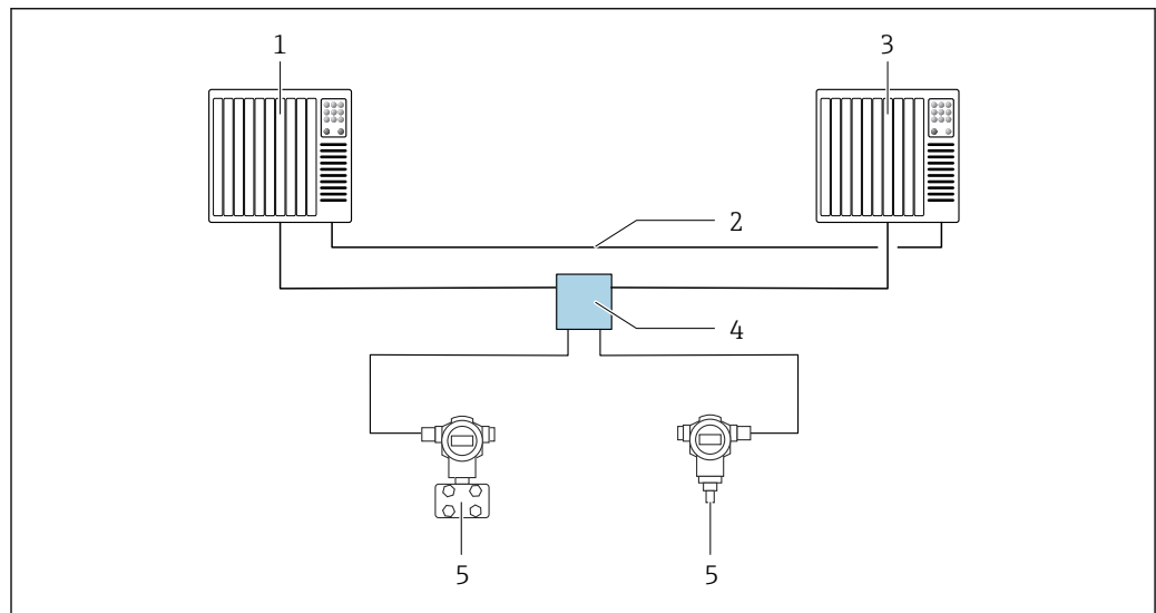
图 19 S2 系统冗余布局实例：星形拓扑结构
