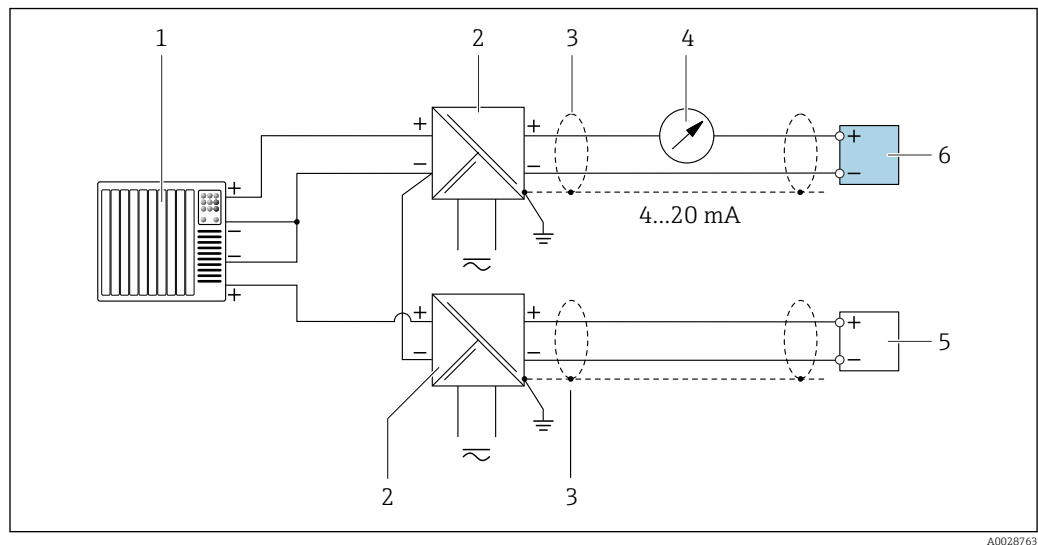
14 Ejemplo de conexión de una entrada HART con negativo común (pasivo)
