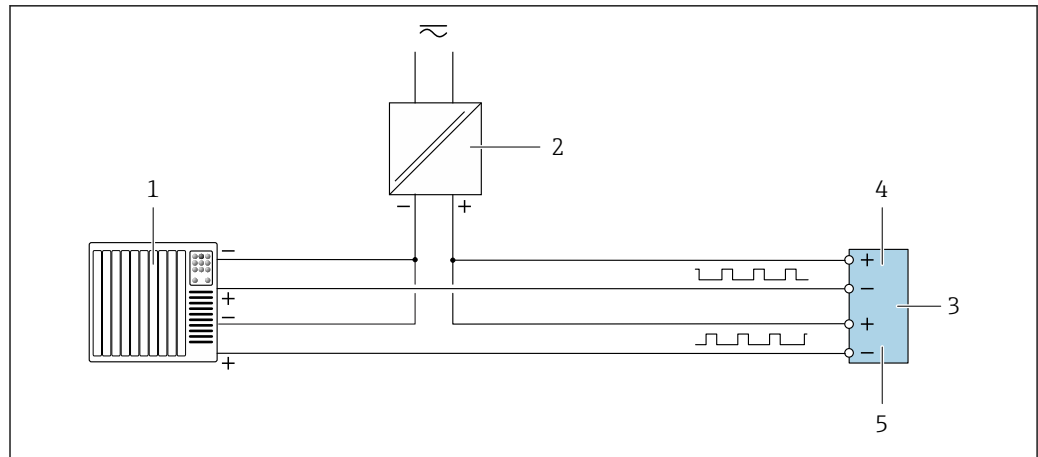
20 Ejemplo de conexión de una doble salida de pulsos (pasiva)
