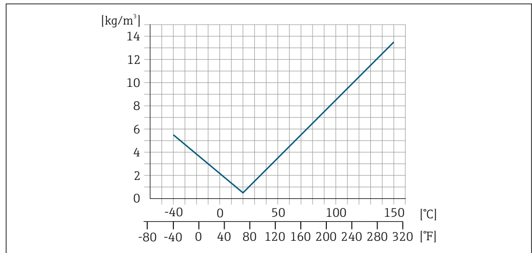
39 Ajuste en campo de la densidad, p. ej., a +20 \text{ }^\circ\text{C} ( +68 \text{ }^\circ\text{F} )
