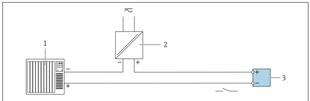
☑ 21 接线实例：继电器输出（无源信号）
