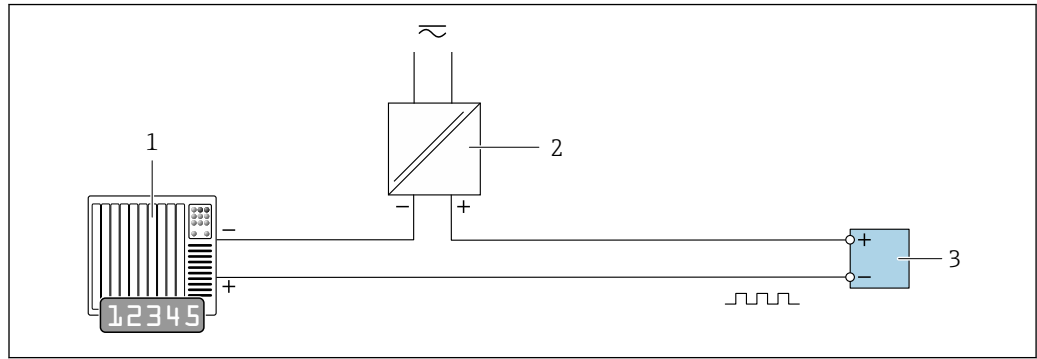
图 17 接线示例：脉冲/频率输出（无源信号）
