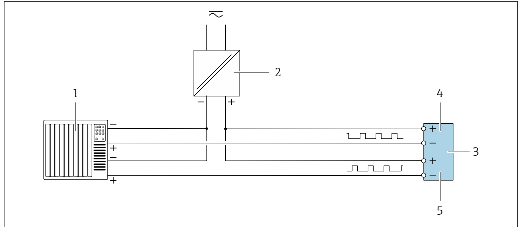
☑ 20 接线实例：双脉冲输出（无源信号）
