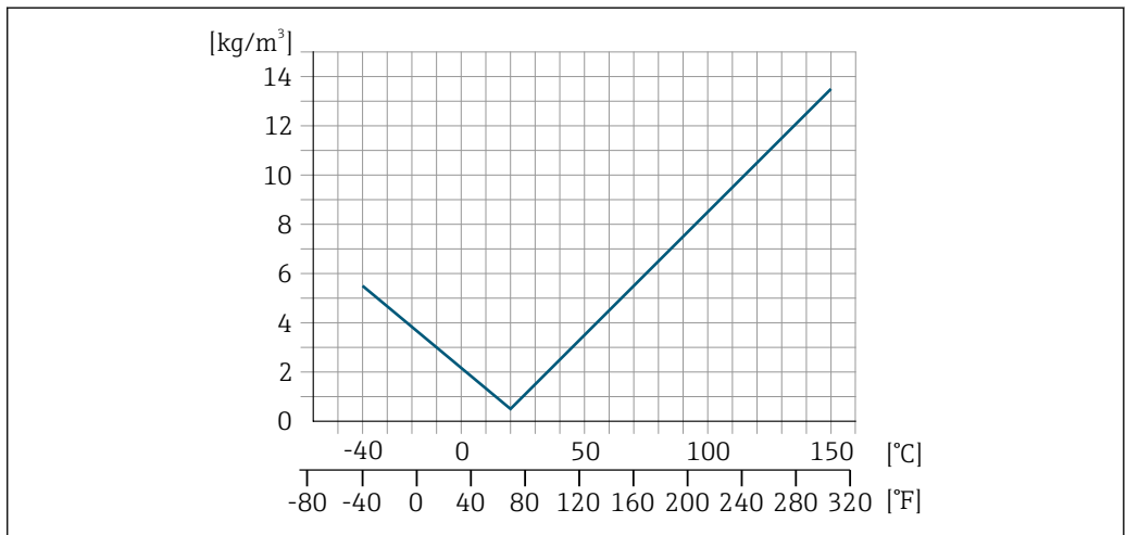
图 39 现场密度校正，例如在 +20 \text{ }^\circ\text{C} ( +68 \text{ }^\circ\text{F} ) 时
