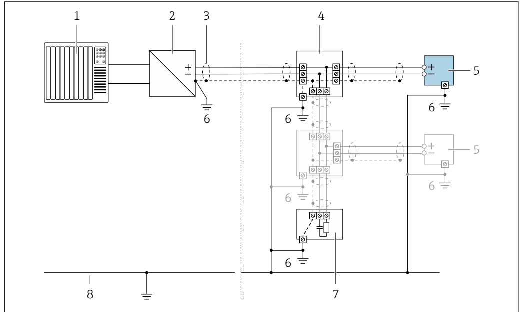
13 Exemple de raccordement pour PROFIBUS PA
