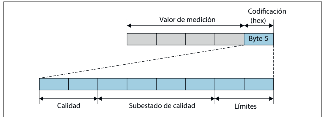
32 Estructura del byte de codificación
