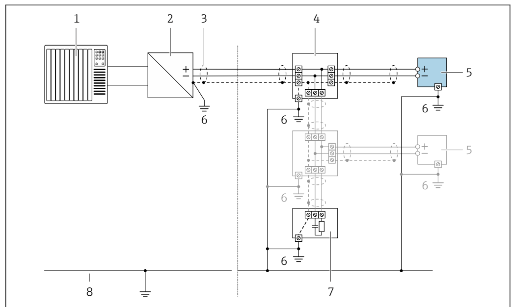
11 Ejemplo de conexión para PROFIBUS PA
