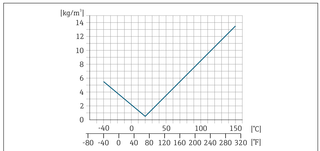
図 43 現場密度調整、例：+20 °C (+68 °F) 時
