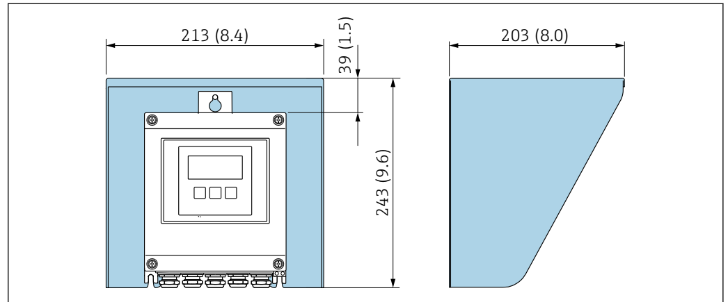
図 10 Proline 500 - デジタル用の日除けカバー、工学単位 mm (in)
