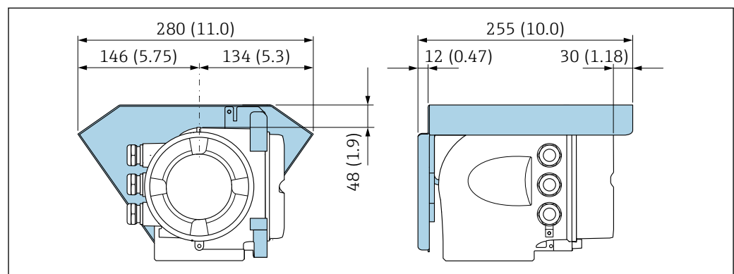
図 11 Proline 500 用の日除けカバー、工学単位 mm (in)
