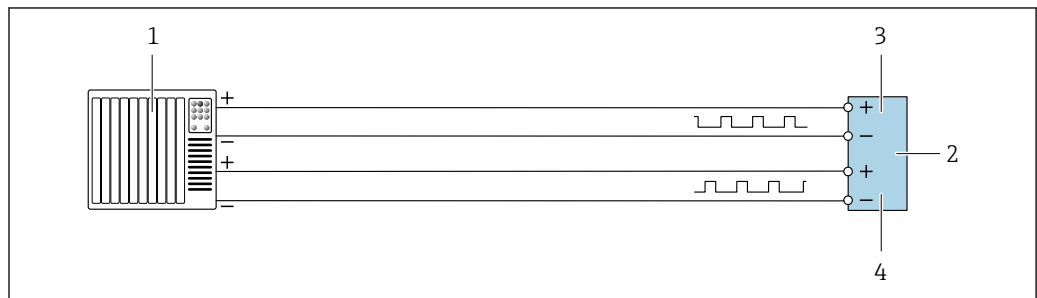
図 26 ダブルパルス出力（アクティブ）の接続例
