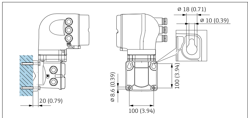
図 14 工学単位 mm (in)
