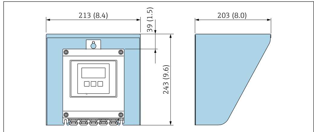
図 10 Proline 500 - デジタル用の日除けカバー、工学単位 mm (in)
