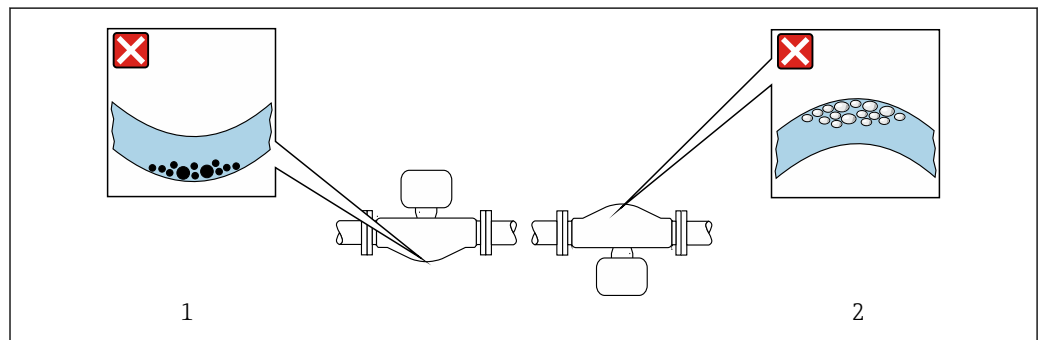
8 弓形計測チューブセンサの取付方向
