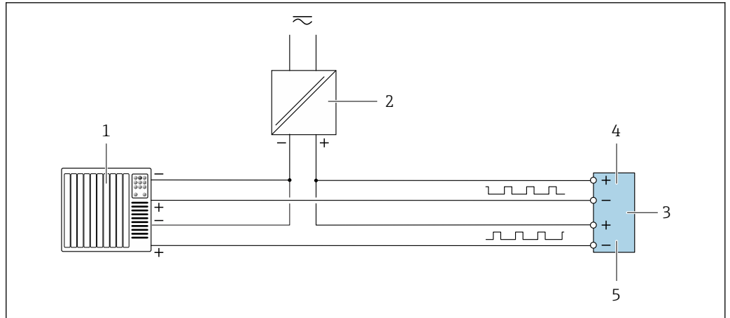
図 27 ダブルパルス出力（パッシブ）の接続例
