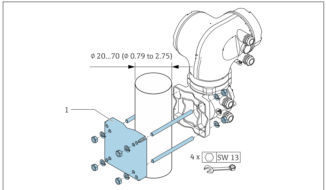
図 15 工学単位 mm (in)
