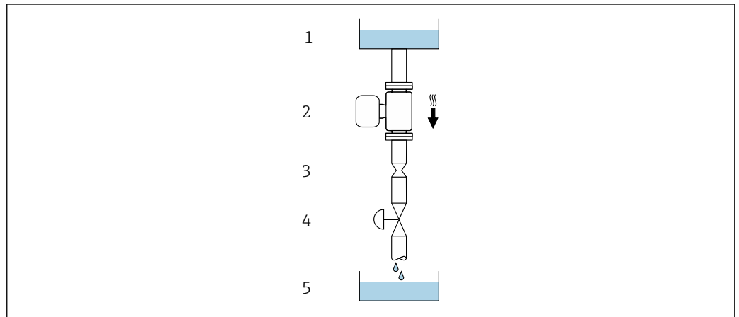
図 7 下り配管への設置（例：パッチアプリケーション用）
