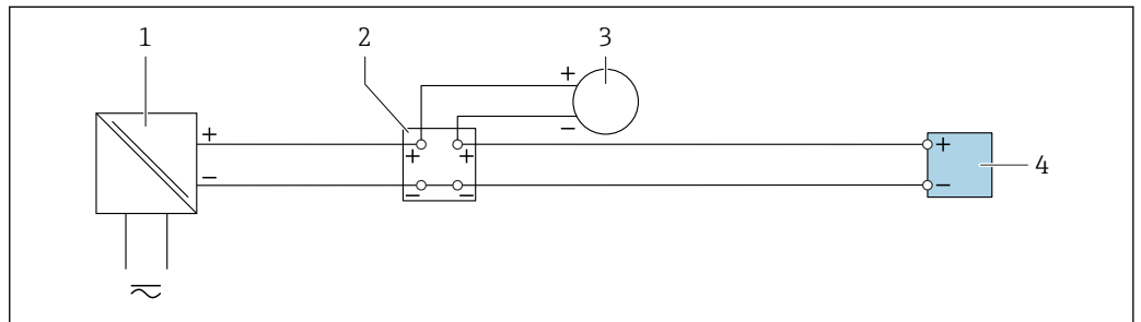
図 29 4~20 mA 電流入力の接続例
