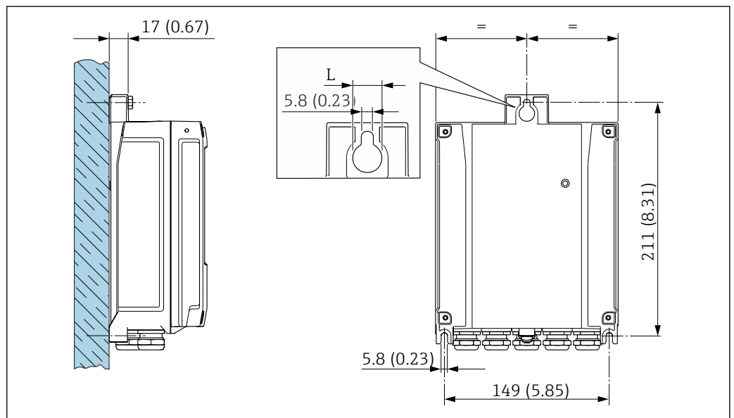
図 13 工学単位 mm (in)
