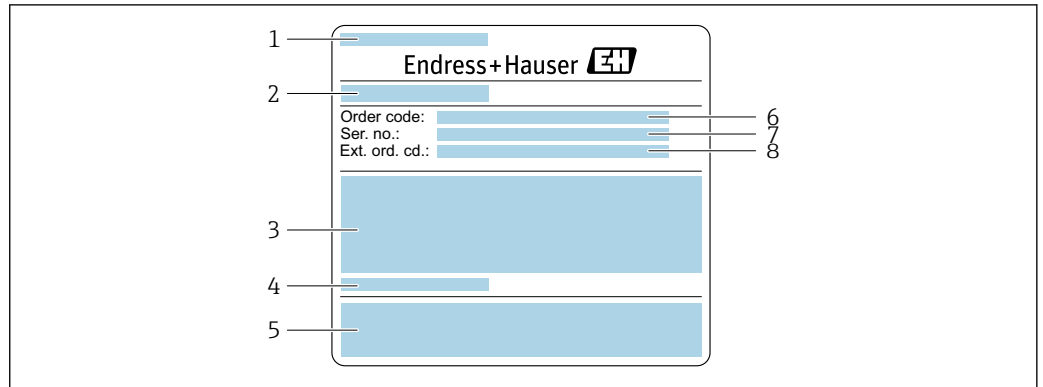
図 5 センサ銘板の例、第 1 部
