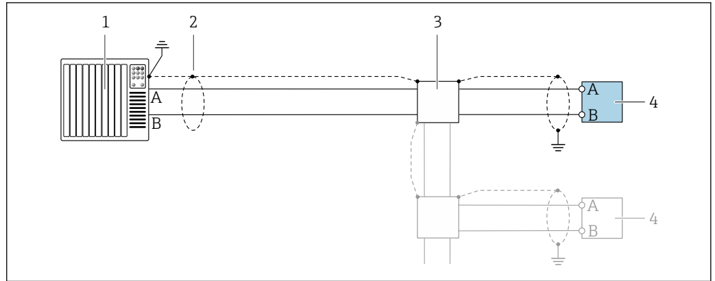
図 19 Modbus RS485（非危険場所および Zone 2; Class I, Division 2 用）の接続例
