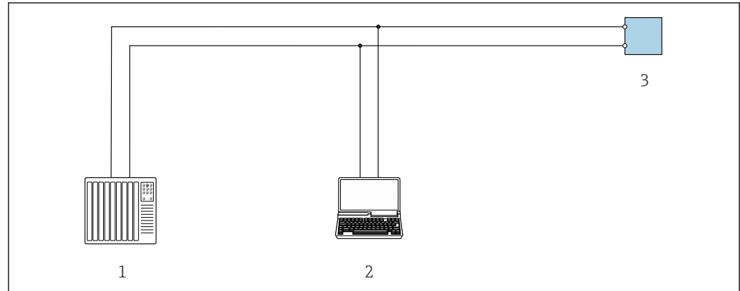
図 33 Modbus RS485 プロトコル経由のリモート操作オプション (アクティブ)
