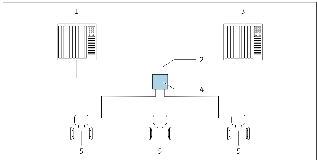
図 25 冗長システム (S2) のレイアウト例：スター型トポロジー
