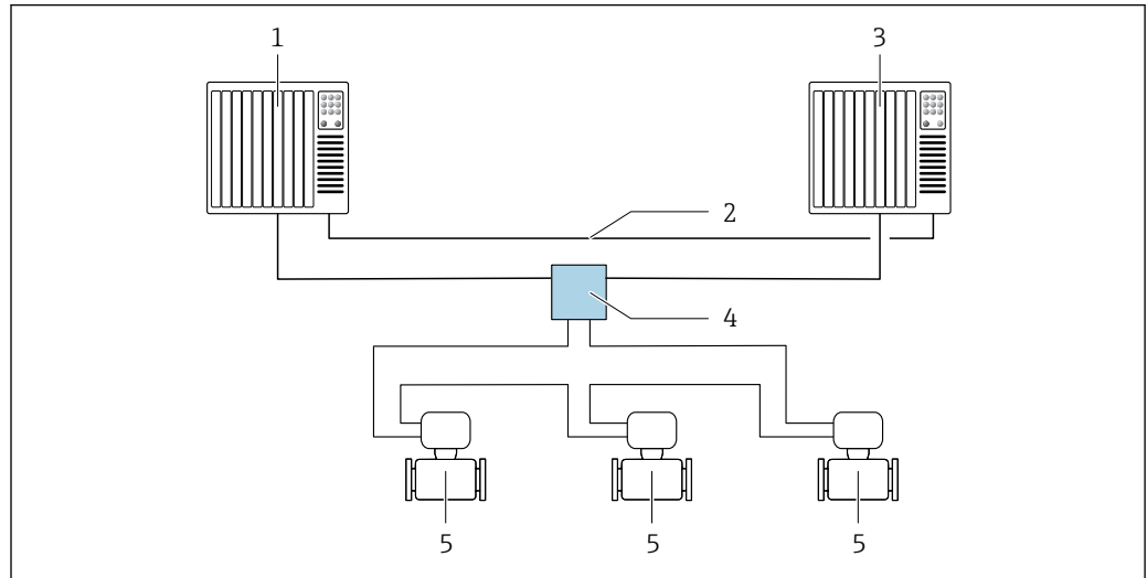
図 24 冗長システム (S2) のレイアウト例：リングトポロジー
