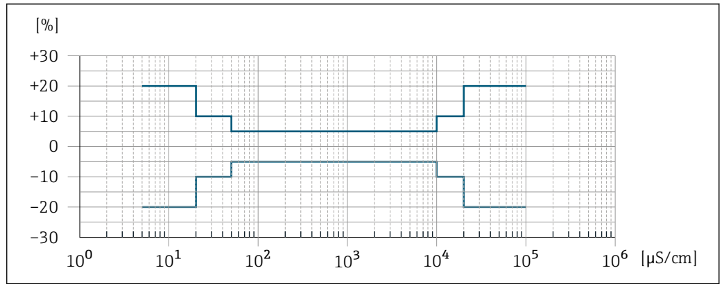
図 47 測定誤差 (オプション:「校正済導電率測定」のオーダーコード、オプション CW)
