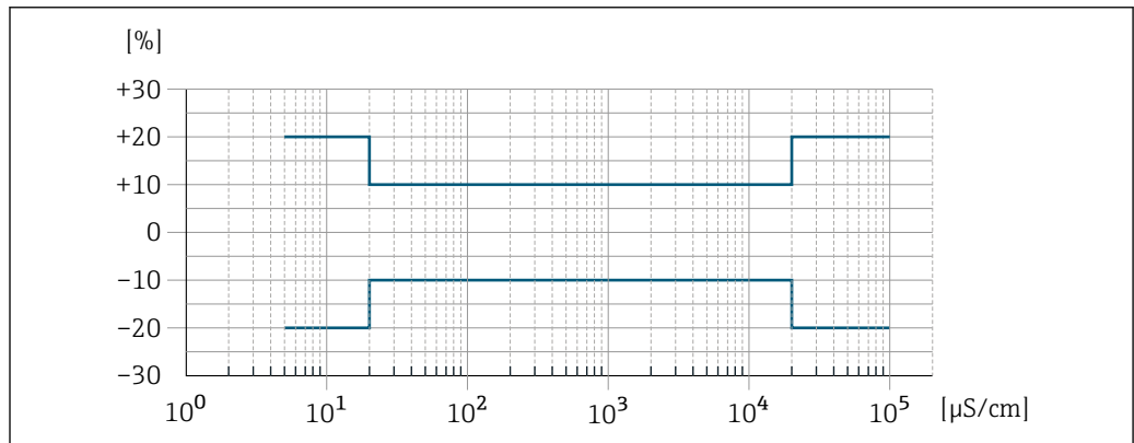
図 46 測定誤差 (標準)
