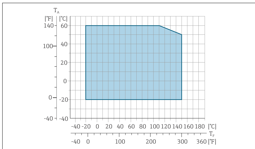
図 48 Promag 500 – デジタル
