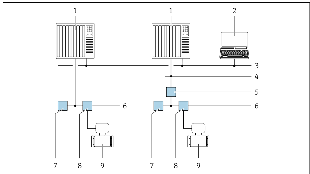
図 31 FOUNDATION フィールドバスネットワークを介したリモート操作用のオプション
