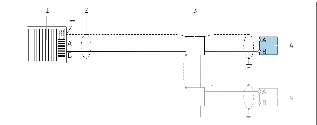
図 18 Modbus RS485（非危険場所およびゾーン 2/Div. 2 用）の接続例
