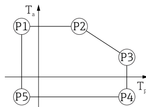
図 27 プラスチックハウジング ; プロセス温度 -40\sim+150\text{ }^{\circ}\text{C} ( -40\sim+302\text{ }^{\circ}\text{F} )
