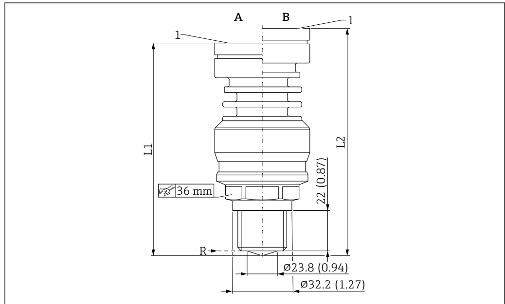
図 65 寸法；内蔵アンテナ、PEEK、20 mm (0.75 in)；プロセス接続、ネジ 3/4"。測定単位 mm (in)
