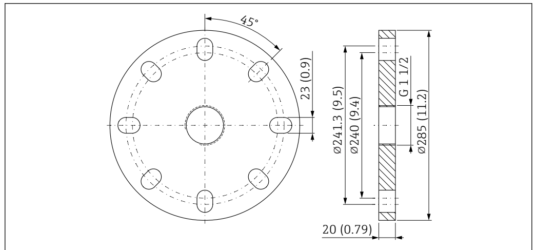
図 64 UNI フランジ 6"/DN150/150A の寸法。測定単位 mm (in)
