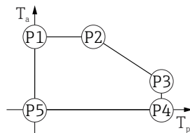
図 26 プラスチックハウジング ; プロセス温度 0\sim+130\text{ }^{\circ}\text{C} ( +32\sim+266\text{ }^{\circ}\text{F} )、CSA C/US 認定取得
