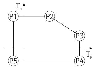
図 21 プラスチックハウジング ; プロセス温度 -20 \sim +200 \text{ }^{\circ}\text{C} ( -4 \sim +392 \text{ }^{\circ}\text{F} )
