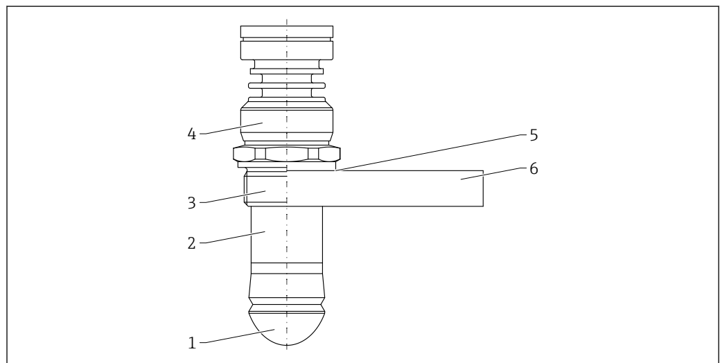
図 68 材質；ドリップオフアンテナ 50 mm (2 in)
