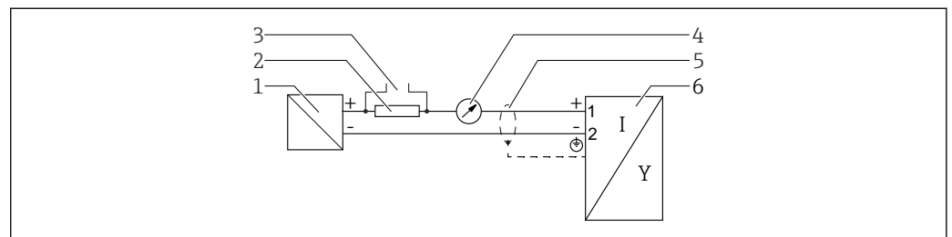
☑ 12 機能図 4~20 mA HART
