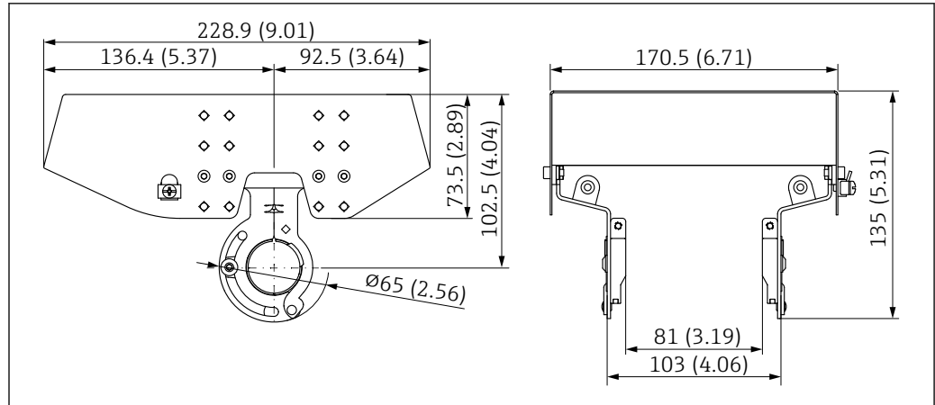
図 73 日除けカバー、SUS 316L 相当、XW112 の寸法。測定単位 mm (in)
