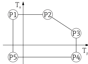
☐ 37 SUS 316L 相当製ハウジング ; プロセス温度 -20~+150 °C (-4~+302 °F)
