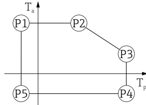
図 19 プラスチックハウジング ; プロセス温度 -20 \sim +150 \text{ }^{\circ}\text{C} ( -4 \sim +302 \text{ }^{\circ}\text{F} )
