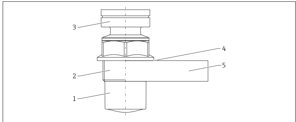
図 67 材質；被覆アンテナ PVDF、40 mm (1.5 in)
