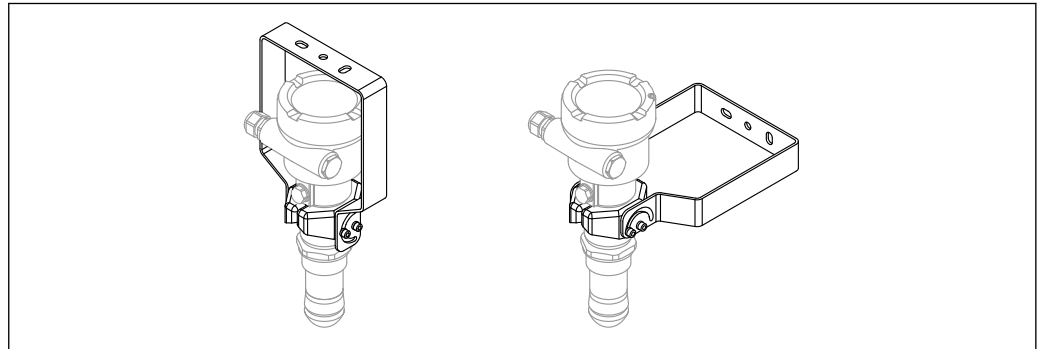
図 75 調整可能な取付ブラケット FMR6xB ; 天井または壁面取付け
