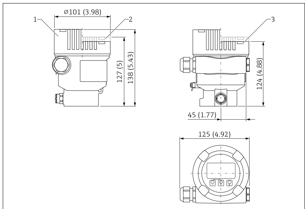
図 50 寸法 ; シングルコンパートメントハウジング (アルミニウム、コーティング) ; M20 カップリングおよびプラグ (プラスチック) 付き。測定単位 mm (in)
