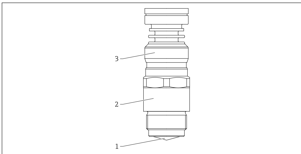
図 70 材質；内蔵アンテナ、40 mm (1.5 in)
