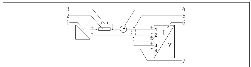
☑ 13 4~20 mA HART、スイッチ出力の機能図
