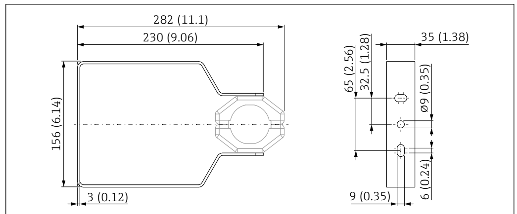
図 76 寸法 ; 調整可能な取付ブラケット FMR6xB。測定単位 mm (in)
