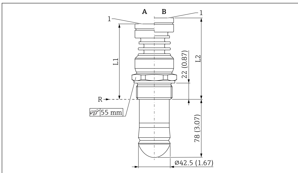
図 60 ドリッポフアンテナ 50 mm (2 in) (ネジ込みプロセス接続) の寸法
