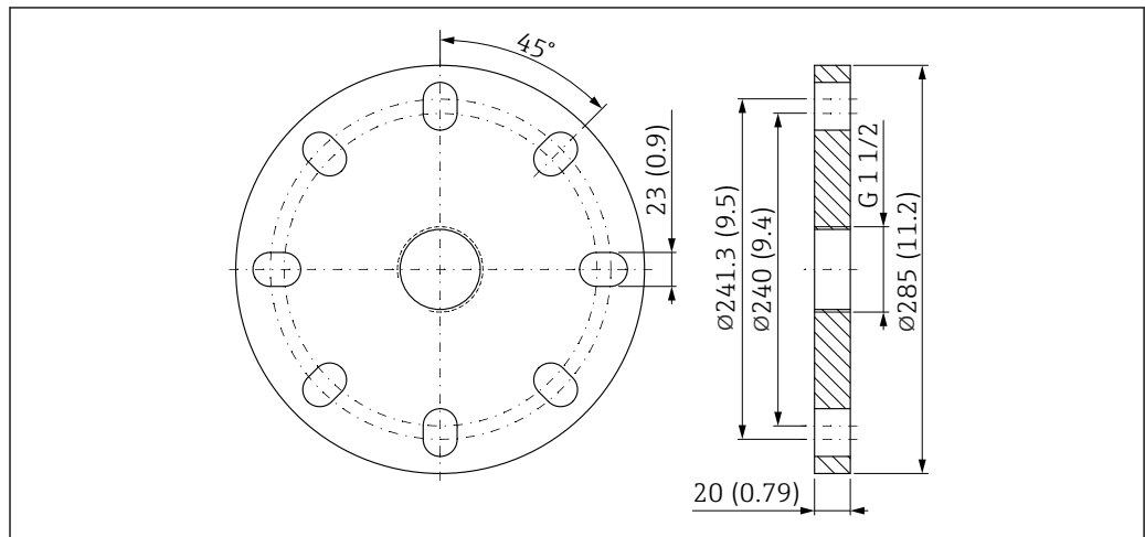
図 59 UNI フランジ 6"/DN150/150A の寸法。測定単位 mm (in)
