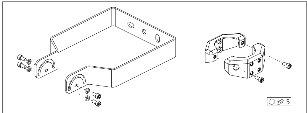
■ 77 納入範囲；調整可能な取付ブラケット FMR6xB
