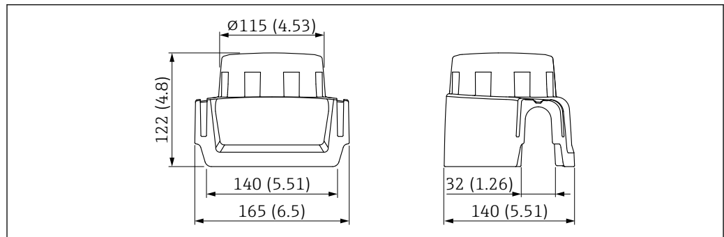
図 74 日除けカバー、プラスチック、XW111 の寸法。測定単位 mm (in)
