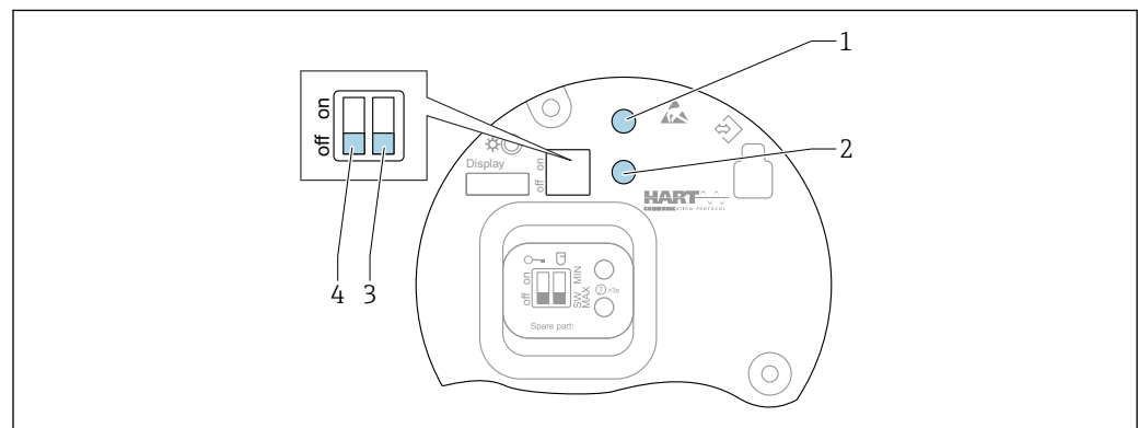
図 71 HART エレクトロニックインサート上の操作キーおよび DIP スイッチ
