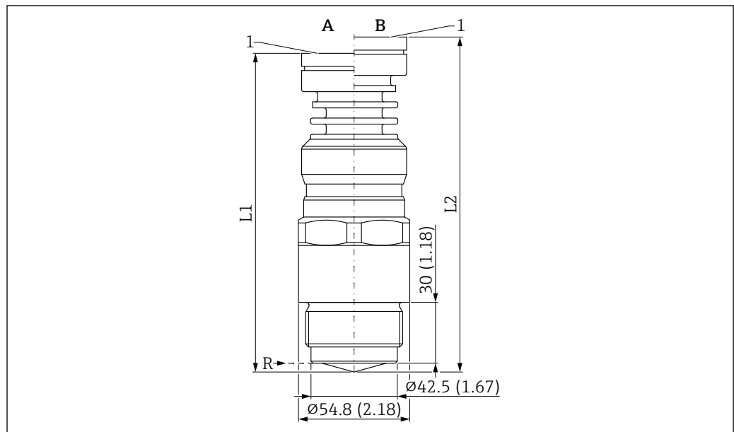
図 66 寸法；内蔵アンテナ、PEEK、40 mm (1.5 in)；プロセス接続、ネジ 1-1/2"。測定単位 mm (in)
