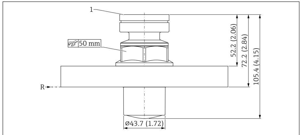
図 56 被覆アンテナ (PVDF、40 mm (1.5 in)、プロセス接続 UNI フランジ) の寸法。測定単位 mm (in)
