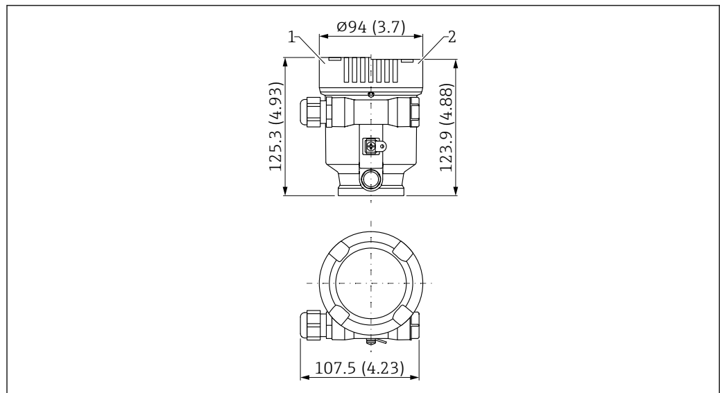
図 49 寸法 ; シングルコンパートメントハウジング (プラスチック) ; M20 カップリングおよびプラグ (プラスチック) 付き。測定単位 mm (in)
