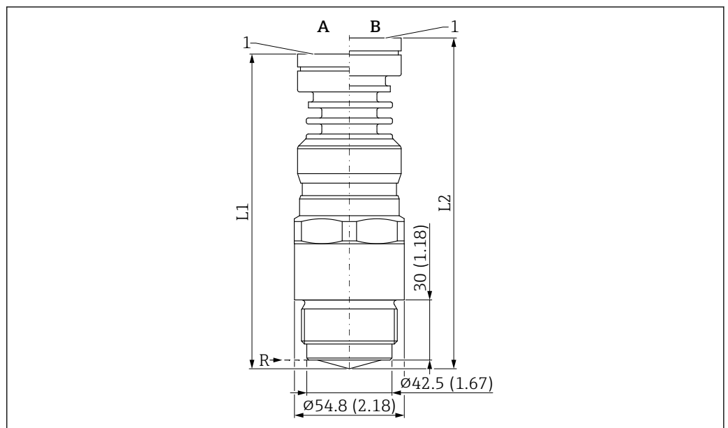
图 66 PEEK 一体式天线 (40 mm (1.5 in) 口径) 的外形尺寸示意图; 1-1/2" 螺纹过程连接。测量单位 mm (in)
