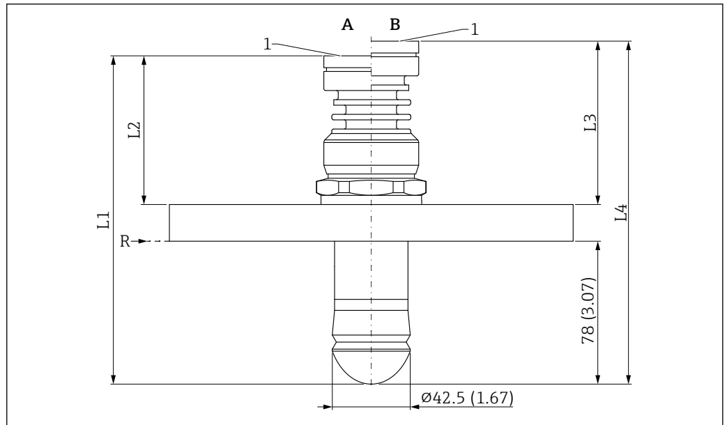
图 61 水滴型天线 (50 mm (2 in)口径) 的外形尺寸示意图; UNI 法兰过程连接。测量单位 mm (in)
