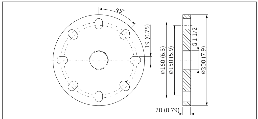
图 62 UNI 3"/DN80/80A 法兰的外形尺寸示意图。测量单位 mm (in)
