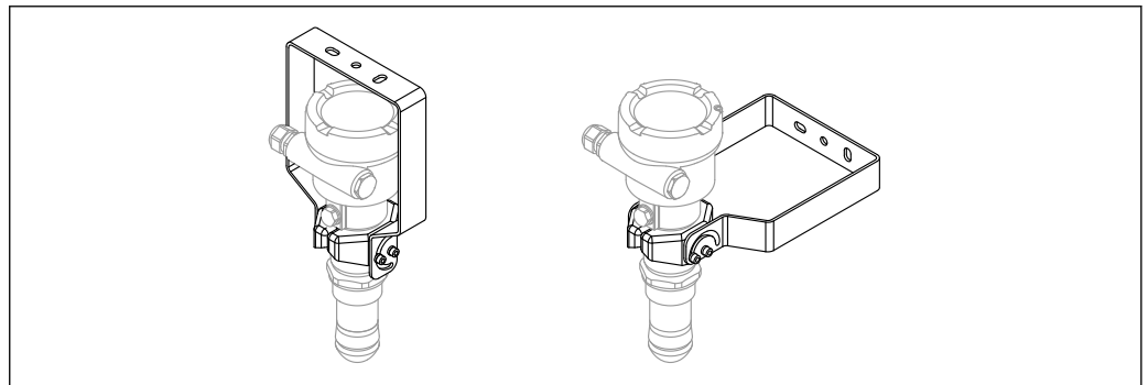
图 75 FMR6xB 的安装架（可调节）；安装在罐顶或墙壁上
