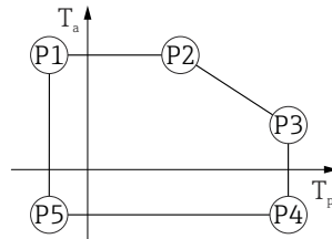
图 19 塑料外壳；过程温度范围：-20 ... +150 °C (-4 ... +302 °F)
