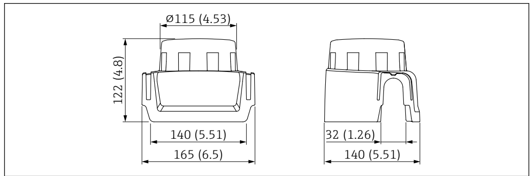
图 74 塑料防护罩 XW111 的外形尺寸示意图。测量单位 mm (in)
