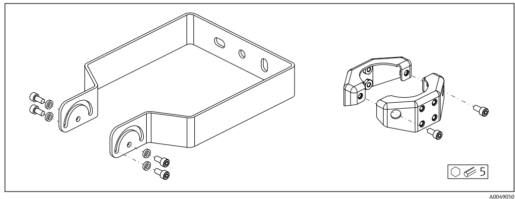
图 77 供货清单; FMR6xB 的安装架 (可调节)
