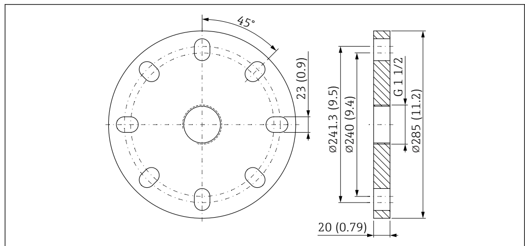
图 64 UNI 6"/DN150/150A 法兰的外形尺寸示意图。测量单位 mm (in)
