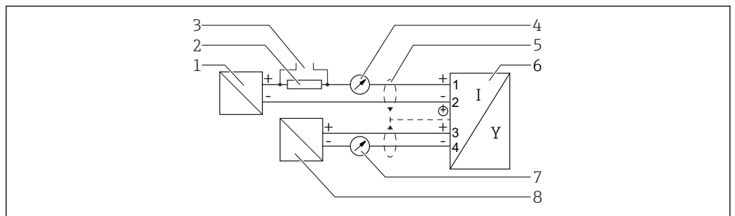
图 16 功能框图: 4 ... 20 mA HART + 4 ... 20 mA 模拟量
