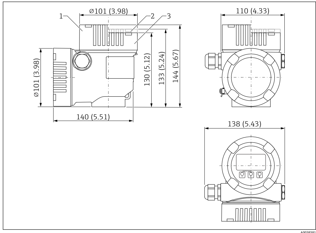
图 53 L 型双腔室铝外壳（带涂层）的外形尺寸示意图；包括 M20 接头和塑料插头。测量单位 mm (in)
