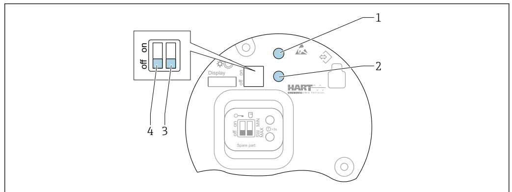
图 71 HART 电子插件上的操作按键和 DIP 开关
