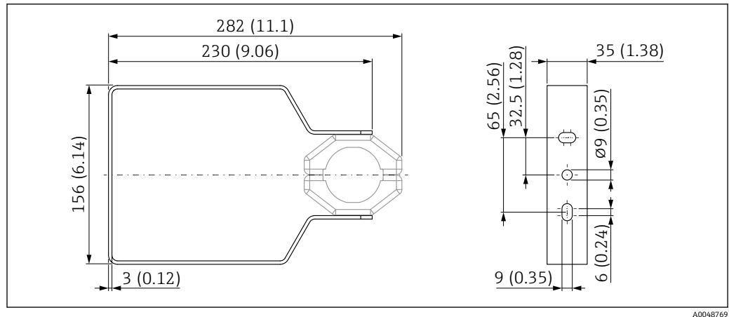
图 76 外形尺寸示意图; FMR6xB 的安装架 (可调节)。测量单位 mm (in)
