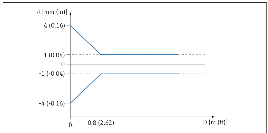
图 17 近距离测量时的最大测量误差
