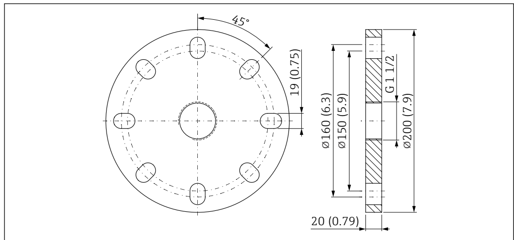
图 57 UNI 3"/DN80/80A 法兰的外形尺寸示意图。测量单位 mm (in)
