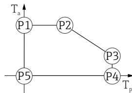
☑ 24 塑料外壳; 过程温度范围: 0 ... +80 °C (+32 ... +176 °F), 适用 CSA C/US 认证型仪表
