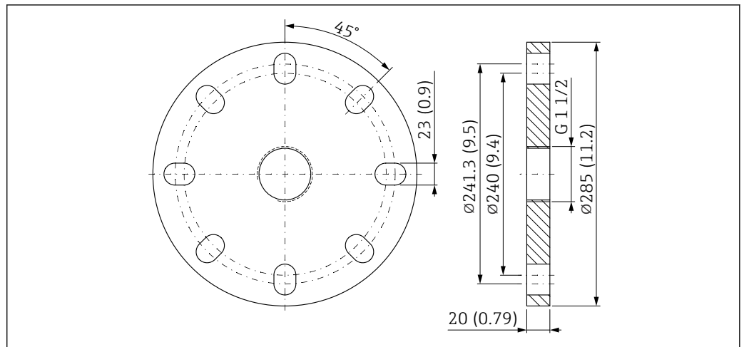
图 59 UNI 6"/DN150/150A 法兰的外形尺寸示意图。测量单位 mm (in)
