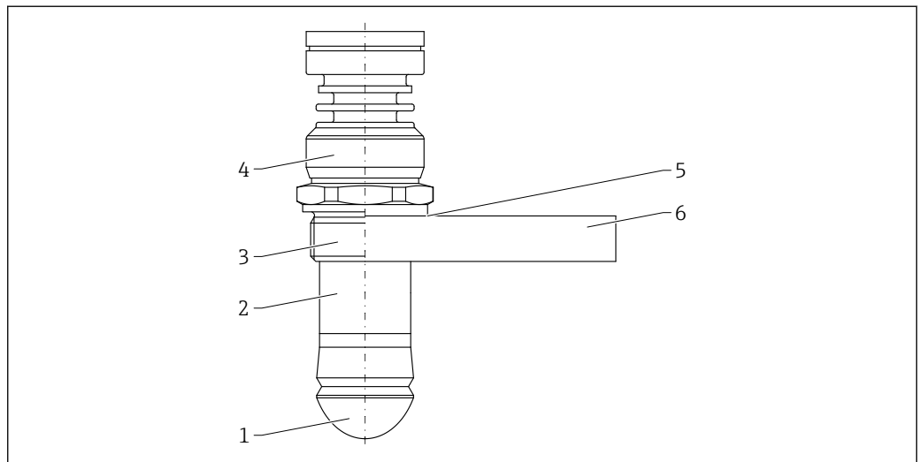
▣ 68 水滴型天线 (50 mm (2 in)口径) 的材质
