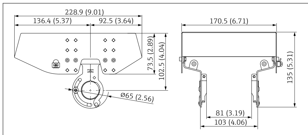
图 73 316L 防护罩 XW112 的外形尺寸示意图。测量单位 mm (in)
