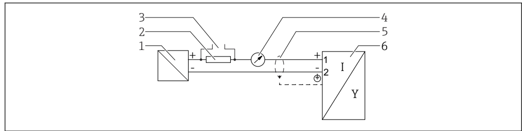
图 12 功能框图: 4 ... 20 mA HART
