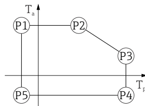
☑ 25 塑料外壳; 过程温度范围: -40 ... +130 °C (-40 ... +266 °F)
