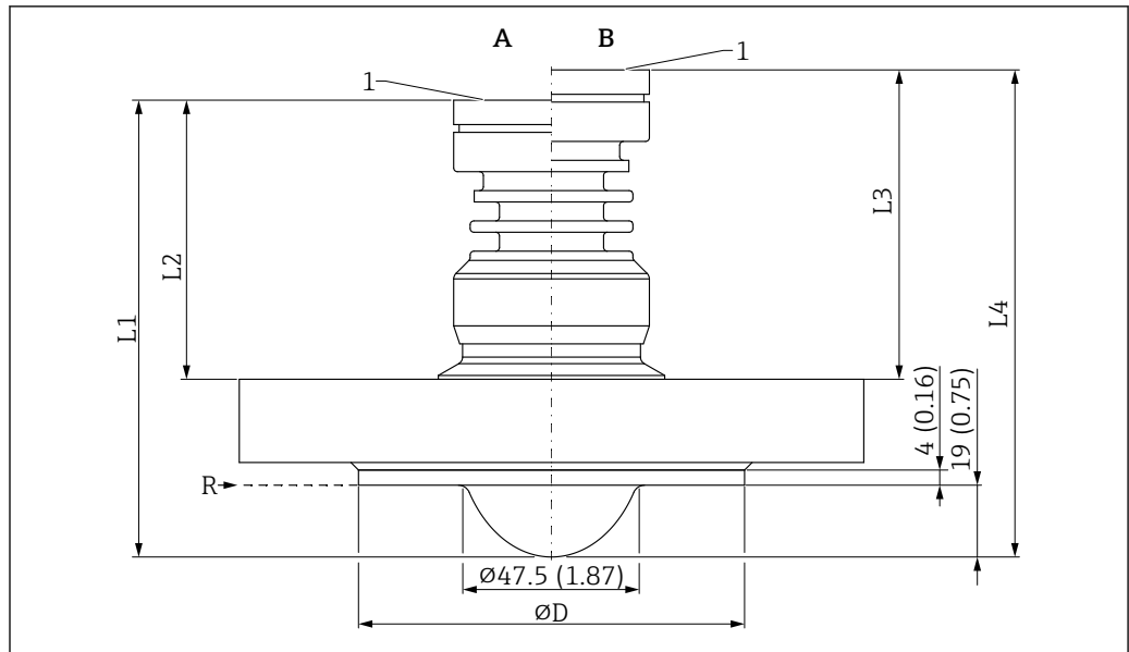
图 69 PTFE 涂层天线（齐平安装，50 mm (2 in)口径）的外形尺寸示意图；带法兰。测量单位 mm (in)
