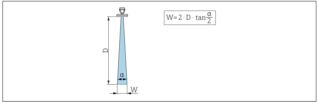
18 波束角 \alpha 、距离 D 和波束宽度 W 的相互关系
