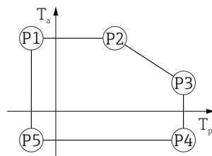
55 316L 外壳, 卫生型; 过程温度范围: -20 ... +150 °C (-4 ... +302 °F)
