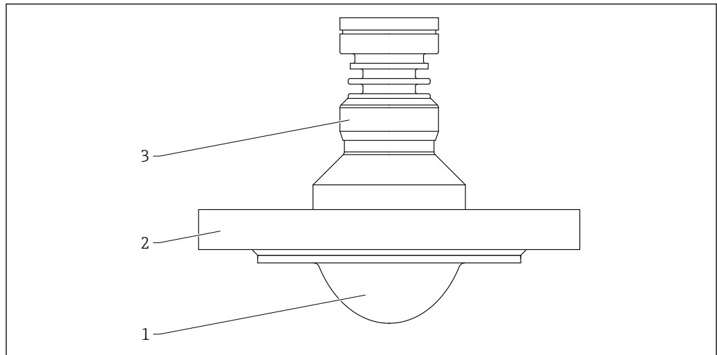
图 74 PTFE 涂层天线（齐平安装，80 mm (3 in)口径）的材质；带法兰
