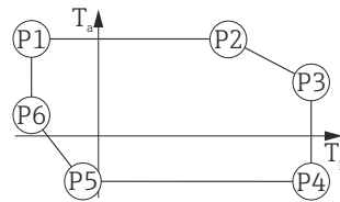
▣ 60 316L 外壳, 卫生型; 过程温度: -196 ... +200 °C (-320 ... +392 °F)
