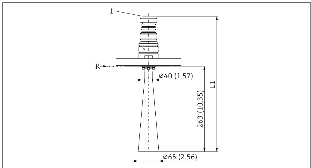
图 67 DN65 喇叭天线的外形尺寸示意图；法兰过程连接。测量单位 mm (in)
