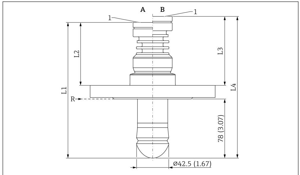
图 68 法兰过程连接的外形尺寸示意图。测量单位 mm (in)
