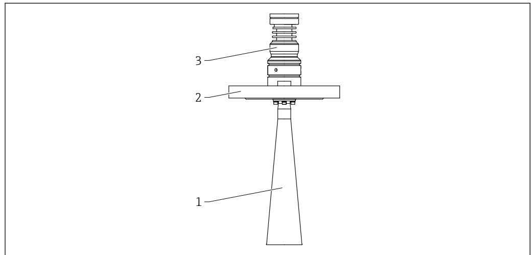
☞ 71 DN65 喇叭天线的材质。测量单位 mm (in)
