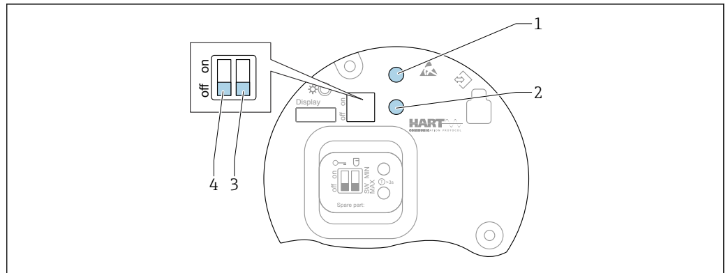
图 75 HART 电子插件上的操作按键和 DIP 开关
