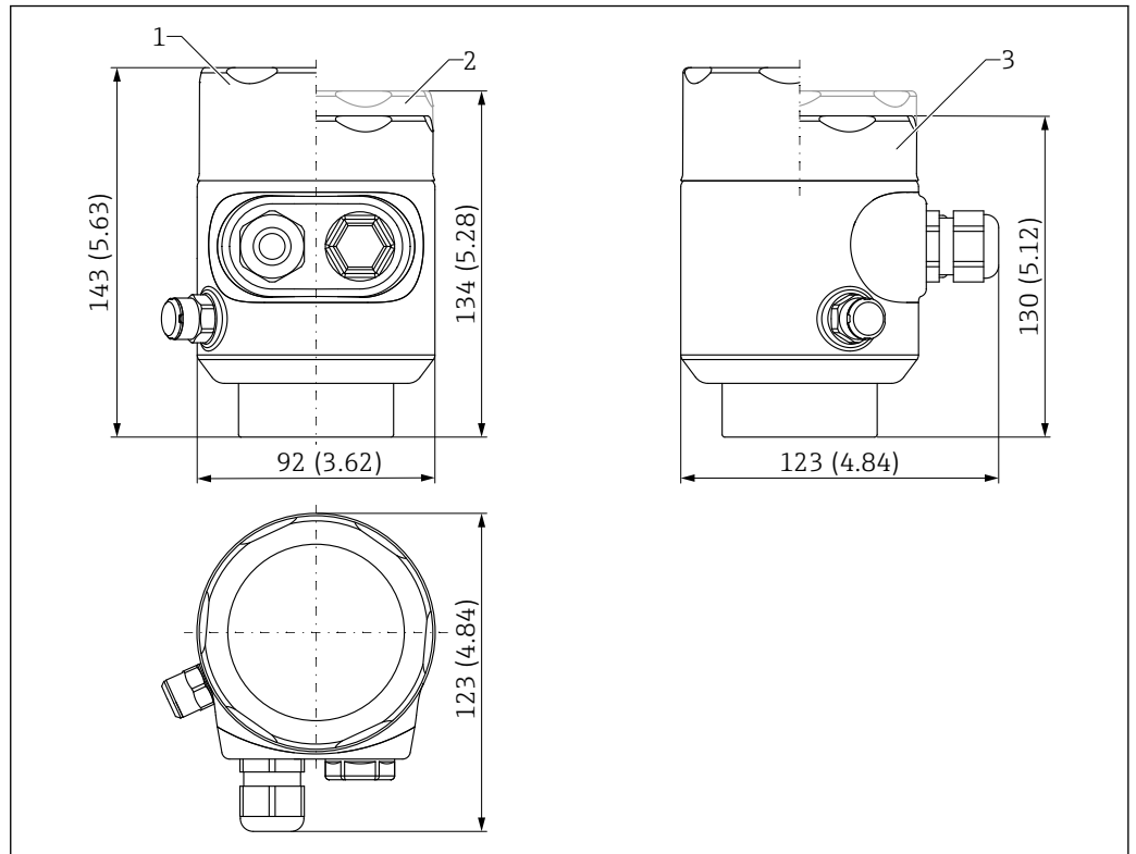
图 63 316L 单腔室外壳（卫生型）的外形尺寸示意图；包括 M20 接头和塑料插头。测量单位 mm (in)
