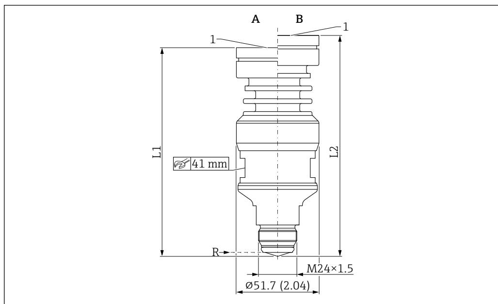
55 内蔵アンテナ、PEEK、20 mm (0.75 in)、M24 プロセス接続ネジ付きの寸法。測定単位 mm (in)
