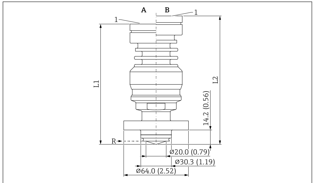
図 62 PEEK 外装付フラッシュマウントアンテナ、20 mm (0.75 in)、NEUMO バイオコントロール D25 の寸法。測定単位 mm (in)
