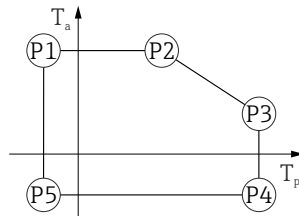
図 33 アルミニウムハウジング ; コーティング ; プロセス温度 -20\sim+150\text{ }^{\circ}\text{C} ( -4\sim+302\text{ }^{\circ}\text{F} )
