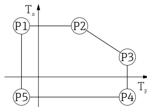
図 34 アルミニウムハウジング ; コーティング ; プロセス温度 -20\sim+200\text{ }^{\circ}\text{C} ( -4\sim+392\text{ }^{\circ}\text{F} )
