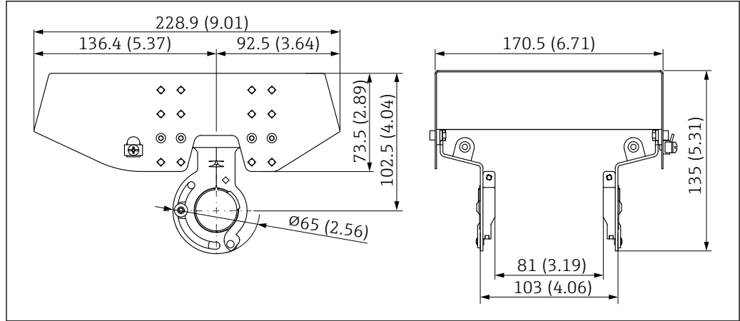
図 74 日除けカバー、SUS 316L 相当、XW112 の寸法。測定単位 mm (in)
