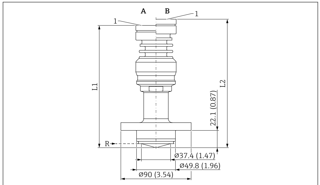
図 63 PEEK 外装付フラッシュマウントアンテナ、40 mm (1.5 in)、NEUMO バイオコントロール D50 の寸法。測定単位 mm (in)
