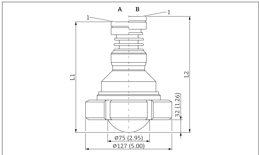
図 57 PTFE 外装付フラッシュマウントアンテナ (80 mm (3 in)、溝付ナット DIN11851) の寸法。測定単位 mm (in)
