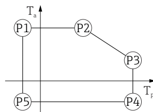
☐ 31 アルミニウムハウジング、コーティング ; プロセス温度 -10~+150 °C (+14~+302 °F)
