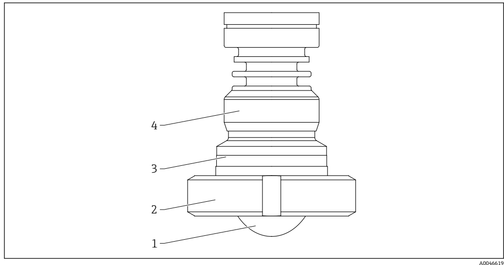
図 65 材質 ; PTFE 外装付フラッシュマウントアンテナ、50 mm (2 in)、溝付ナット DIN11851
