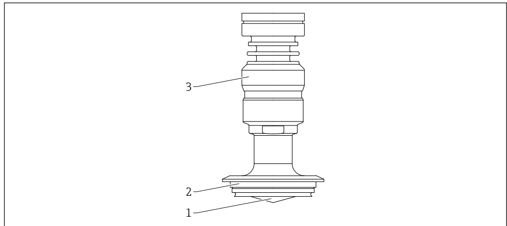
図 69 材質 ; PEEK 外装付フラッシュマウントアンテナ、40 mm (1.5 in)、バリベント N チューブ DN65-162
