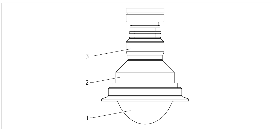
☐ 68 材質 ; PTFE 外装付フラッシュマウントアンテナ、80 mm (3 in)、トリクランプ ISO2852 付き
