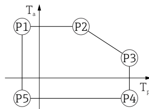
☐ 43 SUS 316L 相当製ハウジング、サニタリ仕様 ; プロセス温度 -10~+150 °C (+14~+302 °F)
