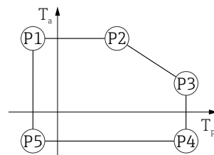
図 19 プラスチックハウジング ; プロセス温度 -10~+150 °C (+14~+302 °F)
