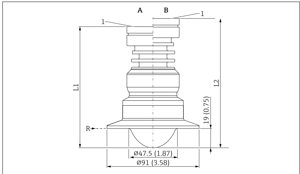
図 59 PTFE 外装付フラッシュマウントアンテナ (50 mm (2 in)、トリクランプ DN70-76.1 (3") ISO2852 付き) の寸法。測定単位 mm (in)
