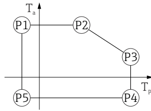
図 23 プラスチックハウジング ; プロセス温度 -20\sim+150\text{ }^{\circ}\text{C} ( -4\sim+302\text{ }^{\circ}\text{F} )
