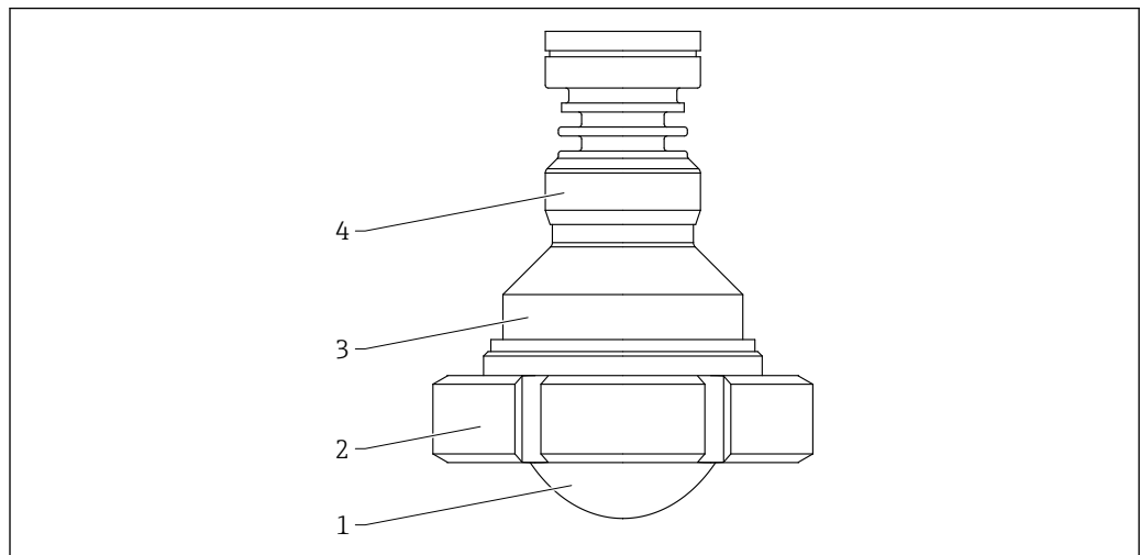
図 66 材質 ; 外装付フラッシュマウントアンテナ、80 mm (3 in)、ナット DIN11851。測定単位 mm (in)
