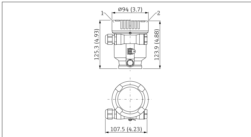
49 寸法；シングルコンパートメントハウジング（プラスチック）；M20 カップリングおよびプラグ（プラスチック）付き。測定単位 mm (in)
