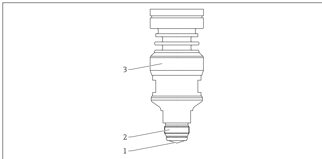
図 64 材質；内蔵アンテナ、PEEK、20 mm (0.75 in)、M24 プロセス接続ネジ付き
