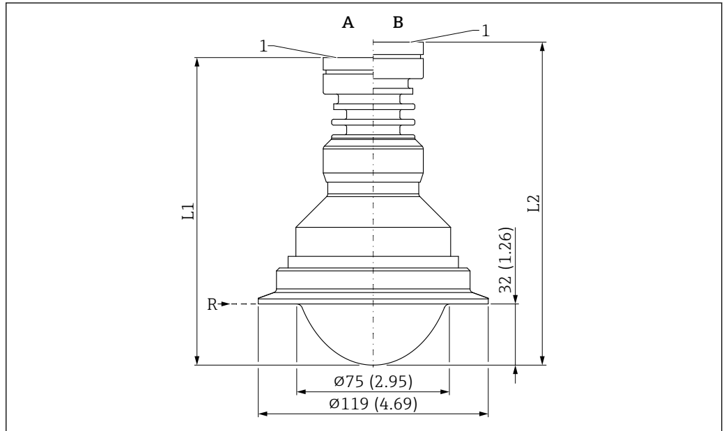
60 PTFE 外装付フラッシュマウントアンテナ (80 mm (3 in)、トリクランプ DN101.6 (4") ISO2852 付き) の寸法。測定単位 mm (in)
