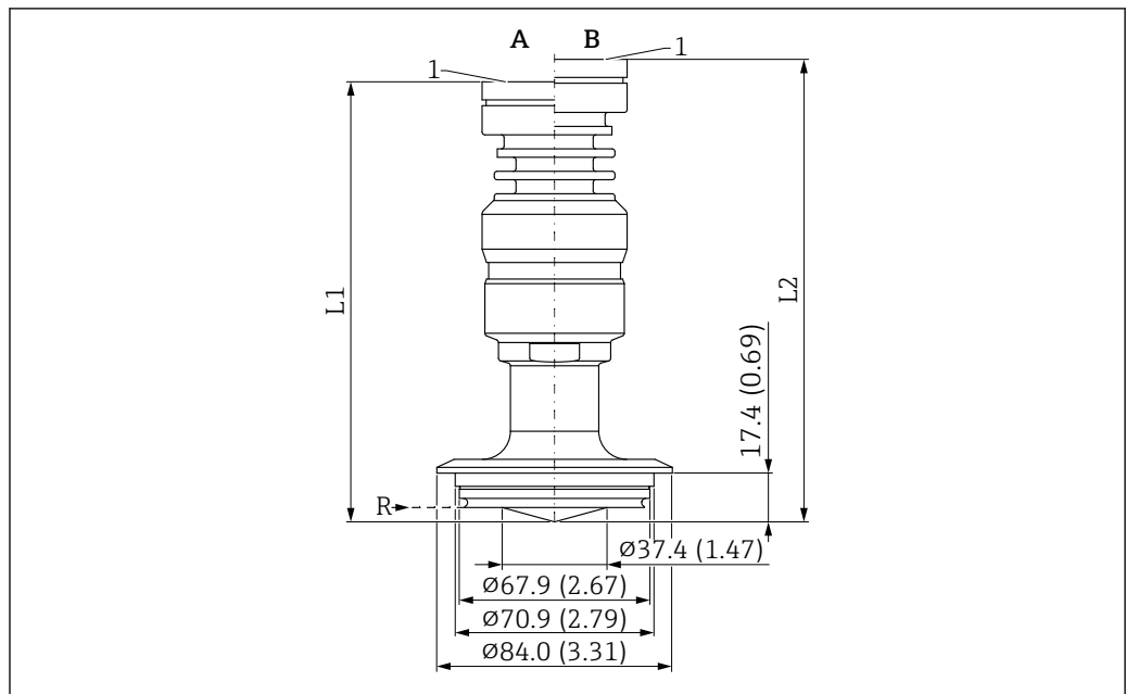
図 61 PEEK 外装付フラッシュマウントアンテナ、40 mm (1.5 in)、バリベント N チューブ DN65-162 の寸法。測定単位 mm (in)
