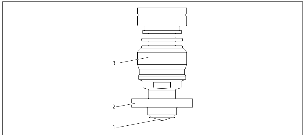
図 70 材質 ; PEEK 外装付フラッシュマウントアンテナ、20 mm (0.75 in)、NEUMO バイオコントロール D25
