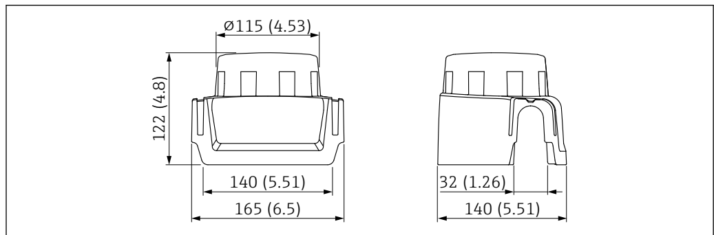
図 75 日除けカバー、プラスチック、XW111 の寸法。測定単位 mm (in)
