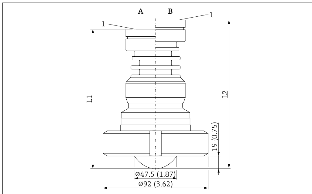
56 PTFE 外装付フラッシュマウントアンテナ (50 mm (2 in)、溝付ナット DIN11851) の寸法。測定単位 mm (in)
