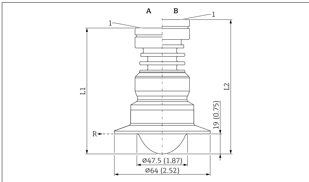
58 PTFE 外装付フラッシュマウントアンテナ (50 mm (2 in)、トリクランプ DN51 (2") ISO2852 付き) の寸法。測定単位 mm (in)
