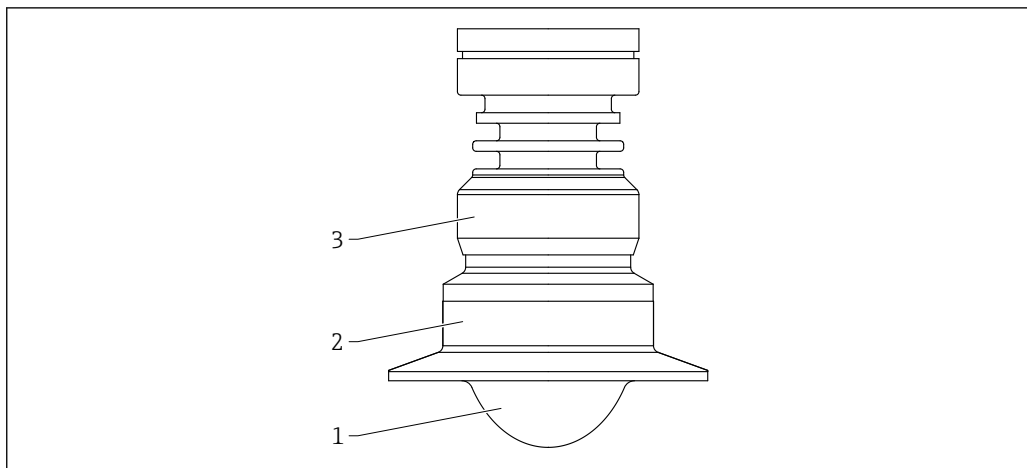
☐ 67 材質 ; PTFE 外装付フラッシュマウントアンテナ、50 mm (2 in)、トリクランプ ISO2852 付き。測定単位 mm (in)
