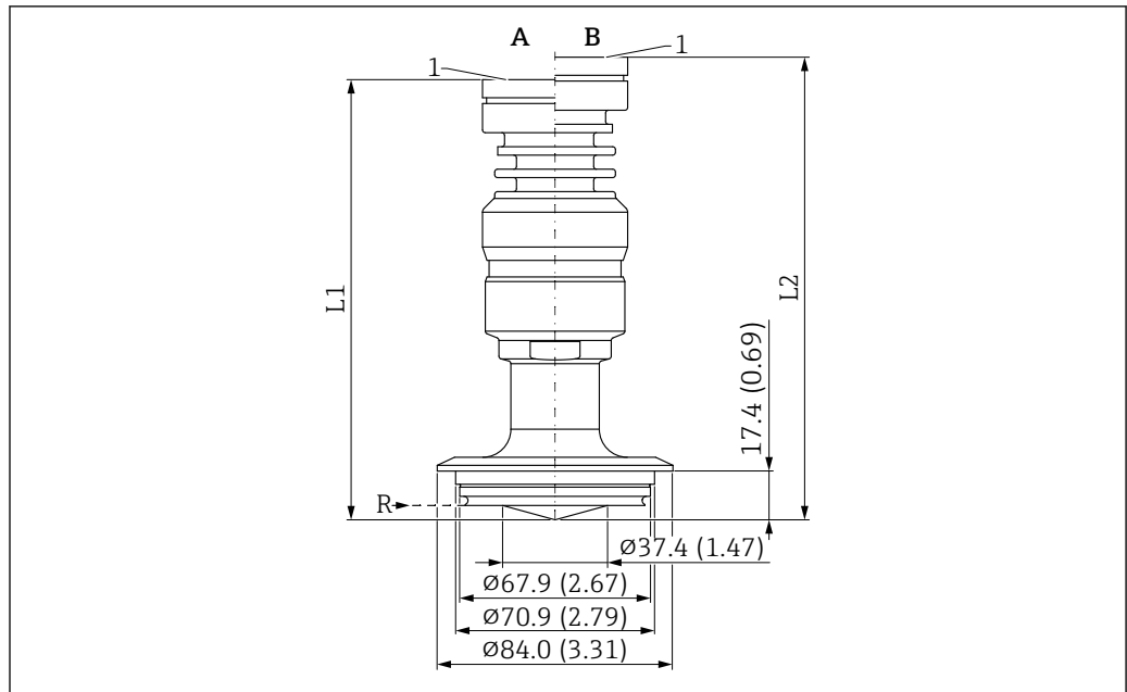
图 61 PEEK 涂层天线的外形尺寸示意图；齐平安装，40 mm (1.5 in) 口径，带 Varivent N DN65-162 接头。 测量单位 mm (in)
