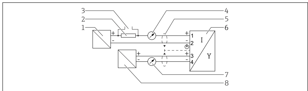
图 16 功能框图: 4 ... 20 mA HART + 4 ... 20 mA 模拟量
