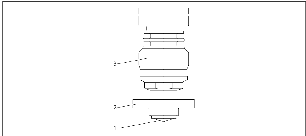
图 70 PEEK 涂层天线的材质；齐平安装，20 mm (0.75 in)口径，带 NEUMO BioControl D25 卫生型连接
