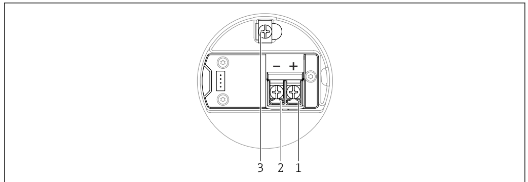
▣ 8 接线腔中的接线端子分配; 4 ... 20 mA HART; 双腔室外壳 (L 型)
