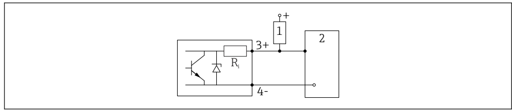
图 15 数字量输入的连接示例
