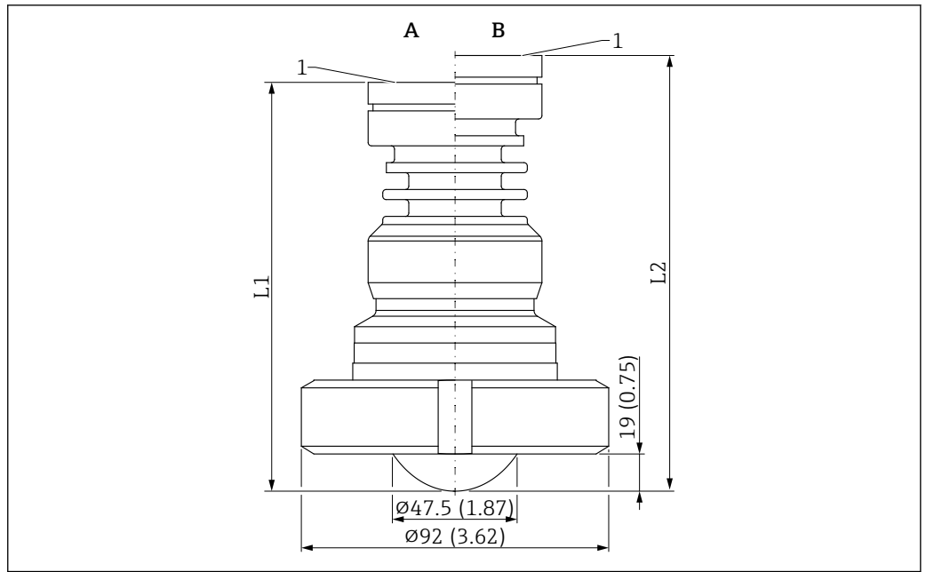
图 56 PTFE 涂层天线（齐平安装，50 mm (2 in)口径）的外形尺寸示意图；带 DIN11851 开槽螺母。测量单位 mm (in)
