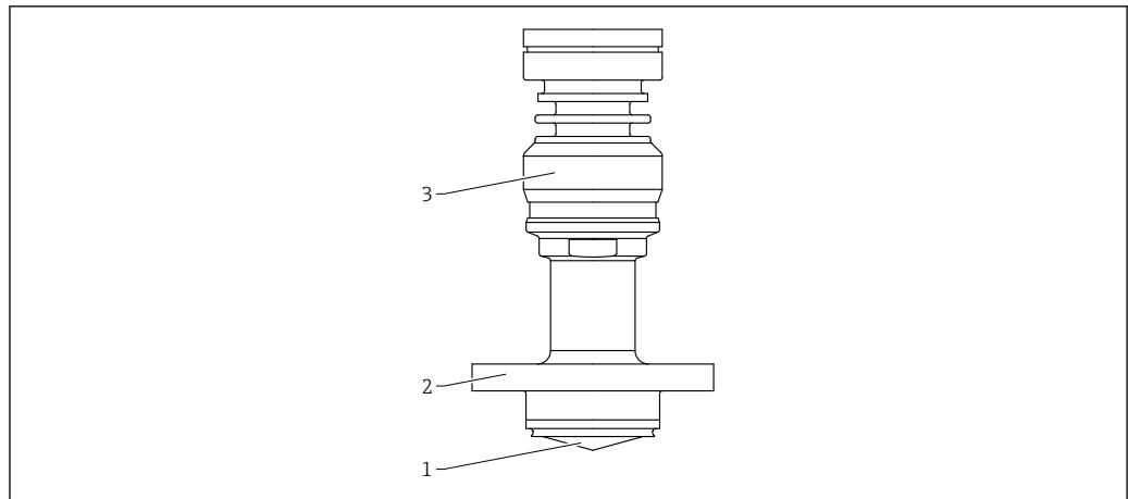
图 71 PEEK 涂层天线的材质；齐平安装，40 mm (1.5 in)口径，带 NEUMO BioControl D50 卫生型连接
