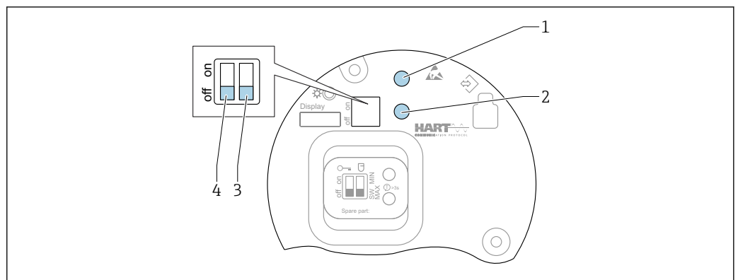
图 72 HART 电子插件上的操作按键和 DIP 开关
