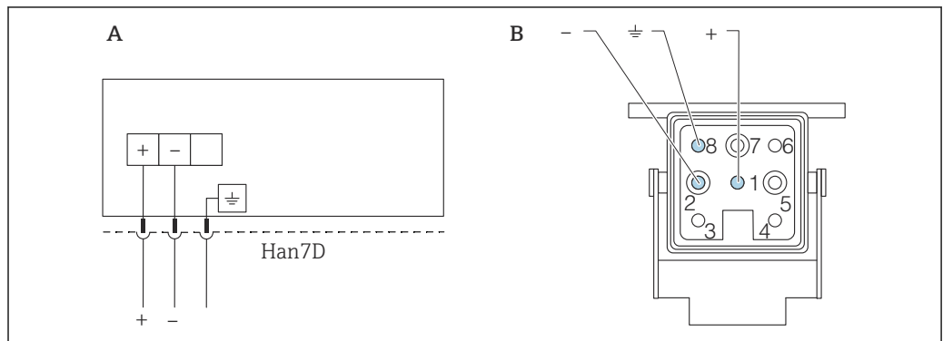
A 带 Harting Han7D 插头的仪表的电气连接示意图
