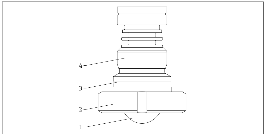
▣ 65 PTFE 涂层天线的材质; 齐平安装, 50 mm (2 in)口径, 带 DIN11851 开槽螺母
