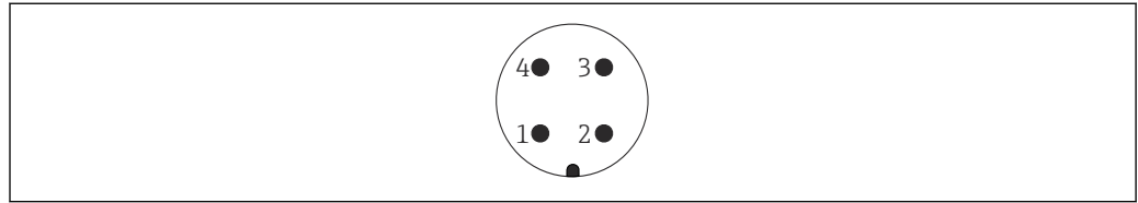
图 11 仪表连接插头示意图
