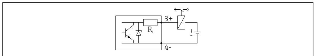
图 14 继电器的连接示例
