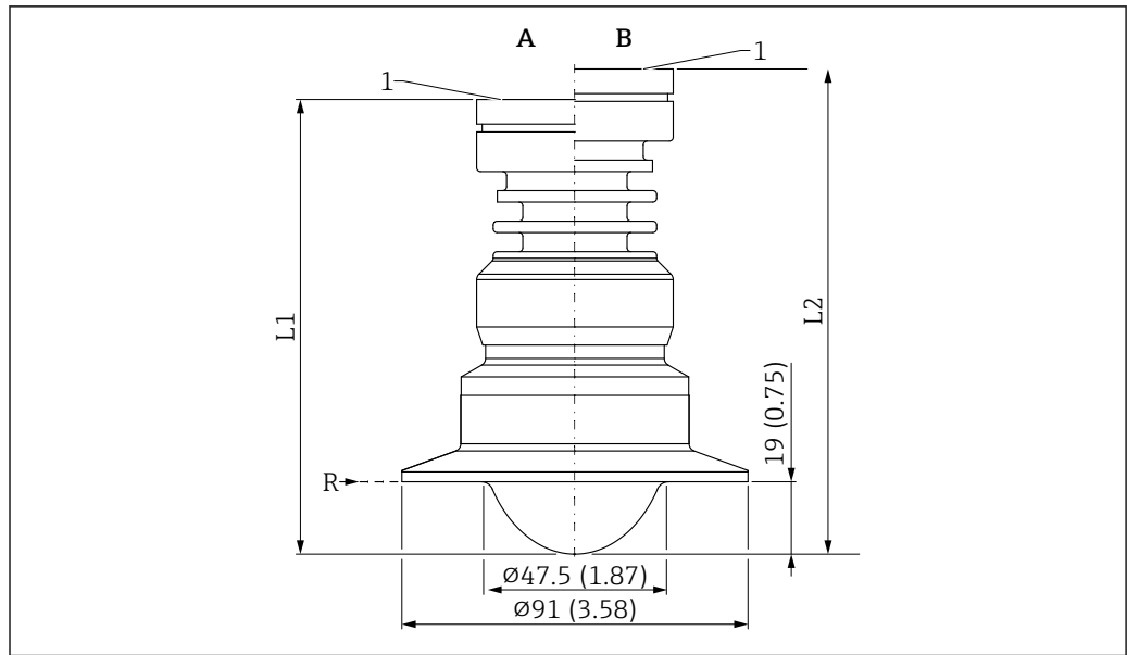
59 PTFE 涂层天线（齐平安装，50 mm (2 in)口径）的外形尺寸示意图；带 ISO2852 Tri-Clamp DN70-76.1 (3")卡箍。测量单位 mm (in)
