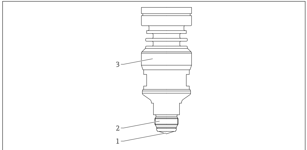
▣ 64 PEEK 一体式天线的材质; 20 mm (0.75 in)口径, 带 M24 螺纹过程连接
