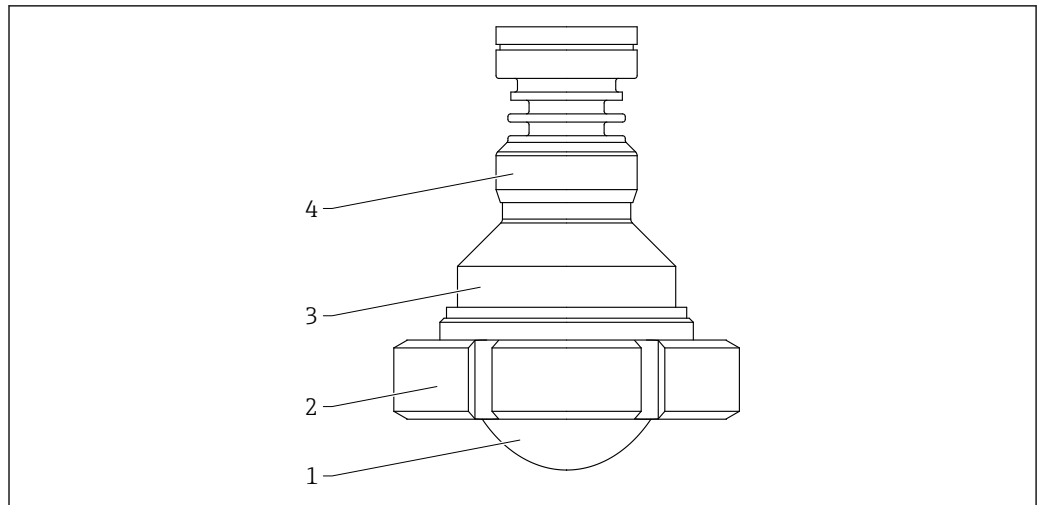
▣ 66 涂层天线的材质；齐平安装，80 mm (3 in)口径，带 DIN11851 开槽螺母。测量单位 mm (in)
