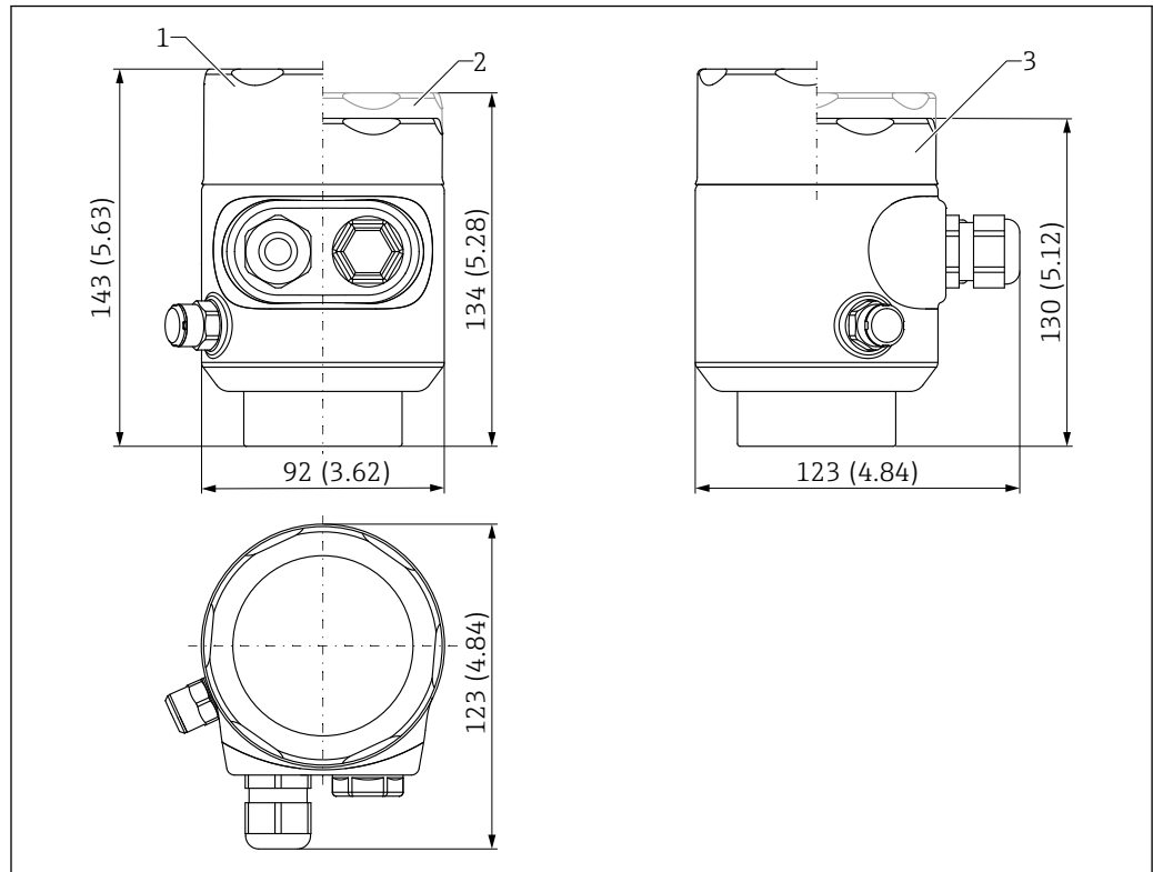
图 51 316L 单腔室外壳 (卫生型) 的外形尺寸示意图; 包括 M20 接头和塑料插头。测量单位 mm (in)
