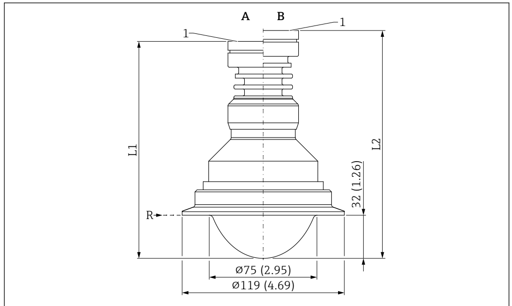
图 60 PTFE 涂层天线（齐平安装，80 mm (3 in)口径）的外形尺寸示意图；带 ISO2852 Tri-Clamp DN101.6 (4")卡箍。测量单位 mm (in)
