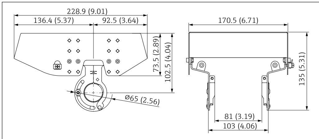
図 48 日除けカバー、SUS 316L 相当、XW112 の寸法。測定単位 mm (in)
