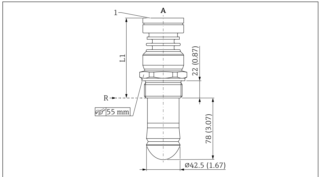
図 39 ドリッポフアンテナ 50 mm (2 in)、ネジ込みプロセス接続の寸法
