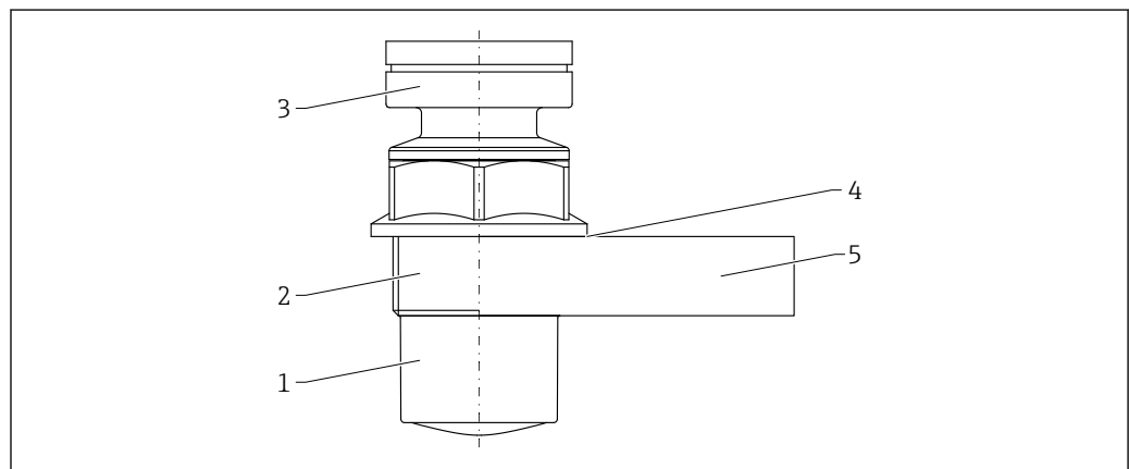
図 44 材質；被覆アンテナ PVDF、40 mm (1.5 in)
