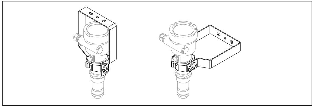
50 調整可能な取付ブラケット FMR6xB ; 天井または壁面取付け
