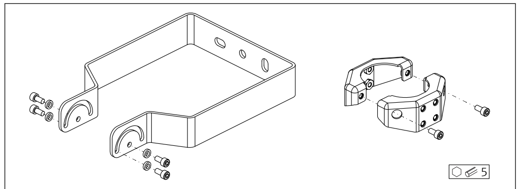
52 納入範囲；調整可能な取付ブラケット FMR6xB
