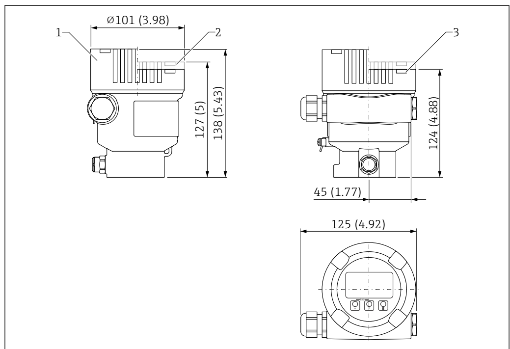
図 29 寸法 ; シングルコンパートメントハウジング (アルミニウム、コーティング) ; M20 カップリングおよびプラグ (プラスチック) 付き。測定単位 mm (in)
