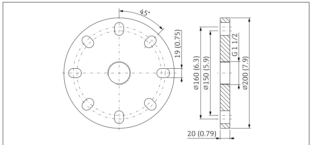
図 36 UNI フランジ 3"/DN80/80A の寸法。測定単位 mm (in)
