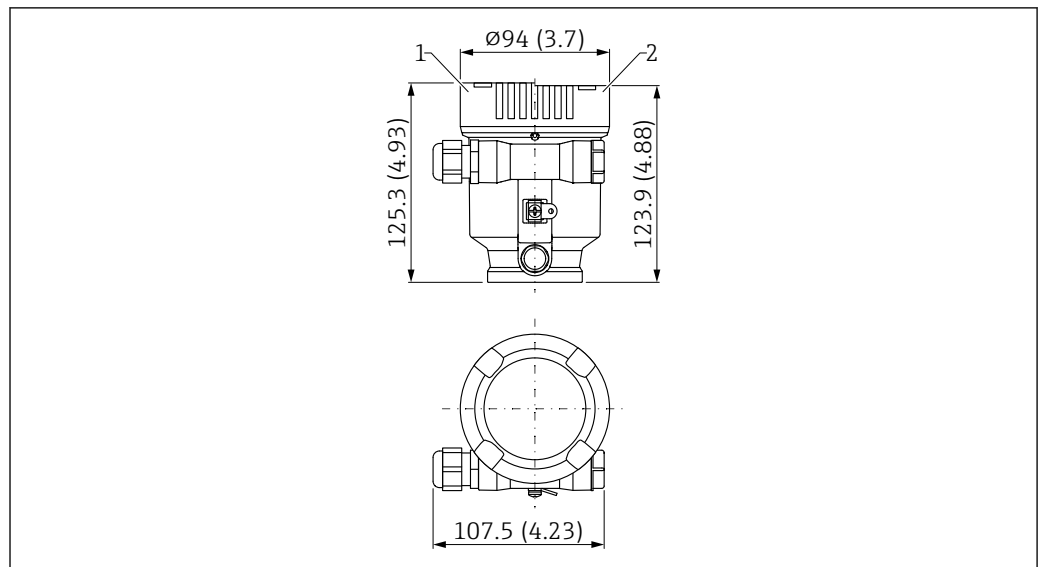
図 28 寸法 ; シングルコンパートメントハウジング (プラスチック) ; M20 カップリングおよびプラグ (プラスチック) 付き。測定単位 mm (in)
