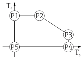
図 19 プラスチックハウジング ; プロセス温度 0\sim+80\text{ }^{\circ}\text{C} ( +32\sim+176\text{ }^{\circ}\text{F} )、CSA C/US 認定取得
