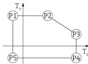
■ 26 SUS 316L 相当製ハウジング、サニタリ仕様 ; プロセス温度 -40\sim+80\text{ }^{\circ}\text{C} ( -40\sim+176\text{ }^{\circ}\text{F} )
