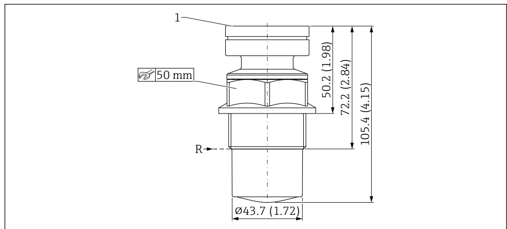
図 34 寸法；被覆アンテナ、PVDF、40 mm (1.5 in)。測定単位 mm (in)
