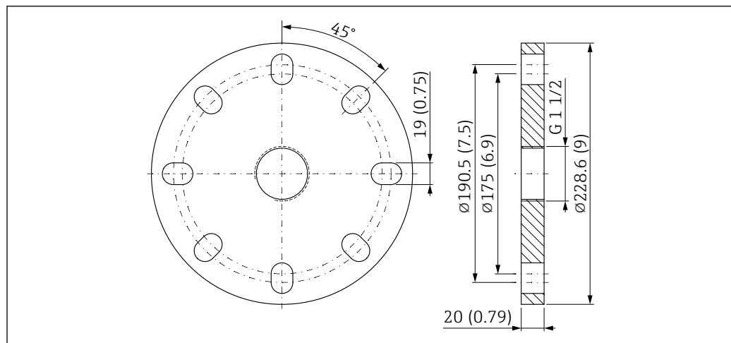
図 42 UNI フランジ 4"/DN100/100A の寸法。測定単位 mm (in)
