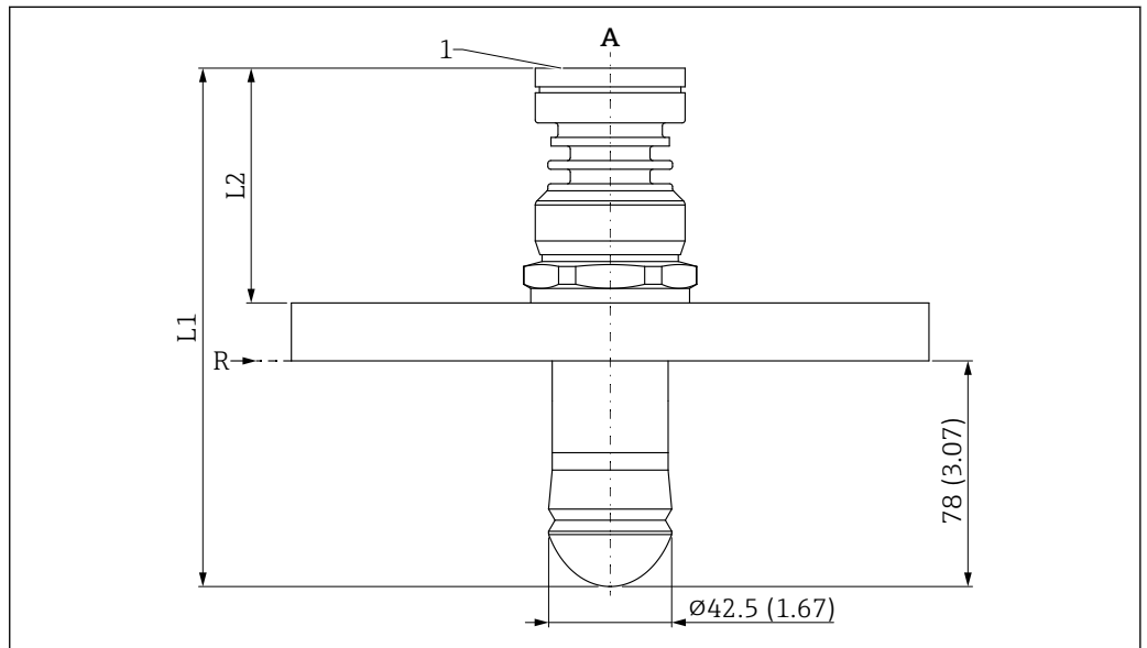
図 40 ドリッポフアンテナ 50 mm (2 in) (UNI フランジプロセス接続) の寸法。測定単位 mm (in)
