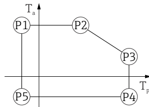
図 20 プラスチックハウジング ; プロセス温度 -40\sim+130\text{ }^{\circ}\text{C} ( -40\sim+266\text{ }^{\circ}\text{F} )
