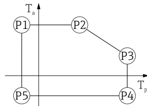
図 22 アルミニウムハウジング ; コーティング ; プロセス温度 -40~+80 °C (-40~+176 °F)
