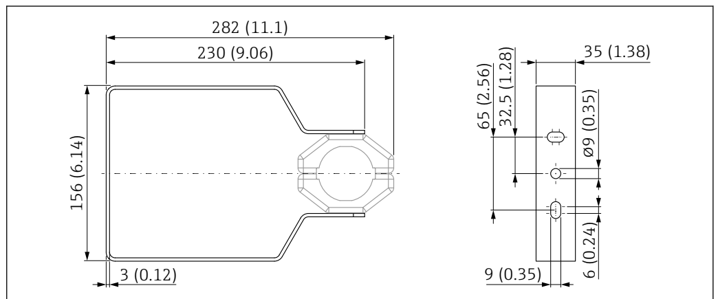
51 寸法；調整可能な取付ブラケット FMR6xB。測定単位 mm (in)
