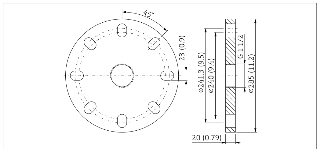
図 38 UNI フランジ 6"/DN150/150A の寸法。測定単位 mm (in)
