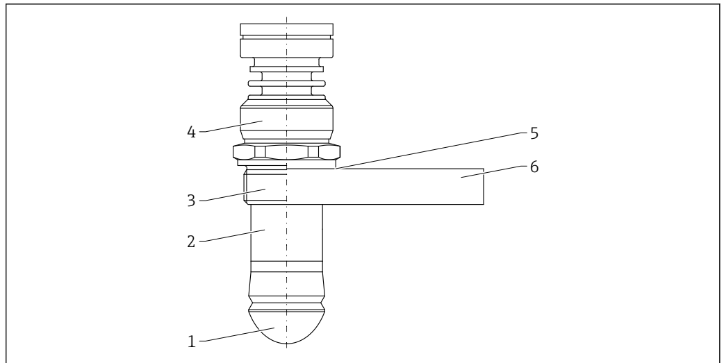
図 45 材質；ドリップオフアンテナ 50 mm (2 in)
