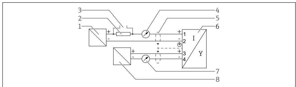
图 15 功能框图: 4 ... 20 mA HART + 4 ... 20 mA 模拟量
