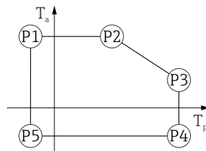
图 23 铝外壳, 带涂层; 过程温度范围: -40 ... +130 °C (-40 ... +266 °F)
