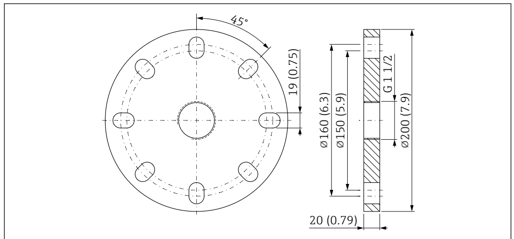
图 36 UNI 3"/DN80/80A 法兰的外形尺寸示意图。测量单位 mm (in)
