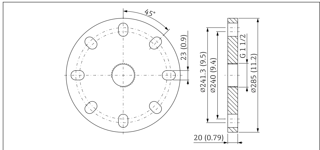
图 38 UNI 6"/DN150/150A 法兰的外形尺寸示意图。测量单位 mm (in)
