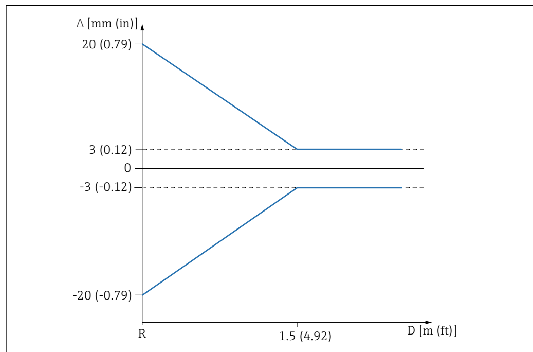
图 16 近距离测量时的最大测量误差
