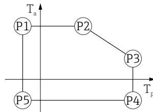
图 22 铝外壳, 带涂层; 过程温度范围: -40 ... +80 °C (-40 ... +176 °F)
