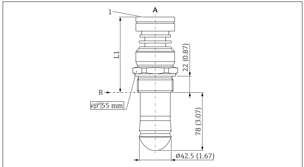
图 39 水滴型天线 (50 mm (2 in)口径) 的外形尺寸示意图，螺纹过程连接
