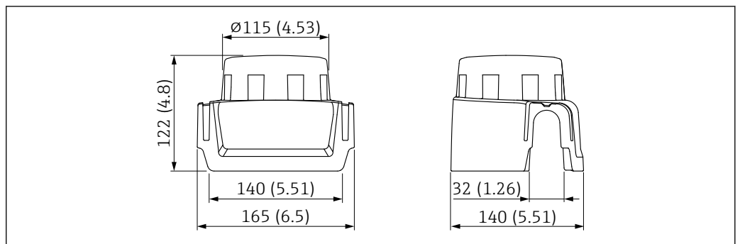
图 49 塑料防护罩 XW111 的外形尺寸示意图。测量单位 mm (in)
