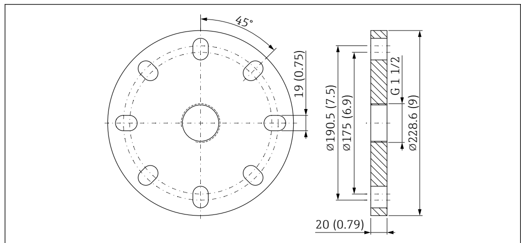
图 42 UNI 4"/DN100/100A 法兰的外形尺寸示意图。测量单位 mm (in)
