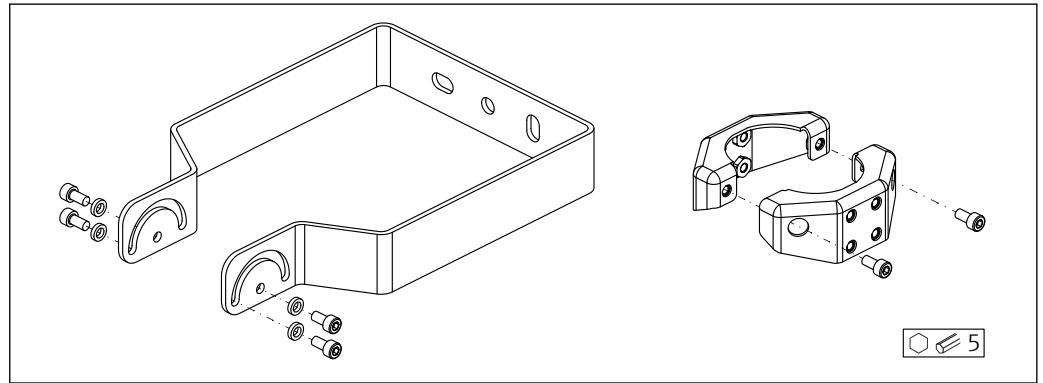
图 52 供货清单; FMR6xB 的安装架 (可调节)
