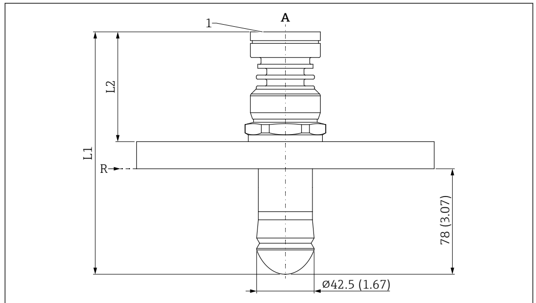
图 40 水滴型天线 (50 mm (2 in)口径) 的外形尺寸示意图；UNI 法兰过程连接。测量单位 mm (in)
