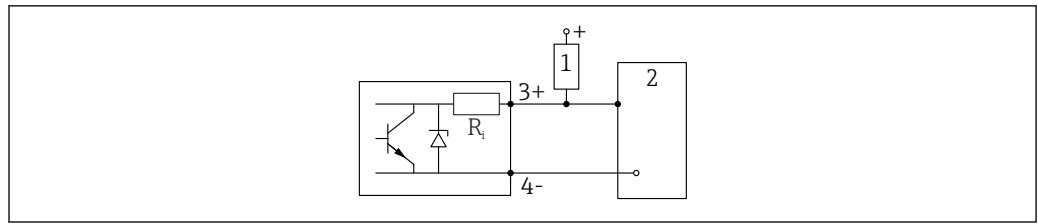
图 14 数字量输入的连接示例
