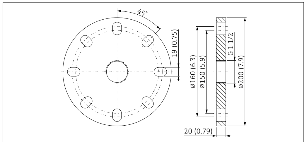
图 41 UNI 3"/DN80/80A 法兰的外形尺寸示意图。测量单位 mm (in)
