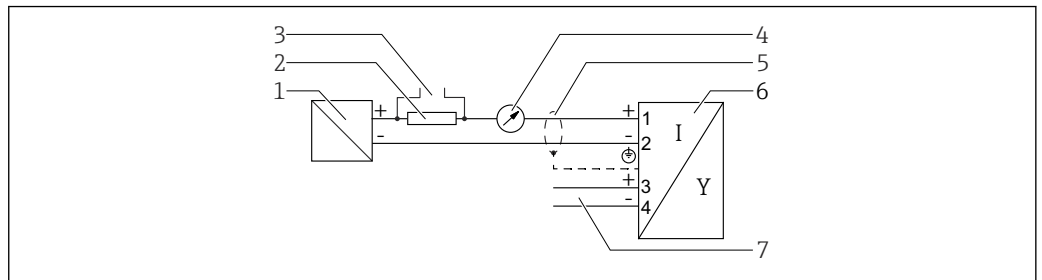
图 12 功能框图: 4 ... 20 mA HART, 开关量输出
