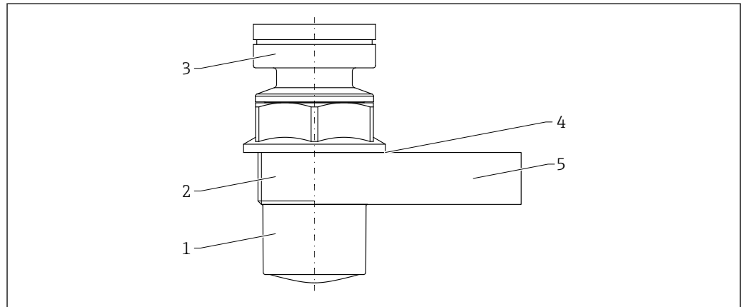
图 44 PVDF 全密封天线（40 mm (1.5 in) 口径）的材质
