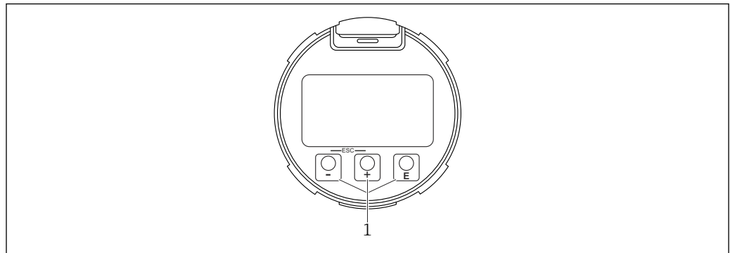
图 47 图形显示单元，带光敏按键（1）
