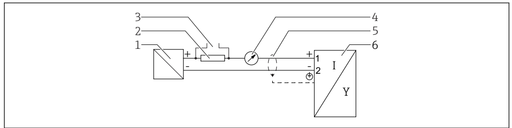
图 11 功能框图: 4 ... 20 mA HART
