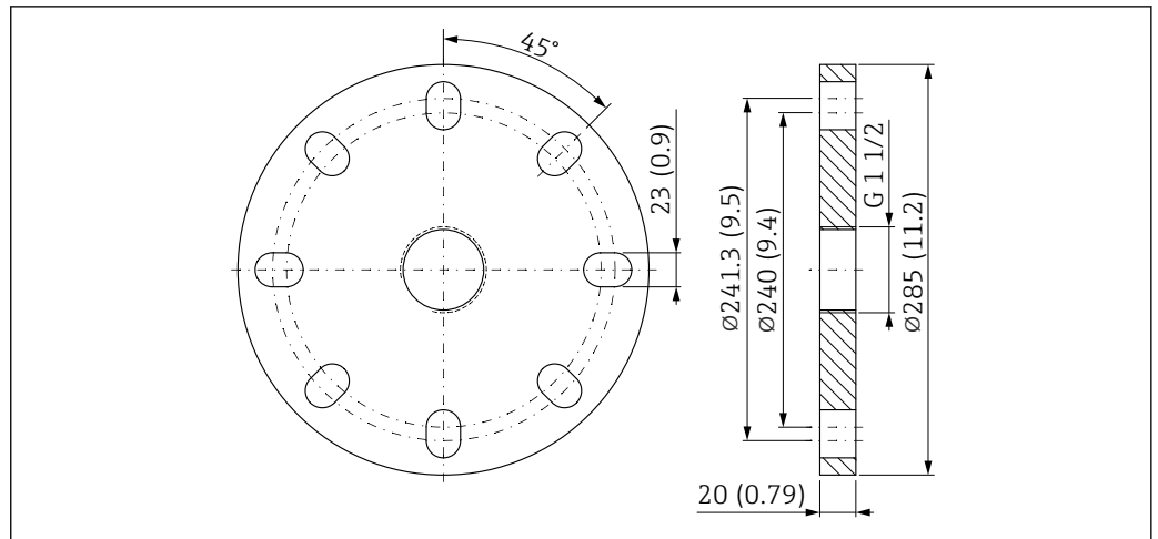
图 43 UNI 6"/DN150/150A 法兰的外形尺寸示意图。测量单位 mm (in)
