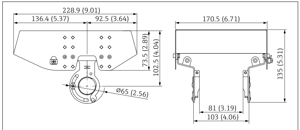
图 48 316L 防护罩 XW112 的外形尺寸示意图。测量单位 mm (in)
