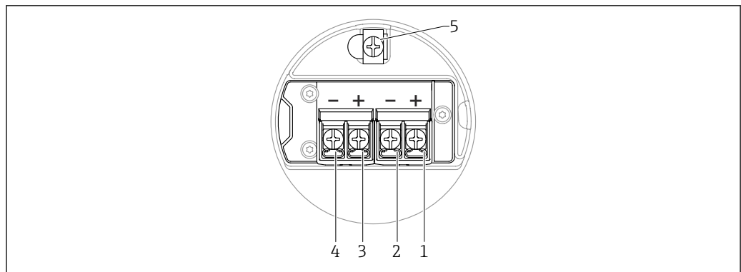
图 6 接线腔中的接线端子分配; 4 ... 20 mA HART, 开关量输出, 双腔室外壳
