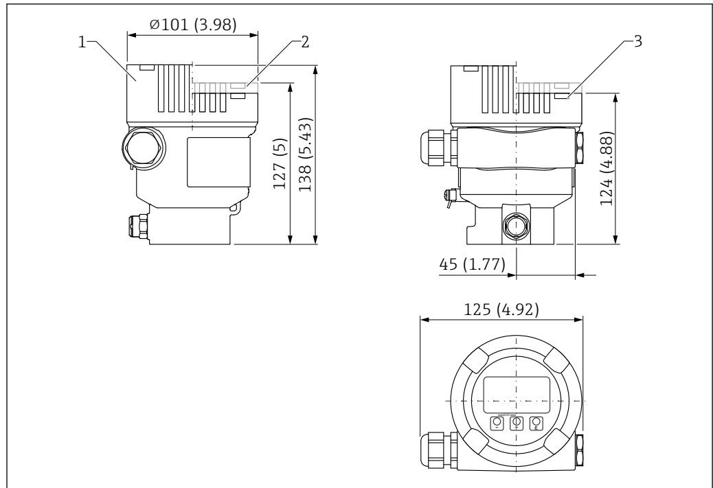
图 29 单腔室铝外壳 (带涂层) 的外形尺寸示意图; 包括 M20 接头和塑料插头。测量单位 mm (in)
