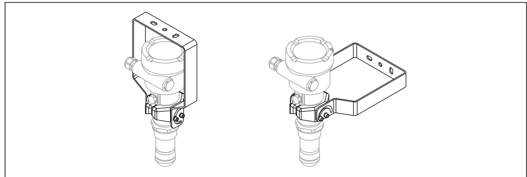
图 50 FMR6xB 的安装架（可调节）；安装在罐顶或墙壁上
