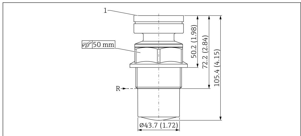
图 34 PVDF 全密封天线（40 mm (1.5 in) 口径）的外形尺寸示意图。测量单位 mm (in)
