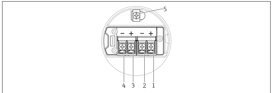
☐ 9 接线腔中的接线端子分配; 4 ... 20 mA HART, 开关量输出; 双腔室外壳 (L 型)
