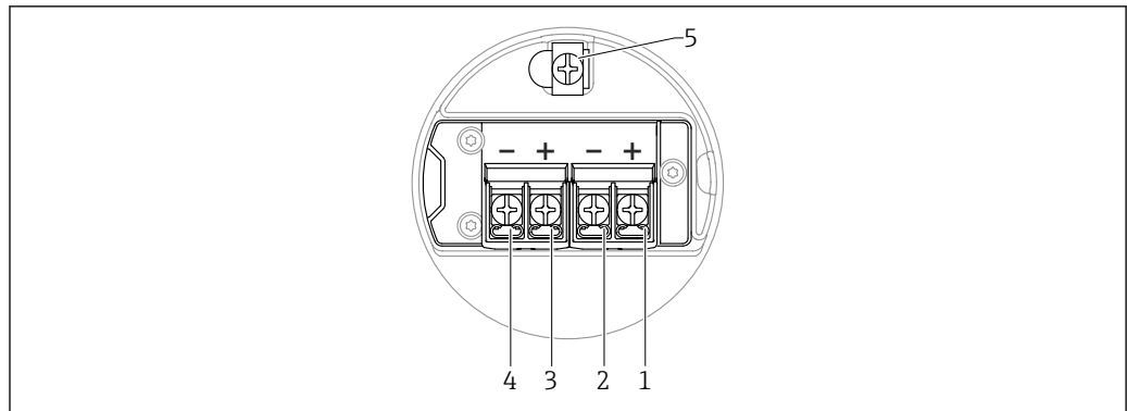
图 5 接线腔中的接线端子分配; 4 ... 20 mA HART + 4 ... 20 mA 模拟量; 双腔室外壳
