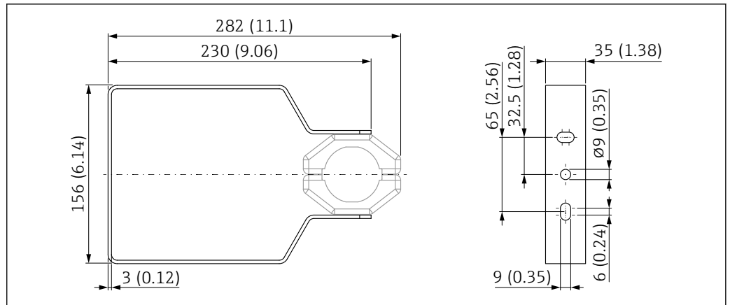
图 51 外形尺寸示意图; FMR6xB 的安装架 (可调节)。测量单位 mm (in)
