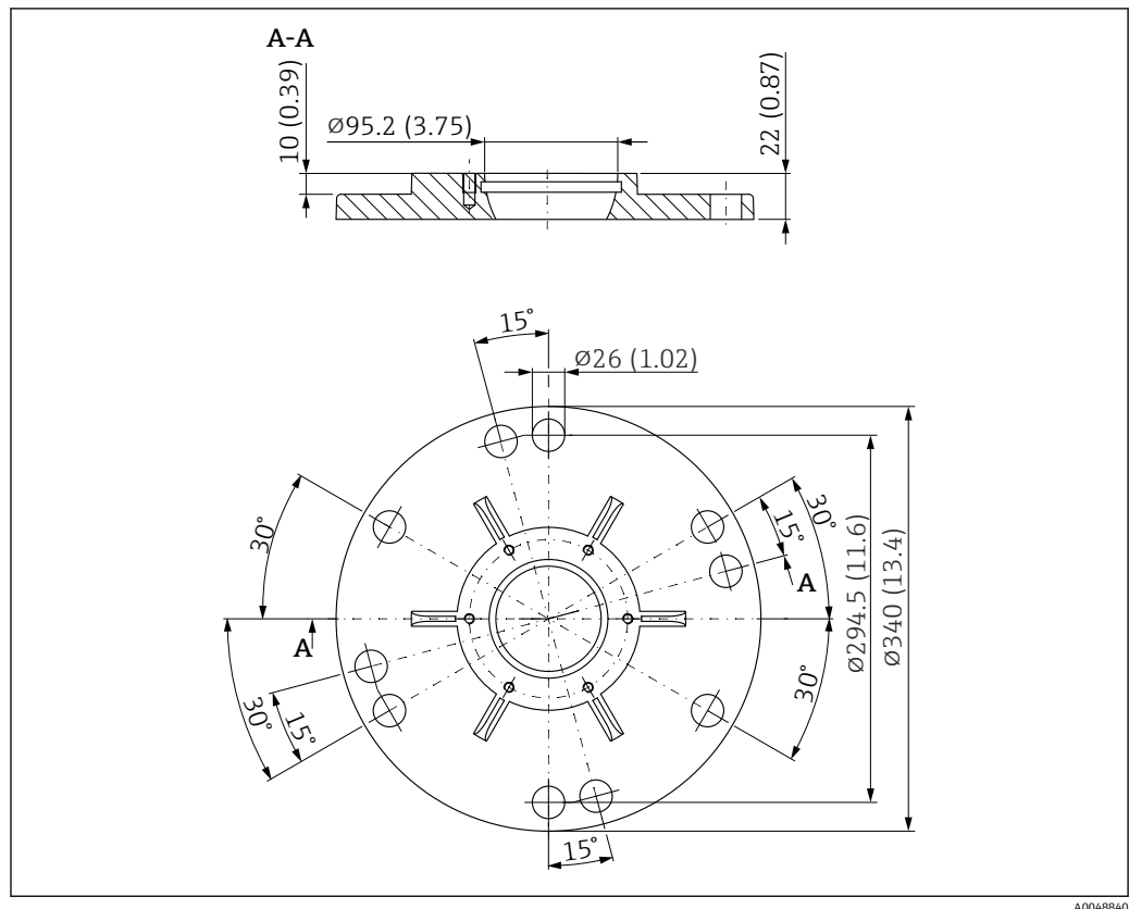
图 67 UNI 8"/DN200/200A 法兰的外形尺寸示意图；适用带天线角度调节装置的天线。测量单位 mm (in)
