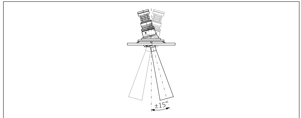
图 17 喇叭天线, 带天线角度调节装置
