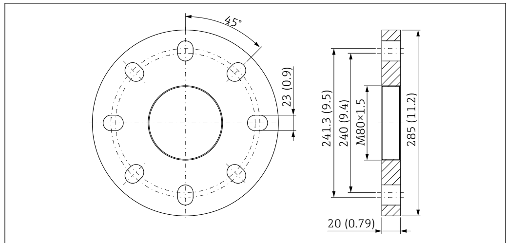
图 59 UNI 6"/DN150/150A 法兰，适用带空气吹扫接口的 PTFE 水滴型天线 (50 mm (2 in)口径)。测量单位 mm (in)
