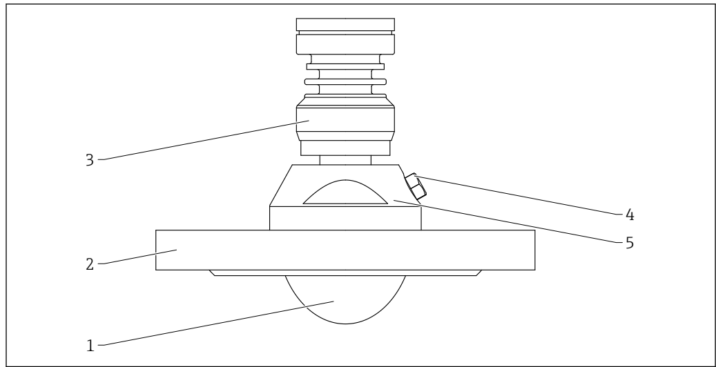
图 72 天线（齐平安装，80 mm (3 in)口径）的材质，带法兰和空气吹扫接口。测量单位 mm (in)
