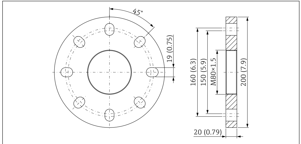
57 UNI 3"/DN80/80A 法兰，适用带空气吹扫接口的 PTFE 水滴型天线 (50 mm (2 in)口径)。测量单位 mm (in)
