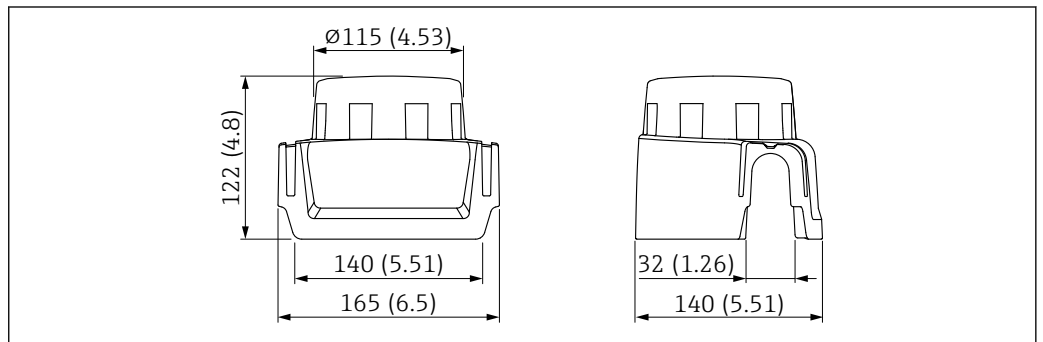
图 78 塑料防护罩 XW111 的外形尺寸示意图。测量单位 mm (in)
