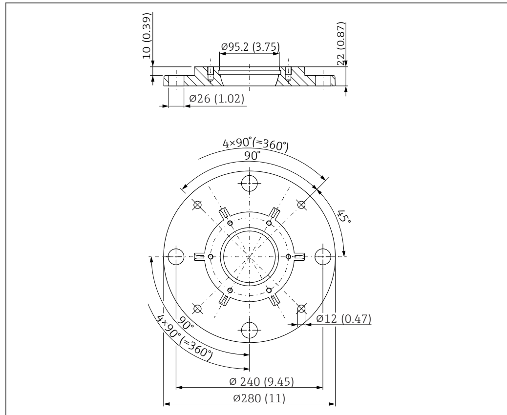
图 53 UNI 6"/DN150/150A 法兰的外形尺寸示意图；适用带角度调节装置的天线。测量单位 mm (in)
