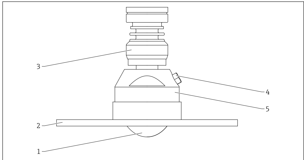
图 73 天线（齐平安装，80 mm (3 in)口径）的材质，带 UNI 法兰和空气吹扫接口。测量单位 mm (in)
