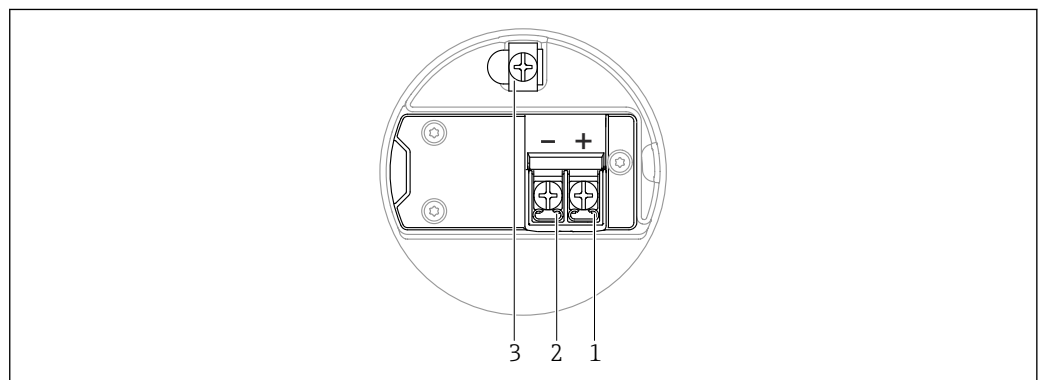
图 4 接线腔中的接线端子分配; 4 ... 20 mA HART; 双腔室外壳
