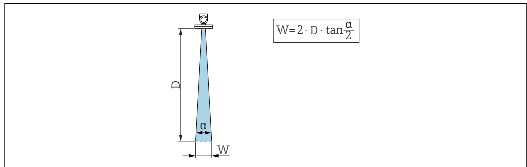
图 20 波束角 \alpha 、距离 D 和波束宽度 W 的相互关系
