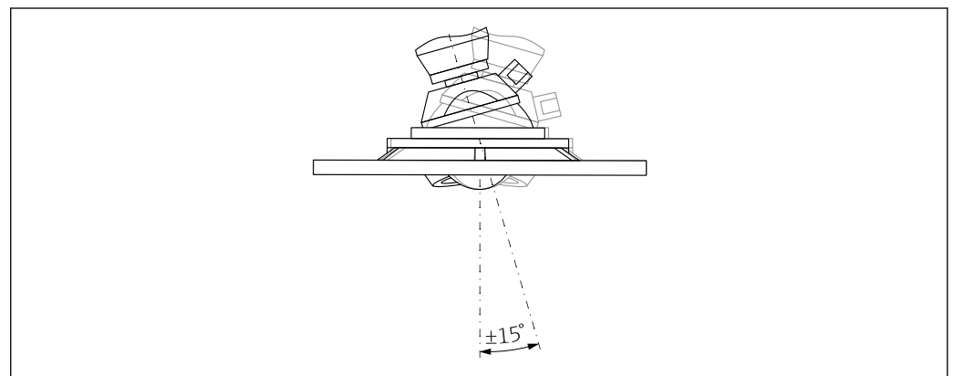
图 18 天线 (齐平安装)，带天线角度调节装置
