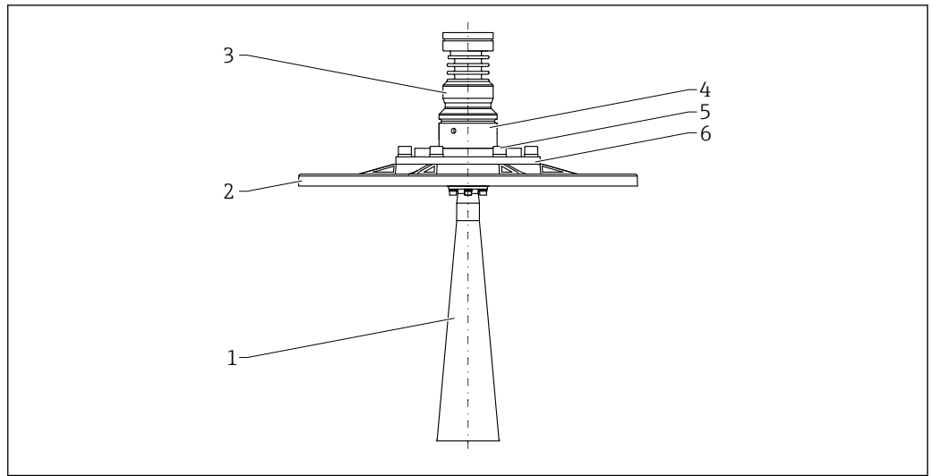
图 70 喇叭天线 (65 mm (2.6 in)口径) 的材质，带 UNI 法兰和天线角度调节装置。测量单位 mm (in)
