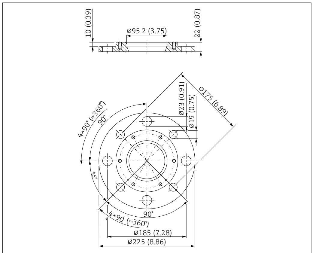
52 UNI 4"/DN100/100A 法兰的外形尺寸示意图；适用带天线角度调节装置的天线。测量单位 mm (in)
