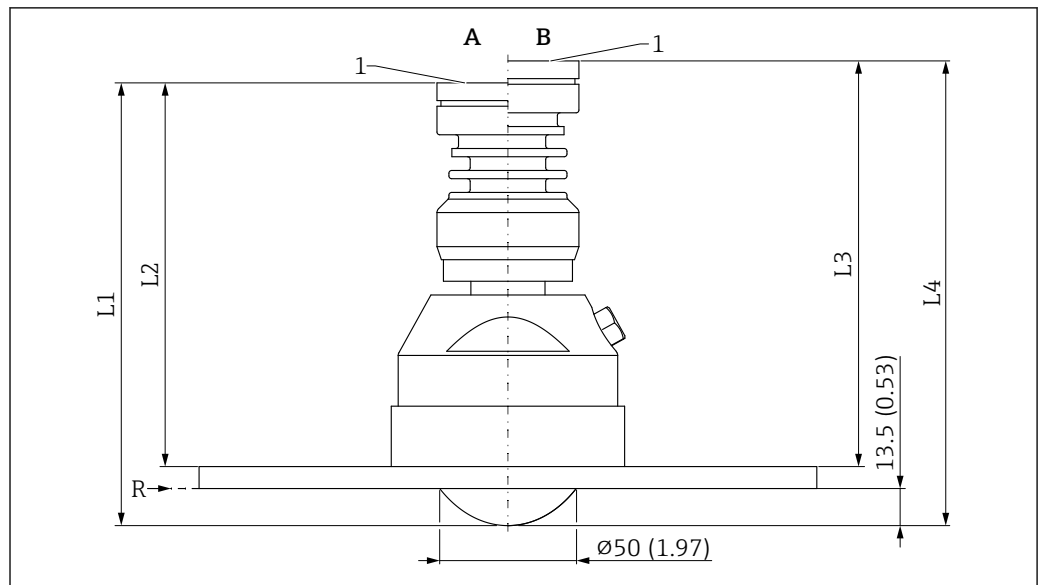
图 61 PTFE 齐平安装天线 (80 mm (3 in)口径) 的外形尺寸示意图; 带 UNI 法兰和空气吹扫接口。测量单位 mm (in)
