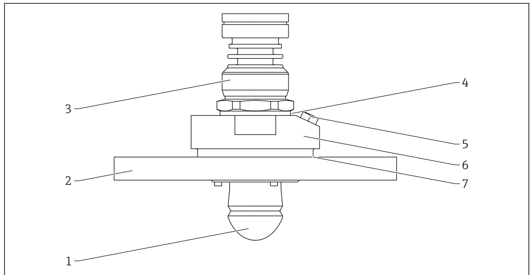
图 71 水滴型天线的材质; 带空气吹扫接口。测量单位 mm (in)
