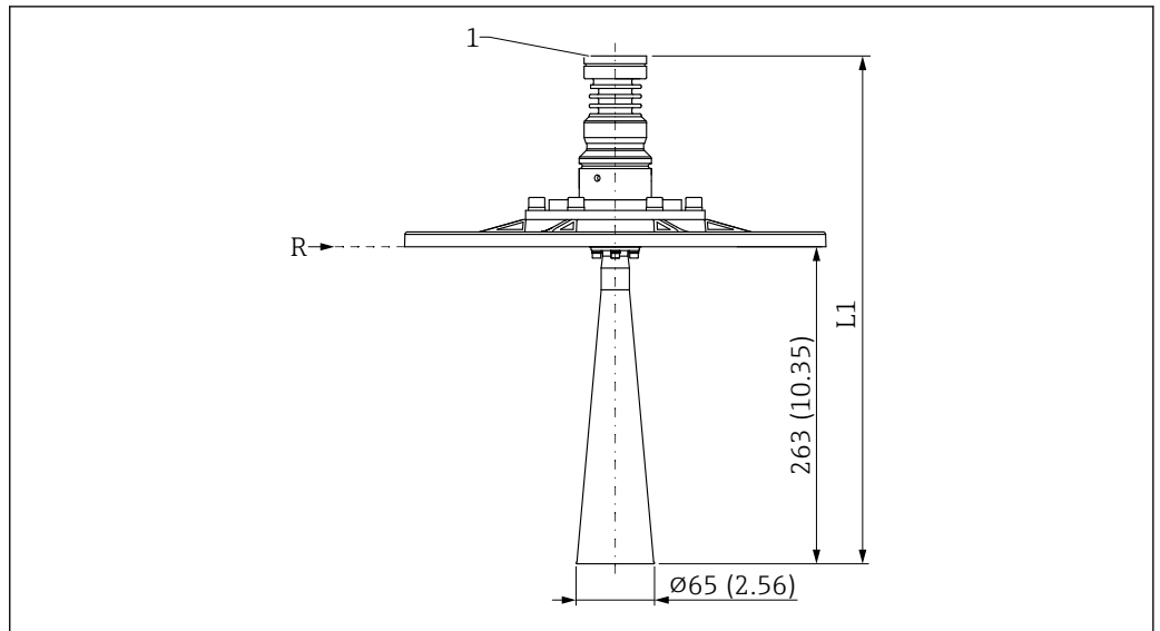
51 DN65 喇叭天线的外形尺寸示意图；带 UNI 法兰和天线角度调节装置。测量单位 mm (in)
