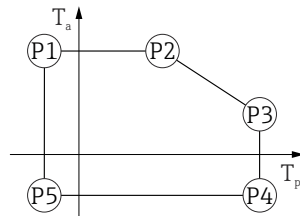
21 塑料外壳; 过程温度范围: -40 ... +80 °C (-40 ... +176 °F)
