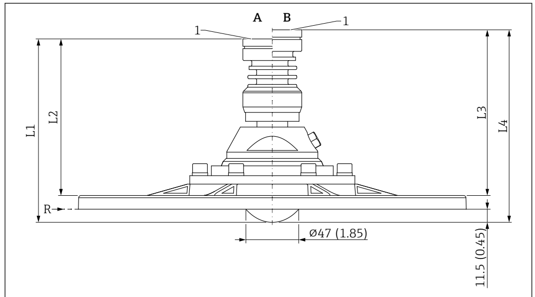
图 64 齐平安装天线 (80 mm (3 in)口径) 的外形尺寸示意图; 带 UNI 法兰、天线角度调节装置和空气吹扫接口。测量单位 mm (in)
