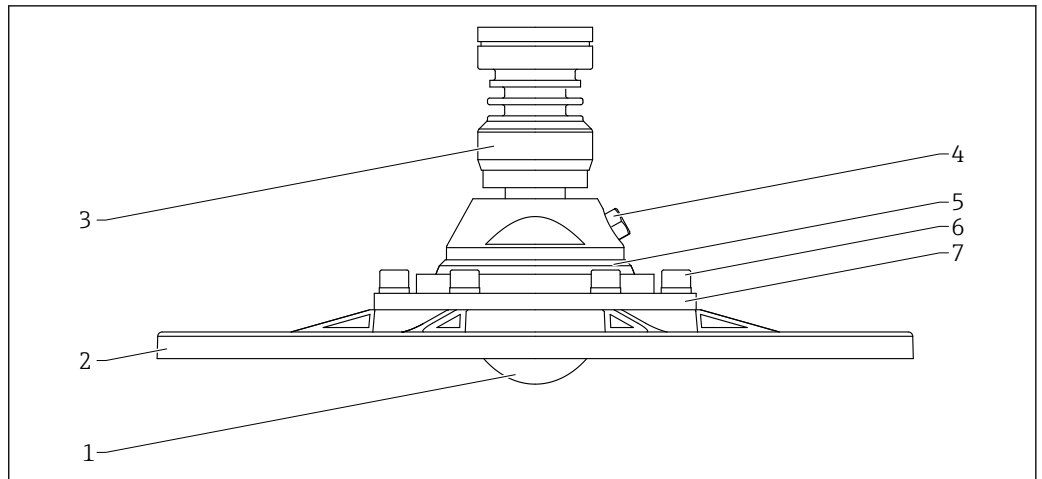
图 74 天线（齐平安装，80 mm (3 in)口径）的材质，带 UNI 法兰、天线角度调节装置和空气吹扫接口
