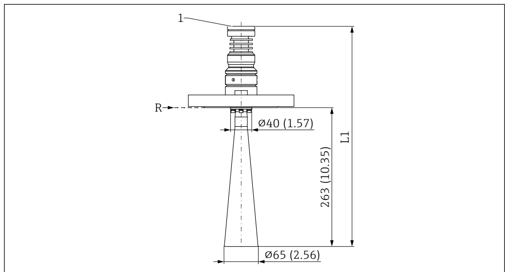
图 50 DN65 喇叭天线的外形尺寸示意图；法兰过程连接。测量单位 mm (in)
