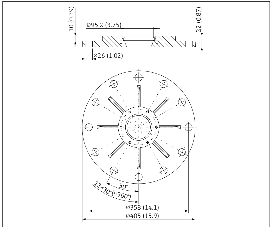
图 55 UNI 10"/DN250/250A 法兰的外形尺寸示意图；适用带天线角度调节装置的天线。测量单位 mm (in)
