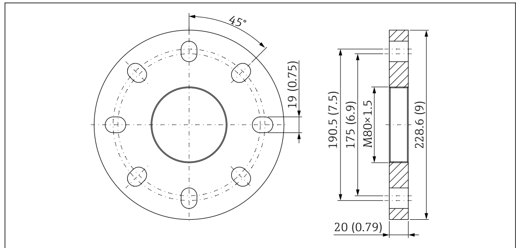
图 58 UNI 4"/DN100/100A 法兰，适用带空气吹扫接口的 PTFE 水滴型天线 (50 mm (2 in)口径)。测量单位 mm (in)
