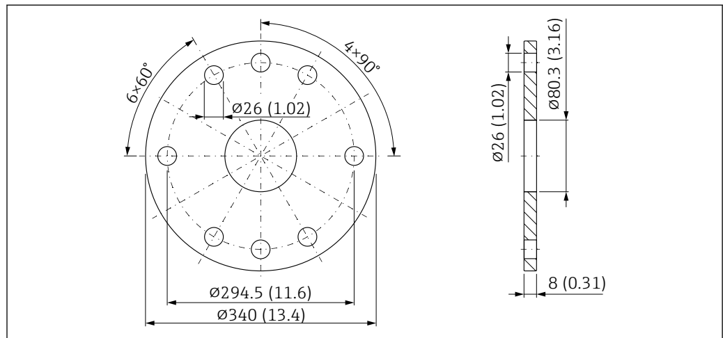
图 62 UNI 8"/DN200/200A 法兰的外形尺寸示意图; 适用带空气吹扫接口的 DN80 天线。测量单位 mm (in)
