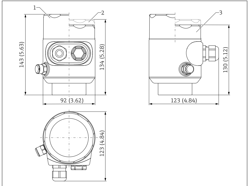
图 46 316L 单腔室外壳（卫生型）的外形尺寸示意图；包括 M20 接头和塑料插头。测量单位 mm (in)
