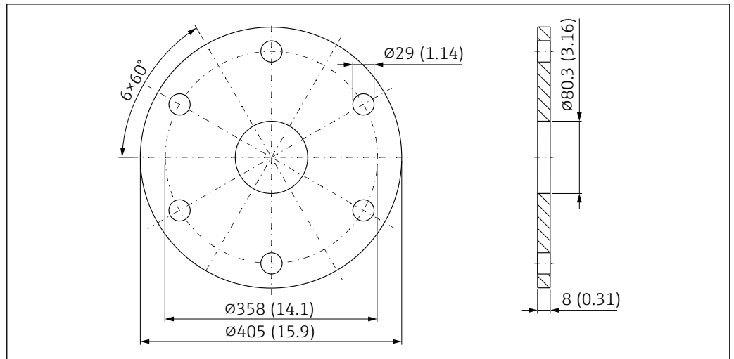
图 63 UNI 10"/DN250/250A 法兰的外形尺寸示意图; 适用带空气吹扫接口的 DN80 天线。测量单位 mm (in)
