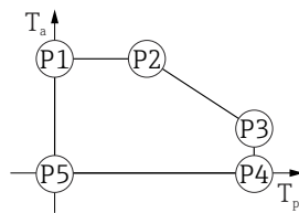
22 塑料外壳; 过程温度范围: 0 ... +80 °C (+32 ... +176 °F), 适用 CSA C/US 认证型仪表
