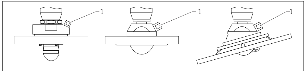
图 19 天线，带空气吹扫接口
