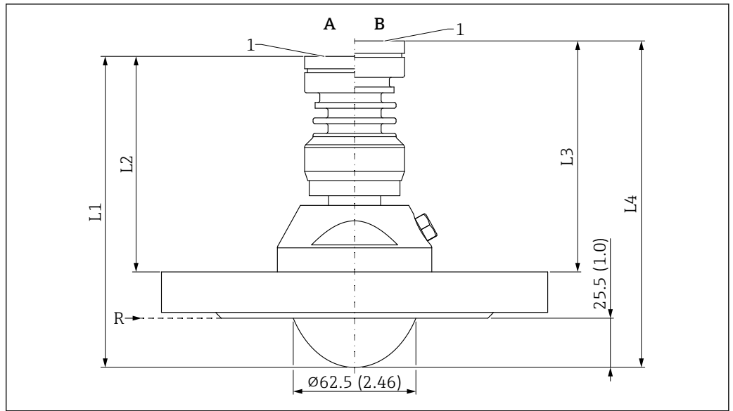
图 60 PTFE 齐平安装天线 (80 mm (3 in) 口径) 的外形尺寸示意图; 带标准法兰和空气吹扫接口。测量单位 mm (in)
