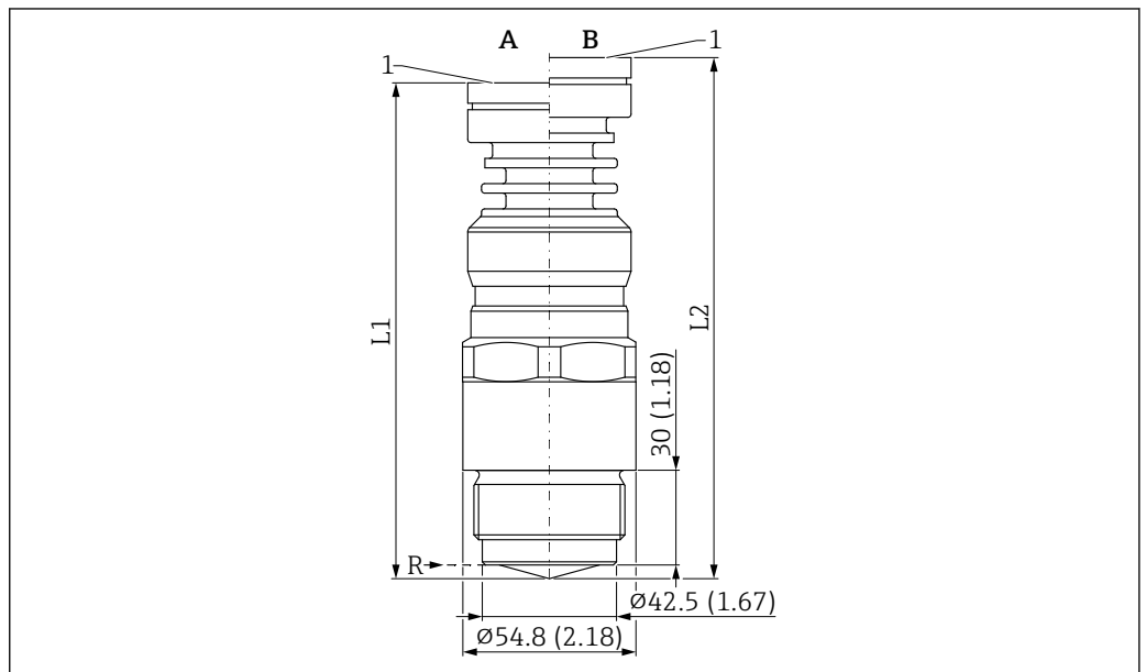
图 57 PEEK 一体式天线 (40 mm (1.5 in) 口径) 的外形尺寸示意图; 1-½"螺纹过程连接。测量单位 mm (in)
