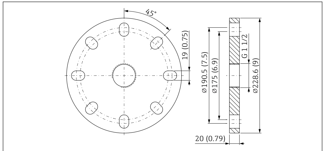
图 49 UNI 4"/DN100/100A 法兰的外形尺寸示意图。测量单位 mm (in)
