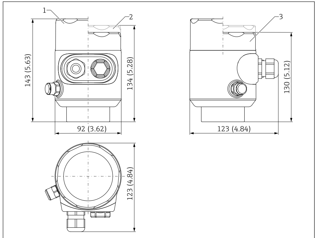
图 42 316L 单腔室外壳 (卫生型) 的外形尺寸示意图; 包括 M20 接头和塑料插头。测量单位 mm (in)
