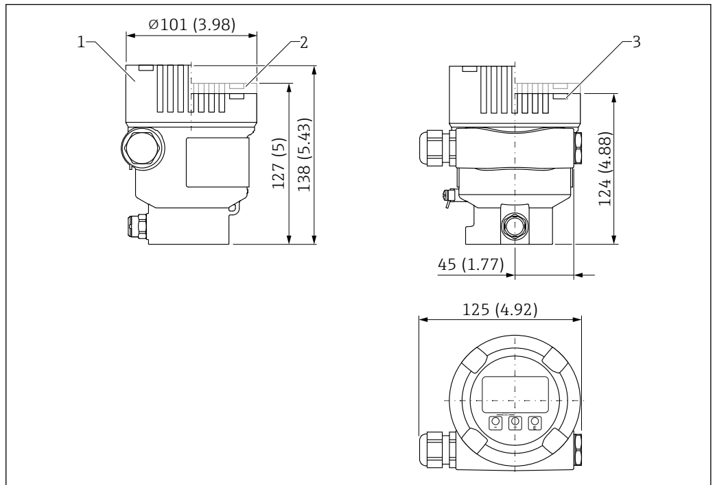
41 单腔室铝外壳（带涂层）的外形尺寸示意图；包括 M20 接头和塑料插头。测量单位 mm (in)
