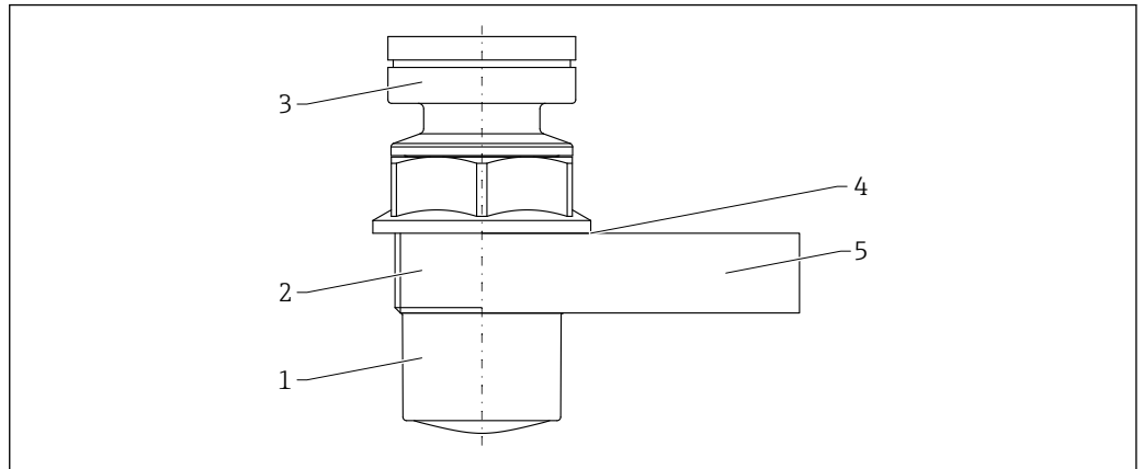
☑ 58 PVDF 全密封天线 (40 mm (1.5 in)口径) 的材质
