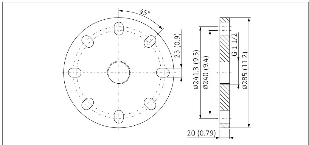
图 55 UNI 6"/DN150/150A 法兰的外形尺寸示意图。测量单位 mm (in)
