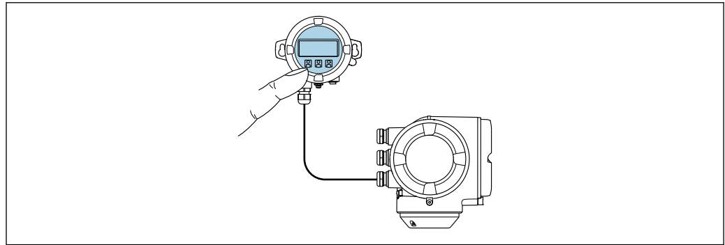
图 42 通过远传显示单元 DKX001 操作
