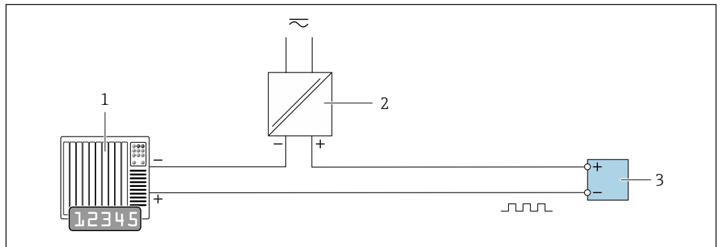
图 18 接线示例：脉冲/频率输出（无源信号）
