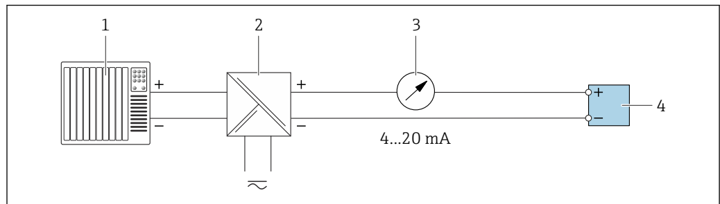
17 Ejemplo de conexión de salida de corriente de 4-20 mA (pasiva)
