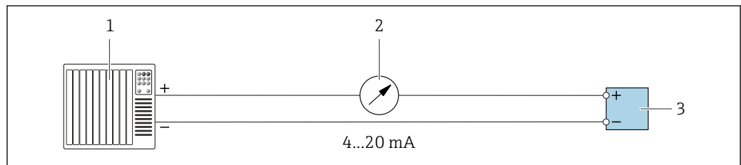
16 Ejemplo de conexión de salida de corriente de 4-20 mA (activa)
