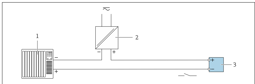
22 Ejemplo de conexión de una salida de relé (pasiva)
