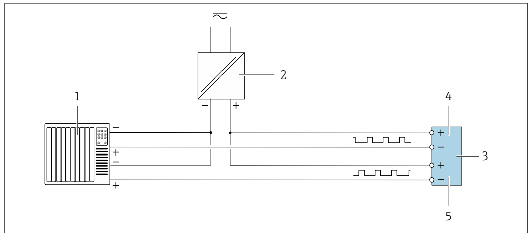
21 Ejemplo de conexión de una doble salida de pulsos (pasiva)
