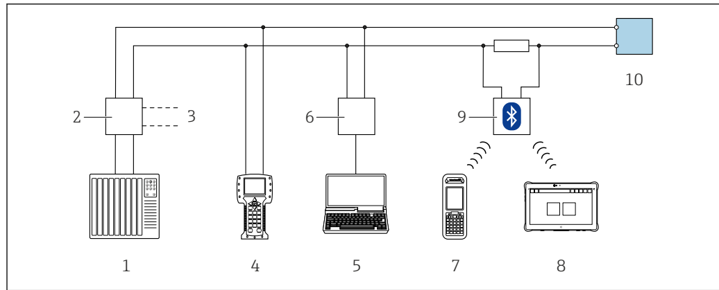
30 Opciones para la configuración a distancia mediante el protocolo HART (pasivo)
