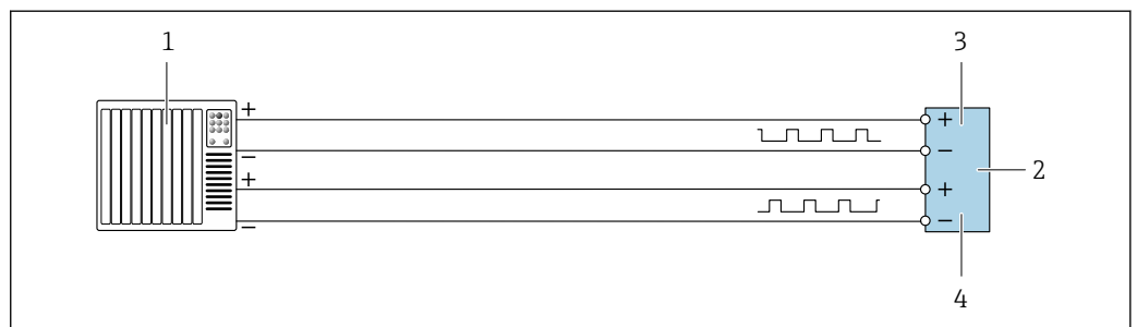
20 Exemplo de conexão para saída de pulso duplo (ativa)
