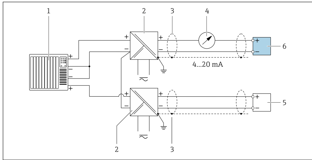
15 Exemplo de conexão para entrada HART com um ponto comum negativo (passivo)
