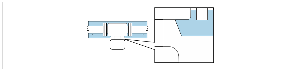
7 Aislamiento térmico con cuello prolongado expuesto
