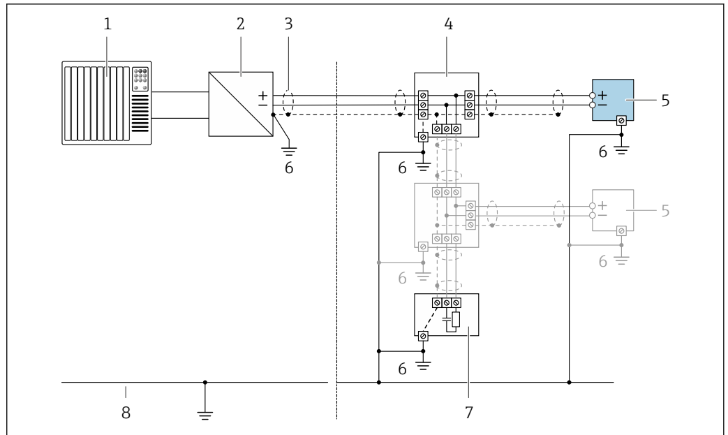
15 Ejemplo de conexión para PROFIBUS PA
