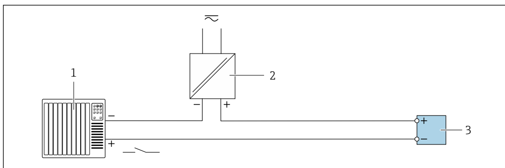
図 27 ステータス入力の接続例
