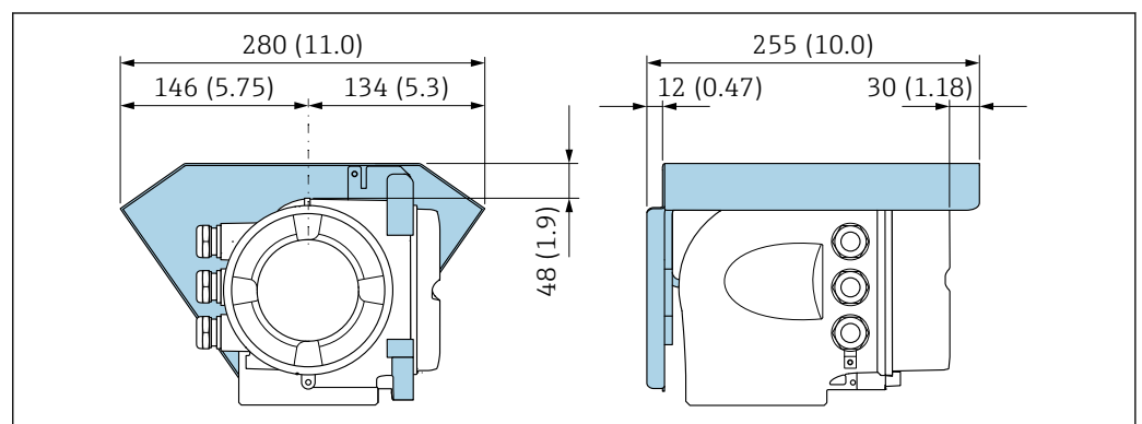
图 10 Proline 500 变送器的防护罩的外形尺寸图；单位：mm (in)
