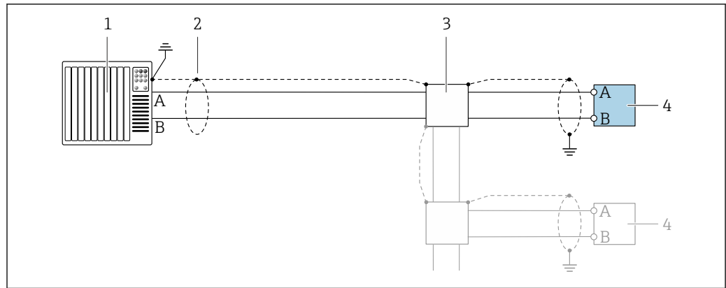
図 18 Modbus RS485（非危険場所および Zone 2; Class I, Division 2 用）の接続例
