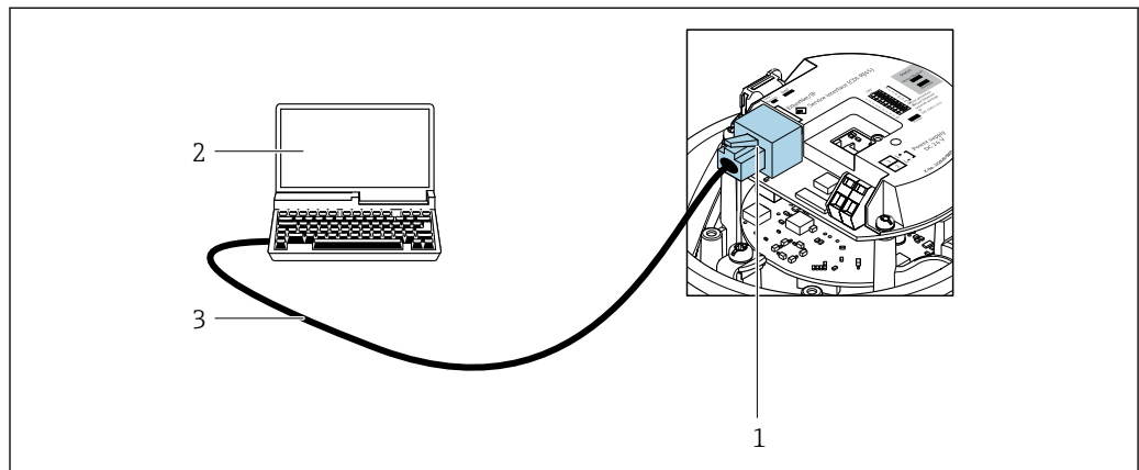
▣ 19 Connessione per codice d'ordine per "Uscita", opzione R: PROFINET
