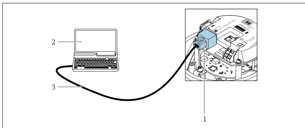
14 Connessione per codice d'ordine per "Uscita", opzione R: PROFINET
