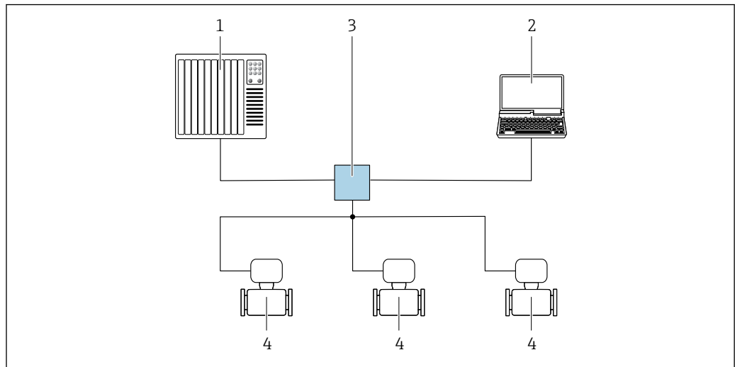
▣ 18 Opzioni per il funzionamento a distanza mediante rete PROFINET: topologia a stella
