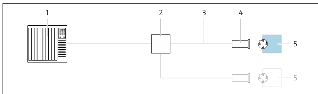
11 Esempio di collegamento per PROFINET
