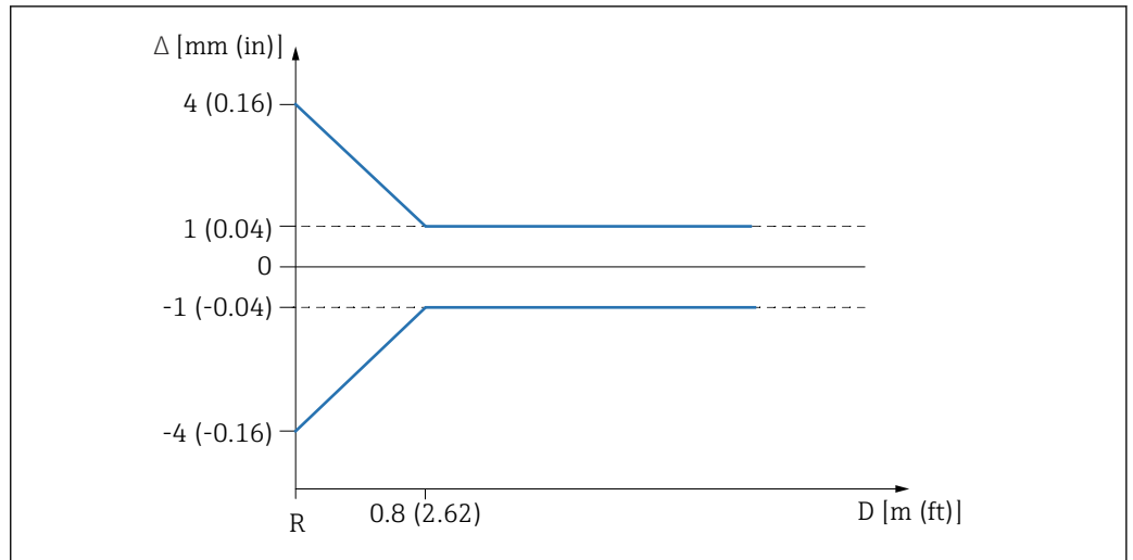
图 8 近距离测量时的最大测量误差
