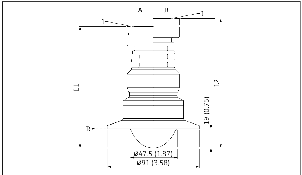
50 PTFE 涂层天线 (齐平安装, 50 mm (2 in)口径) 的外形尺寸示意图; 带 ISO2852 Tri-Clamp DN70-76.1 (3")卡箍。测量单位 mm (in)
