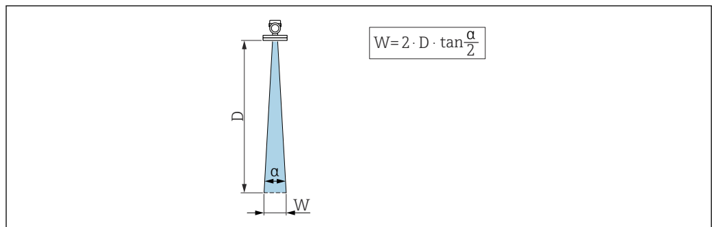
图 9 波束角 α、距离 D 和波束宽度 W 的相互关系
