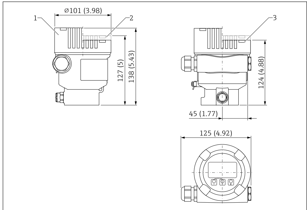
图 41 单腔室铝外壳 (带涂层) 的外形尺寸示意图; 包括 M20 接头和塑料插头。测量单位 mm (in)
