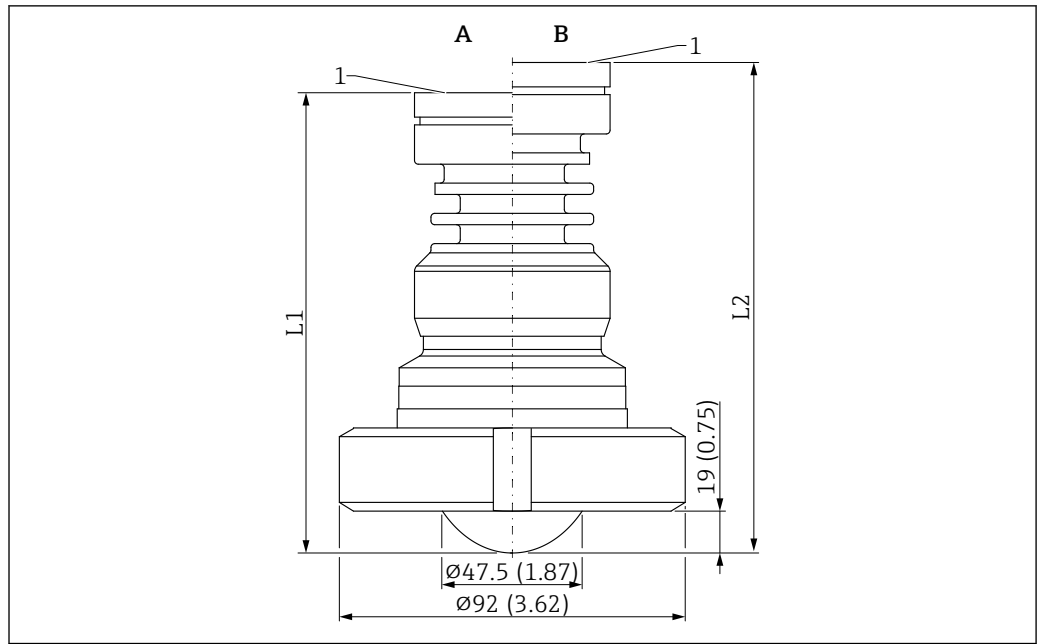
图 47 PTFE 涂层天线 (齐平安装, 50 mm (2 in)口径) 的外形尺寸示意图; 带 DIN11851 开槽螺母。测量单位 mm (in)
