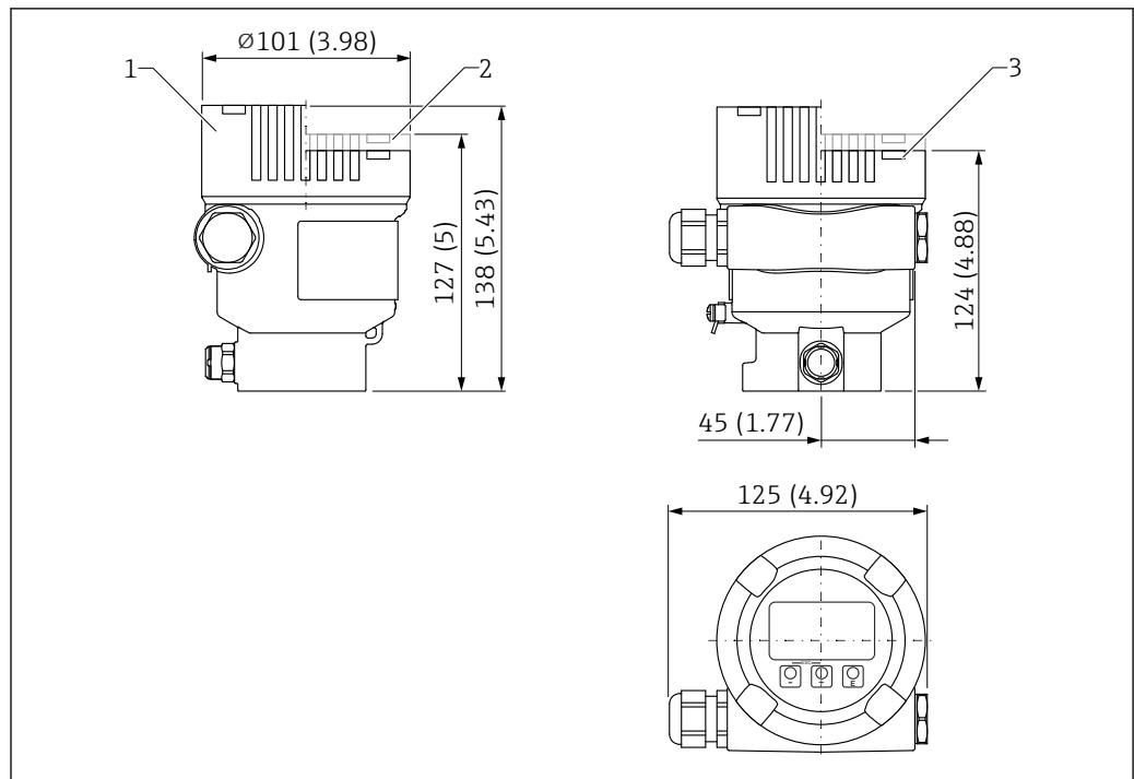
图 42 单腔室铝外壳 (带涂层) 的外形尺寸示意图; 包括 M20 接头和塑料插头。测量单位 mm (in)
