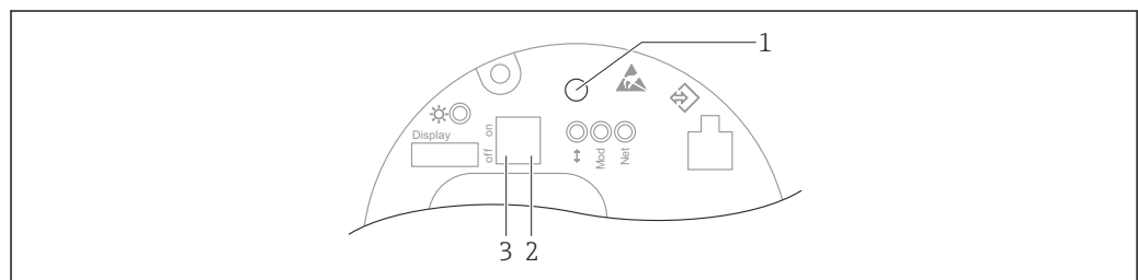
图 64 Ethernet-APL 电子插件上的操作按键和 DIP 开关
