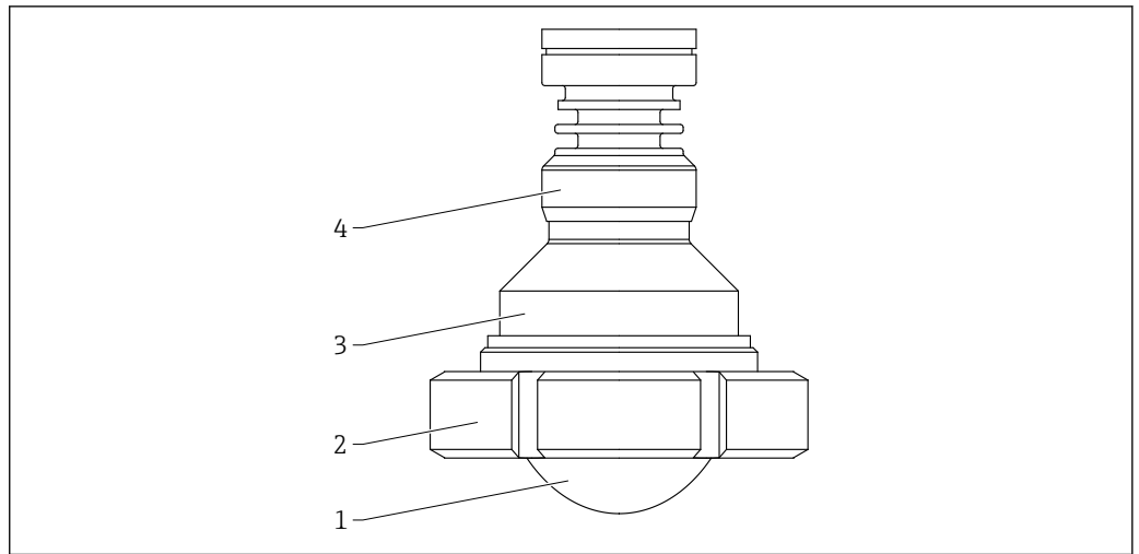
☑ 58 涂层天线的材质；齐平安装，80 mm (3 in)口径，带 DIN11851 开槽螺母。测量单位 mm (in)
