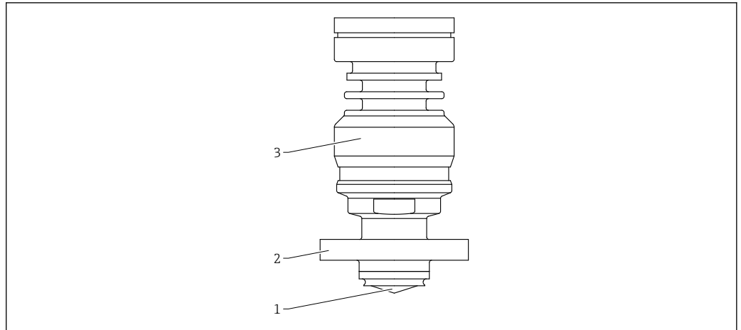
图 62 PEEK 涂层天线的材质；齐平安装，20 mm (0.75 in)口径，带 NEUMO BioControl D25 卫生型连接
