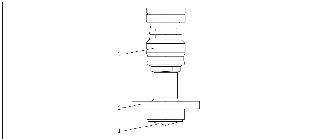
图 63 PEEK 涂层天线的材质；齐平安装，40 mm (1.5 in)口径，带 NEUMO BioControl D50 卫生型连接
