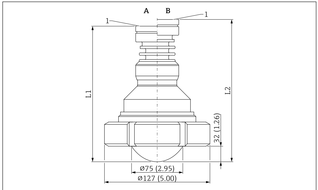
49 PTFE 涂层天线 (齐平安装, 80 mm (3 in)口径) 的外形尺寸示意图; 带 DIN11851 开槽螺母。测量单位 mm (in)
