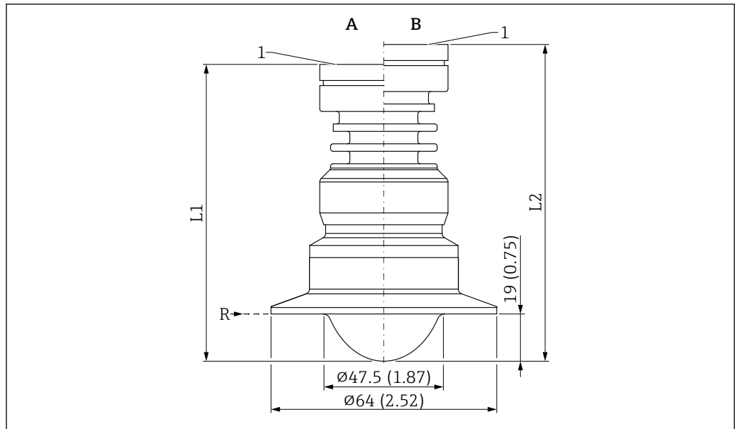
图 50 PTFE 涂层天线（齐平安装，50 mm (2 in)口径）的外形尺寸示意图；带 ISO2852 Tri-Clamp DN51 (2")卡箍。测量单位 mm (in)
