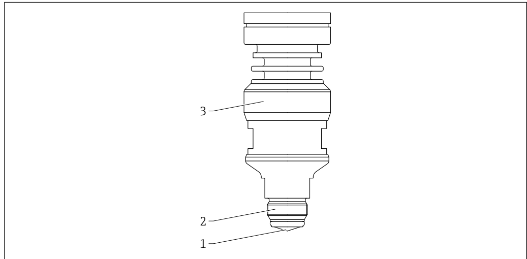
图 56 PEEK 一体式天线的材质; 20 mm (0.75 in)口径, 带 M24 螺纹过程连接
