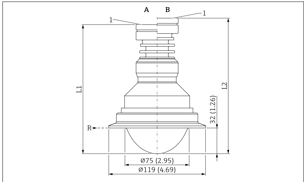
图 52 PTFE 涂层天线（齐平安装，80 mm (3 in)口径）的外形尺寸示意图；带 ISO2852 Tri-Clamp DN101.6 (4")卡箍。测量单位 mm (in)
