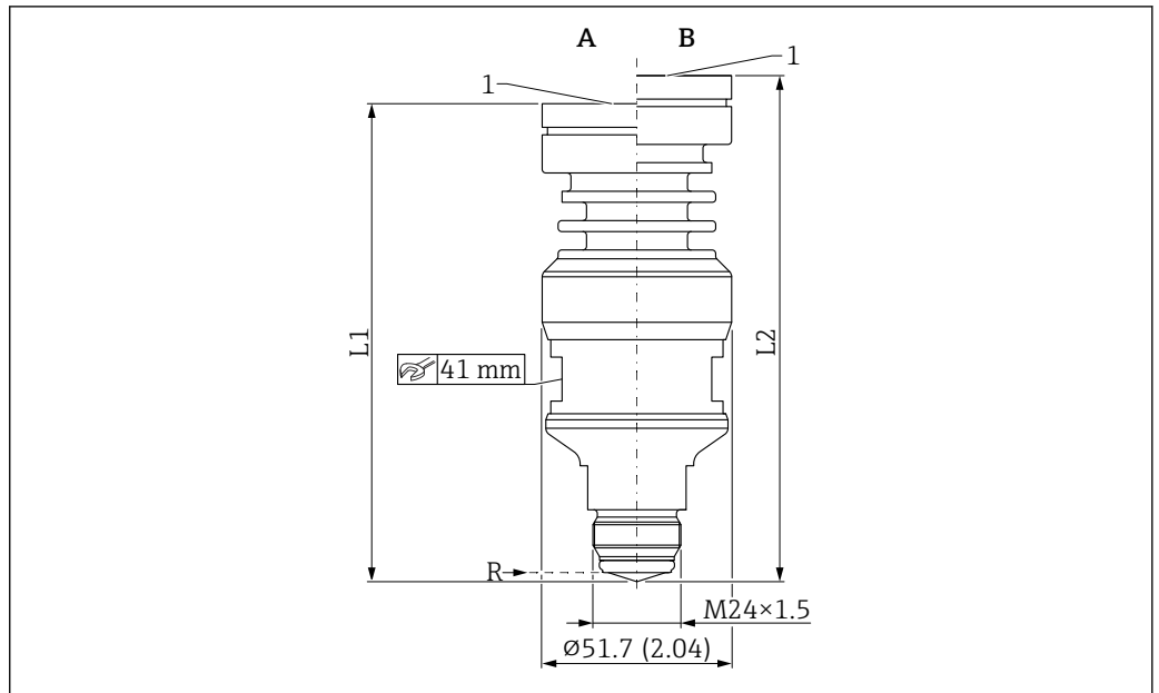
47 PEEK 一体式天线的外形尺寸示意图；20 mm (0.75 in)口径，带 M24 螺纹过程连接。测量单位 mm (in)
