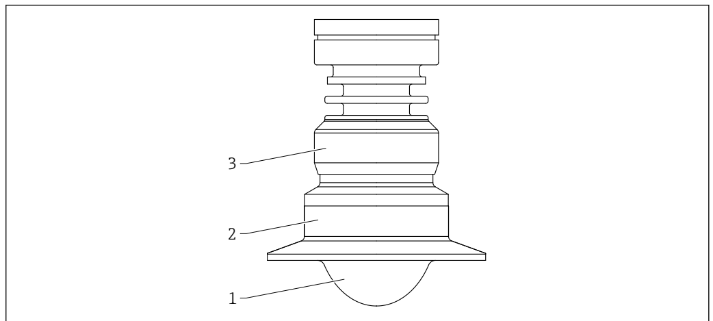
☑ 59 PTFE 涂层天线的材质；齐平安装，50 mm (2 in)口径，带 ISO2852 Tri-Clamp 卡箍。测量单位 mm (in)
