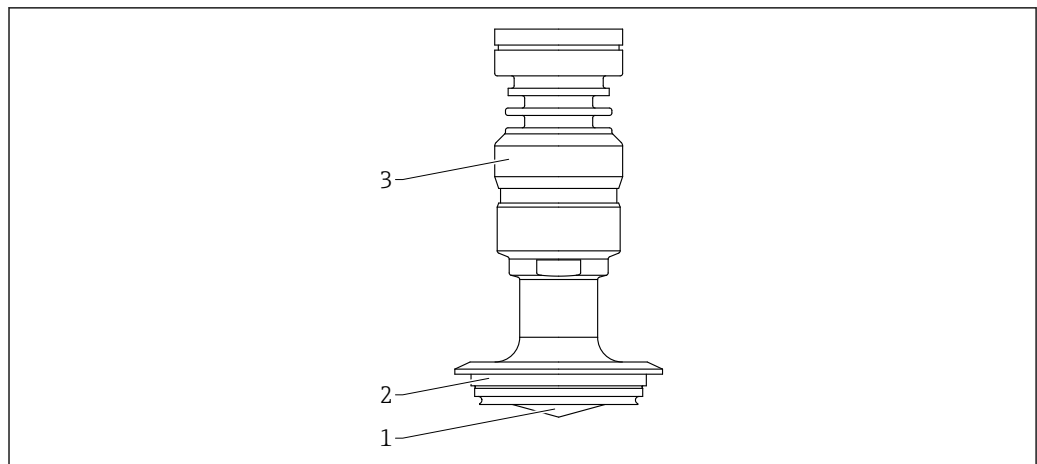
▣ 61 PEEK 涂层天线的材质；齐平安装，40 mm (1.5 in)口径，带 Varivent N DN65-162 接头
