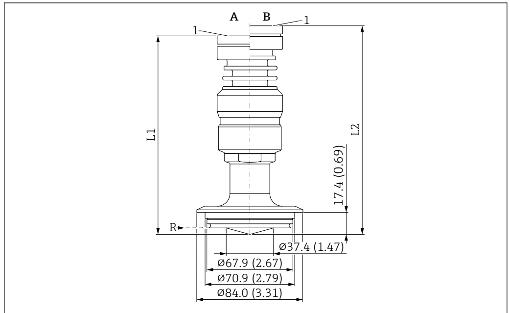
53 PEEK 涂层天线的外形尺寸示意图；齐平安装，40 mm (1.5 in) 口径，带 Varivent N DN65-162 接头。 测量单位 mm (in)
