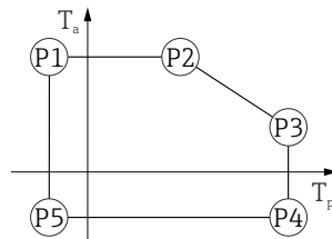
☐ 34 316L 外壳, 卫生型; 过程温度范围: -40 ... +200 °C (-40 ... +392 °F)
