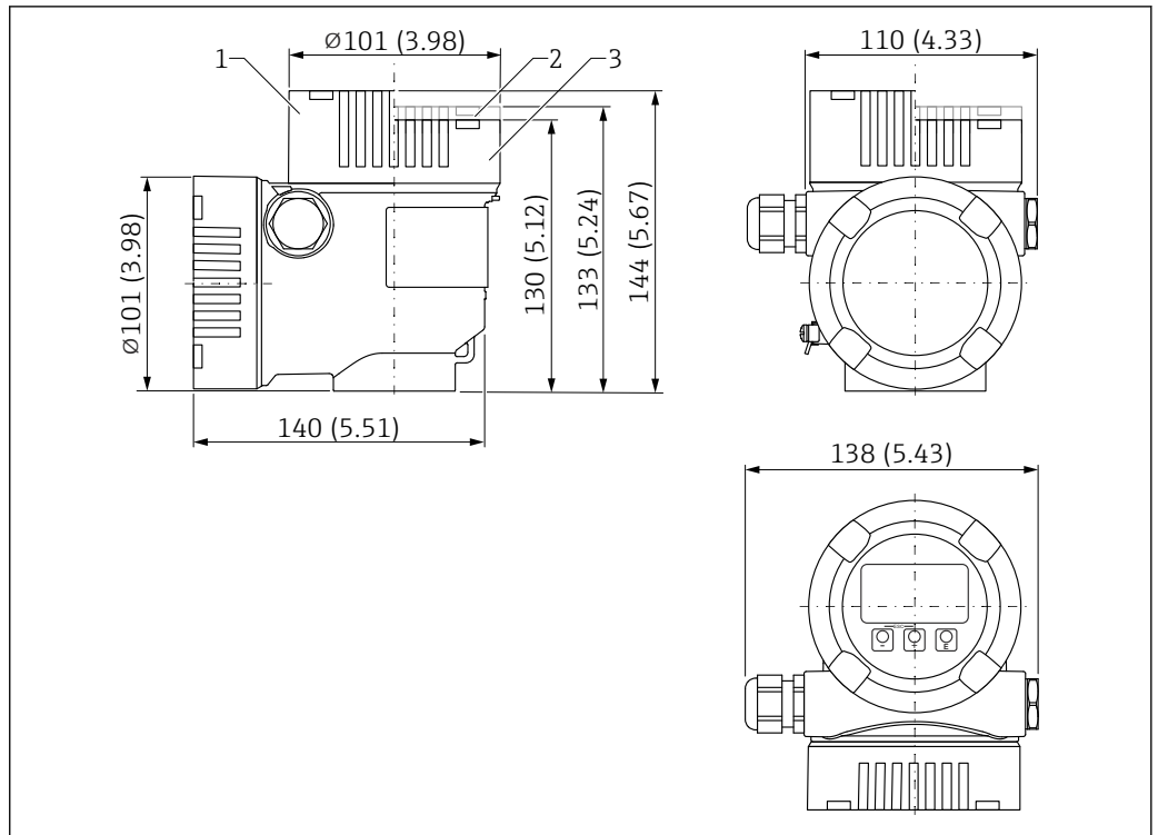
图 40 L 型双腔室 316L 外壳的外形尺寸示意图；包括 M20 接头和塑料插头。测量单位 mm (in)
