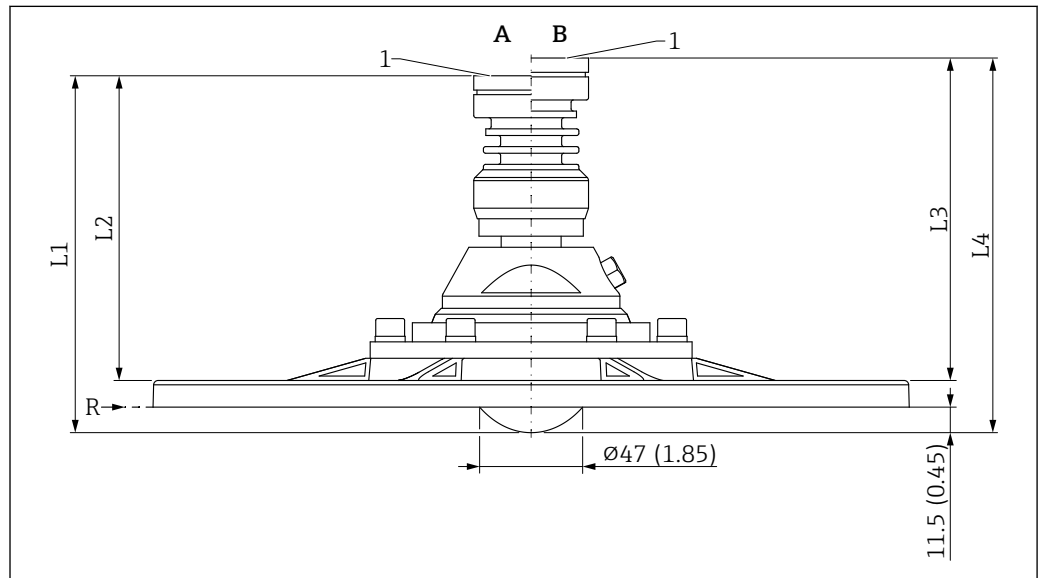
图 55 齐平安装天线 (80 mm (3 in) 口径) 的外形尺寸示意图; 带 UNI 法兰、天线角度调节装置和空气吹扫接口。测量单位 mm (in)
