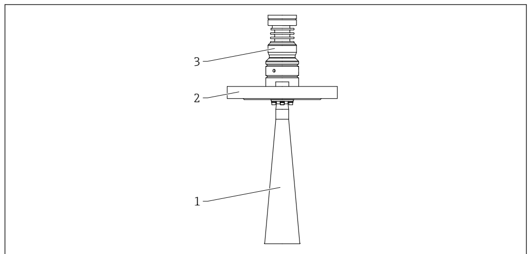
☑ 60 喇叭天线 (65 mm (2.6 in) 口径) 的材质。测量单位 mm (in)
