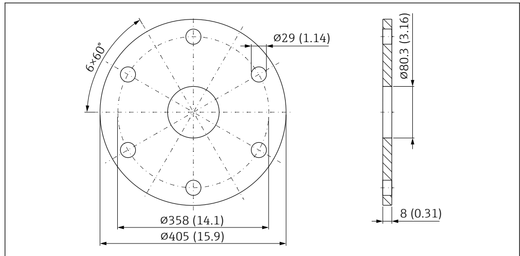
图 54 UNI 10"/DN250/250A 法兰的外形尺寸示意图; 适用带空气吹扫接口的 DN80 天线。测量单位 mm (in)
