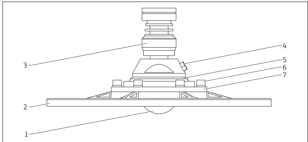
图 65 天线（齐平安装，80 mm (3 in)口径）的材质，带 UNI 法兰、天线角度调节装置和空气吹扫接口
