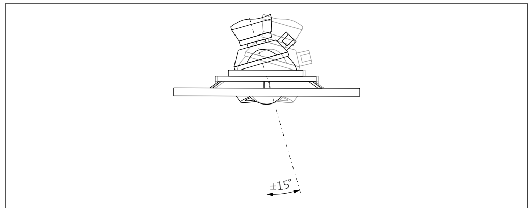
图 9 天线 (齐平安装)，带天线角度调节装置
