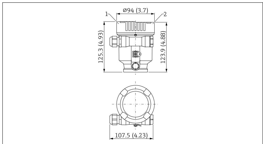
图 35 单腔室塑料外壳的外形尺寸示意图; 包括 M20 接头和塑料插头。测量单位 mm (in)
