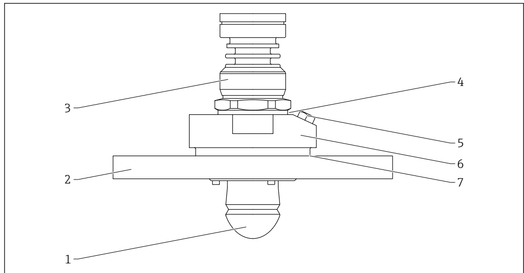
图 62 水滴型天线的材质；带空气吹扫接口。测量单位 mm (in)
