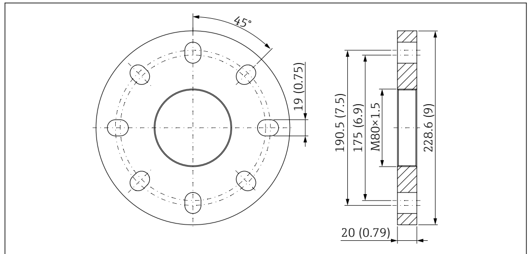
49 UNI 4"/DN100/100A 法兰, 适用带空气吹扫接口的 PTFE 水滴型天线 (50 mm (2 in) 口径)。测量单位 mm (in)
