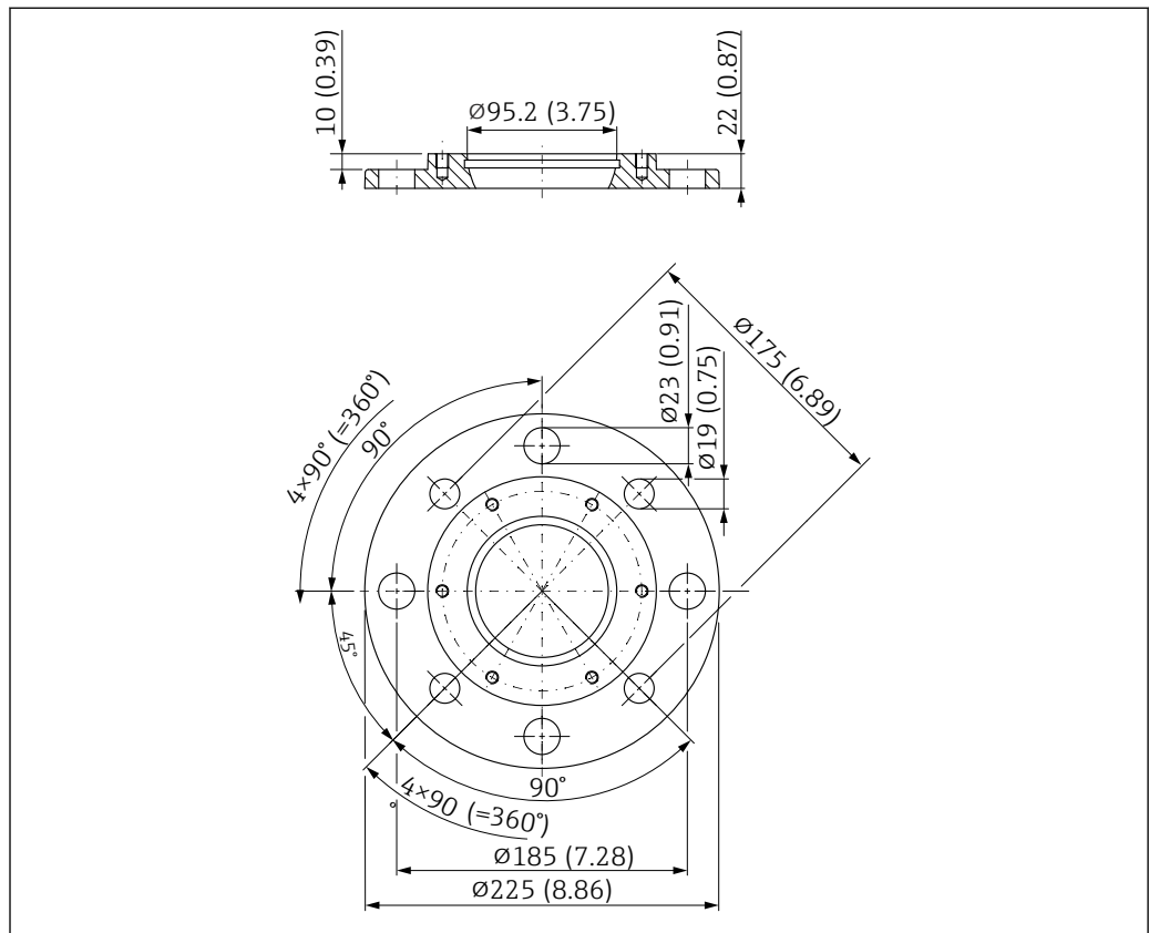
图 43 UNI 4"/DN100/100A 法兰的外形尺寸示意图；适用带天线角度调节装置的天线。测量单位 mm (in)
