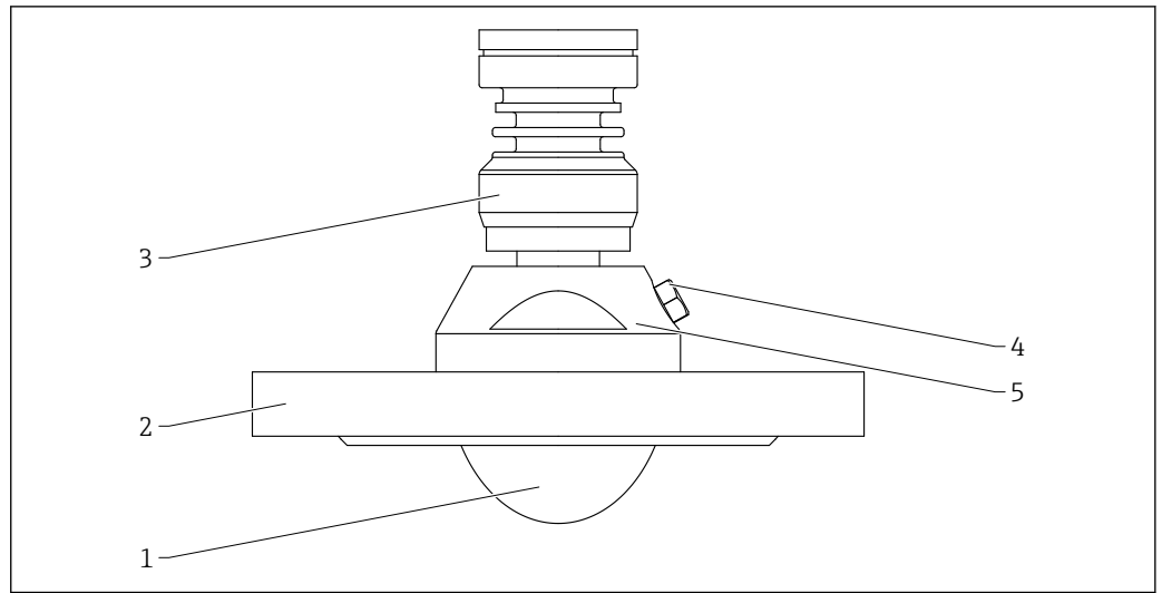
图 63 天线（齐平安装，80 mm (3 in)口径）的材质，带法兰和空气吹扫接口。测量单位 mm (in)
