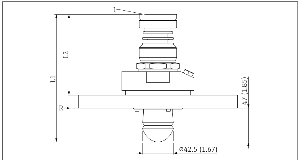
图 47 PTFE 水滴型天线 (50 mm (2 in)口径) 的外形尺寸示意图; 带 UNI 法兰和空气吹扫接口。测量单位 mm (in)
