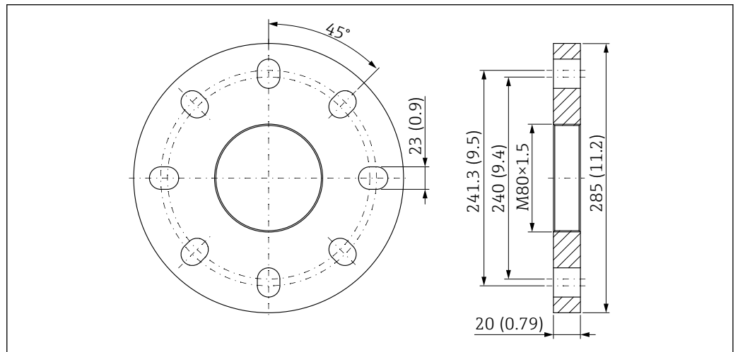
50 UNI 6"/DN150/150A 法兰, 适用带空气吹扫接口的 PTFE 水滴型天线 (50 mm (2 in) 口径)。测量单位 mm (in)
