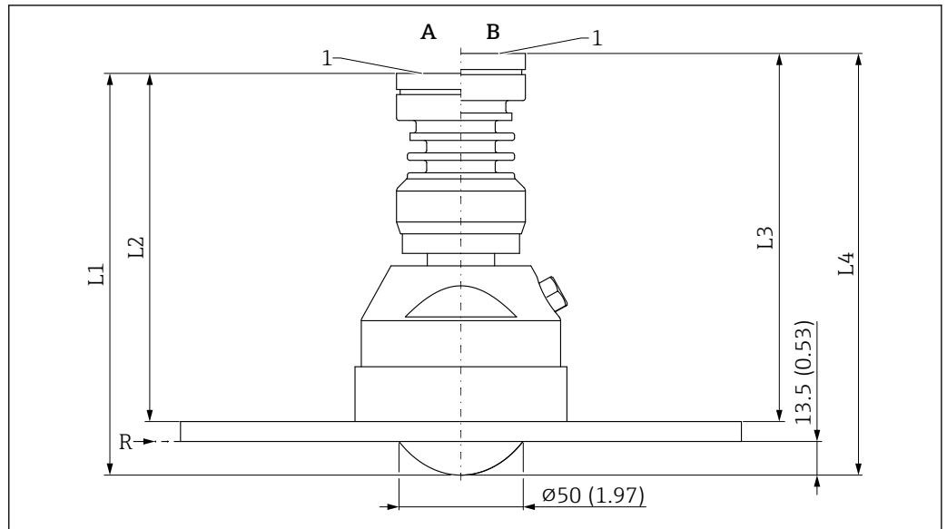
图 52 PTFE 齐平安装天线 (80 mm (3 in) 口径) 的外形尺寸示意图; 带 UNI 法兰和空气吹扫接口。测量单位 mm (in)
