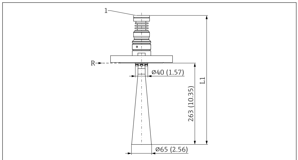
图 41 DN65 喇叭天线的外形尺寸示意图；法兰过程连接。测量单位 mm (in)
