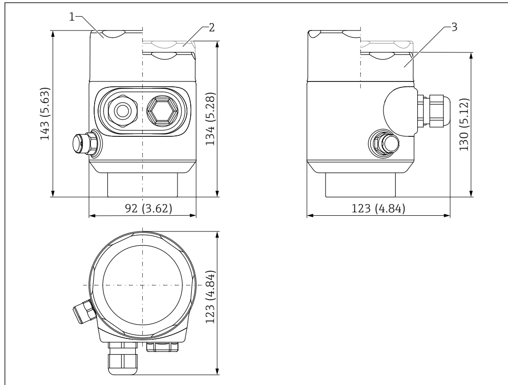
图 37 316L 单腔室外壳（卫生型）的外形尺寸示意图；包括 M20 接头和塑料插头。测量单位 mm (in)
