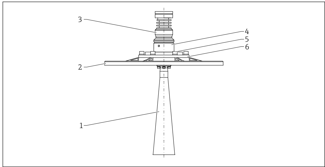
图 61 喇叭天线 (65 mm (2.6 in)口径) 的材质，带 UNI 法兰和天线角度调节装置。测量单位 mm (in)
