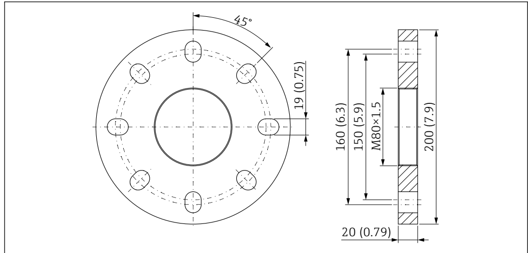
图 48 UNI 3"/DN80/80A 法兰，适用带空气吹扫接口的 PTFE 水滴型天线 (50 mm (2 in)口径)。测量单位 mm (in)
