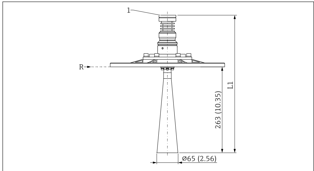
图 42 DN65 喇叭天线的外形尺寸示意图；带 UNI 法兰和天线角度调节装置。测量单位 mm (in)
