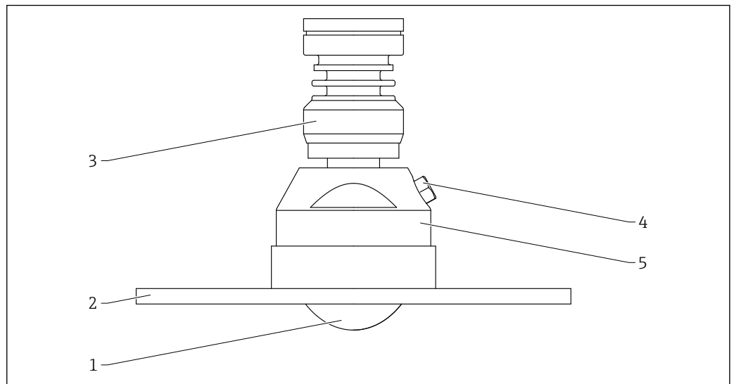
图 64 天线（齐平安装，80 mm (3 in)口径）的材质，带 UNI 法兰和空气吹扫接口。测量单位 mm (in)
