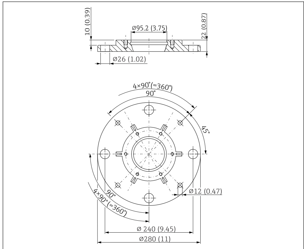
图 57 UNI 6"/DN150/150A 法兰的外形尺寸示意图；适用带角度调节装置的天线。测量单位 mm (in)
