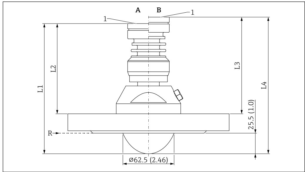
图 51 PTFE 齐平安装天线 (80 mm (3 in) 口径) 的外形尺寸示意图; 带标准法兰和空气吹扫接口。测量单位 mm (in)
