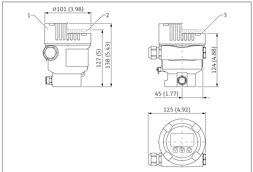
图 36 单腔室铝外壳（带涂层）的外形尺寸示意图；包括 M20 接头和塑料插头。测量单位 mm (in)
