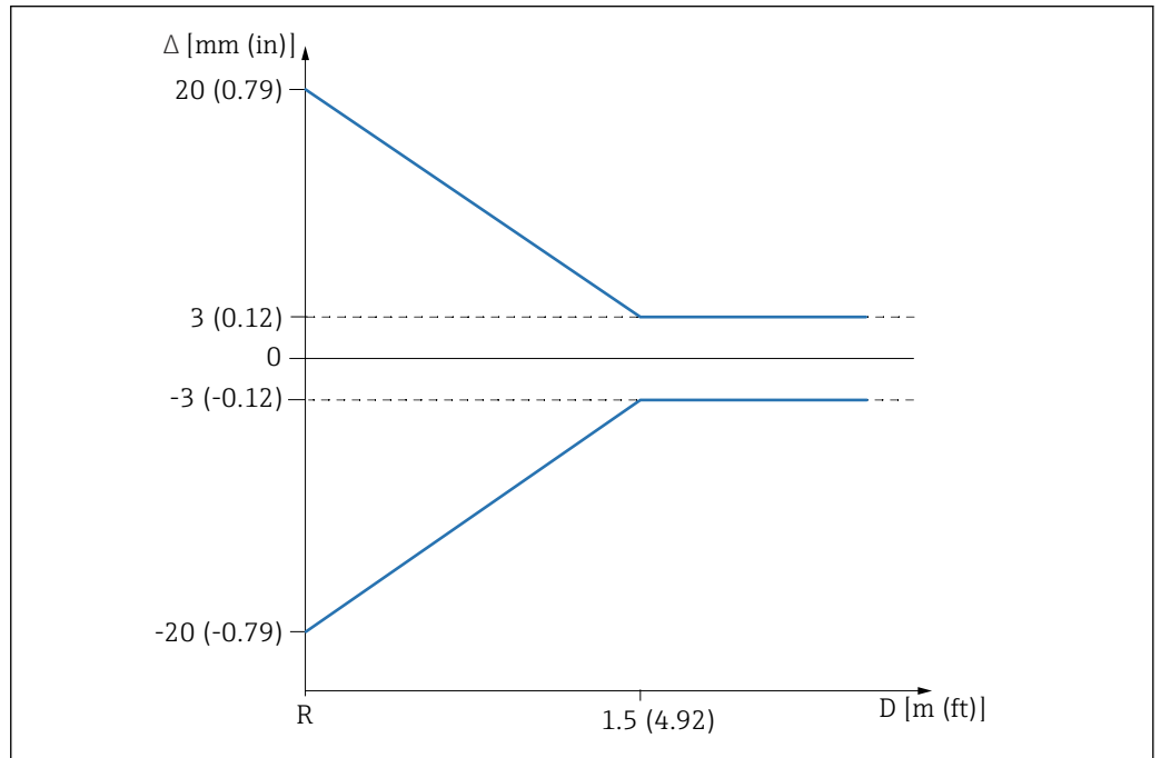
图 7 近距离测量时的最大测量误差
