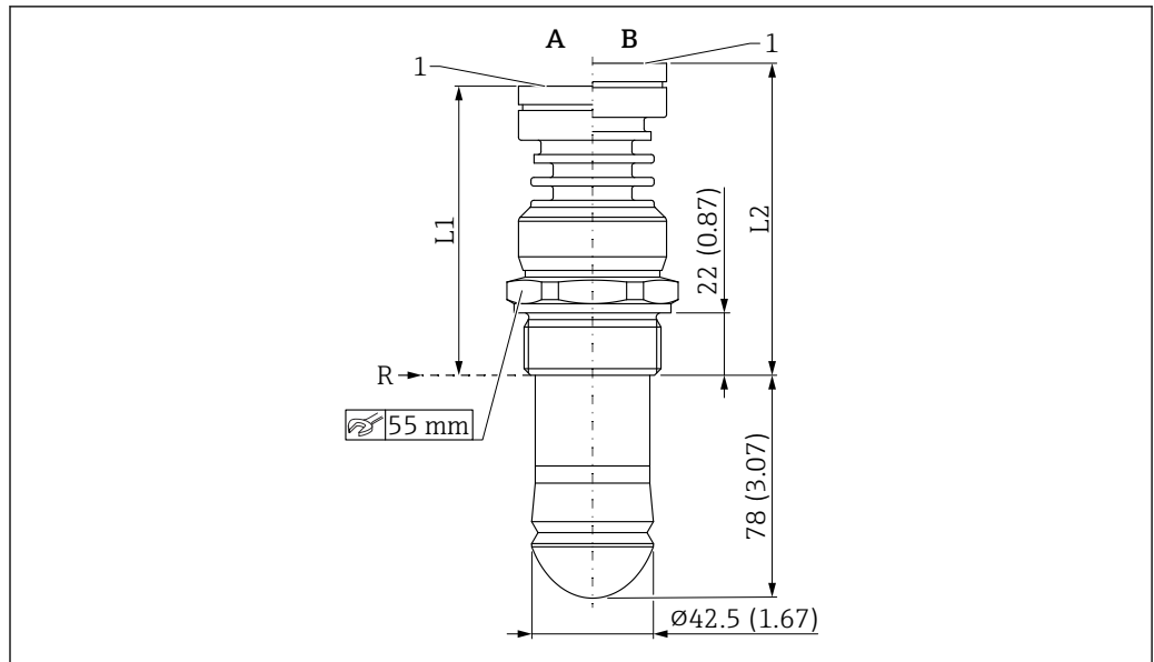
図 52 ドリップオフアンテナ 50 mm (2 in) (ネジ込みプロセス接続) の寸法
