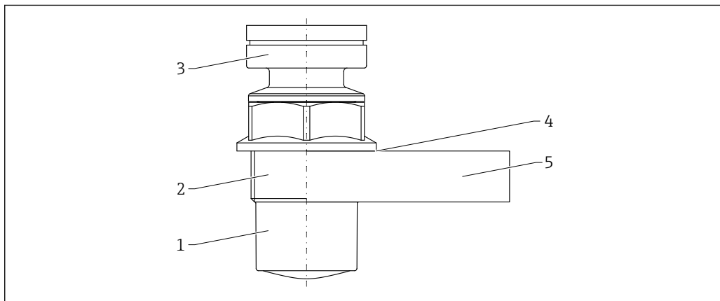
☐ 59 材質；被覆アンテナ PVDF、40 mm (1.5 in)
