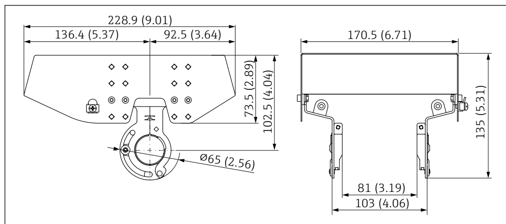
図 66 日除けカバー、SUS 316L 相当、XW112 の寸法。測定単位 mm (in)
