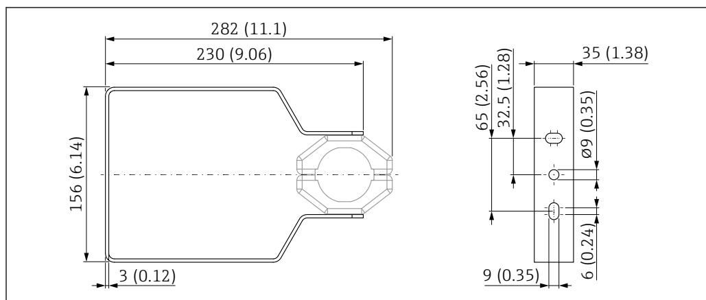
図 69 寸法；調整可能な取付ブラケット FMR6xB。測定単位 mm (in)
