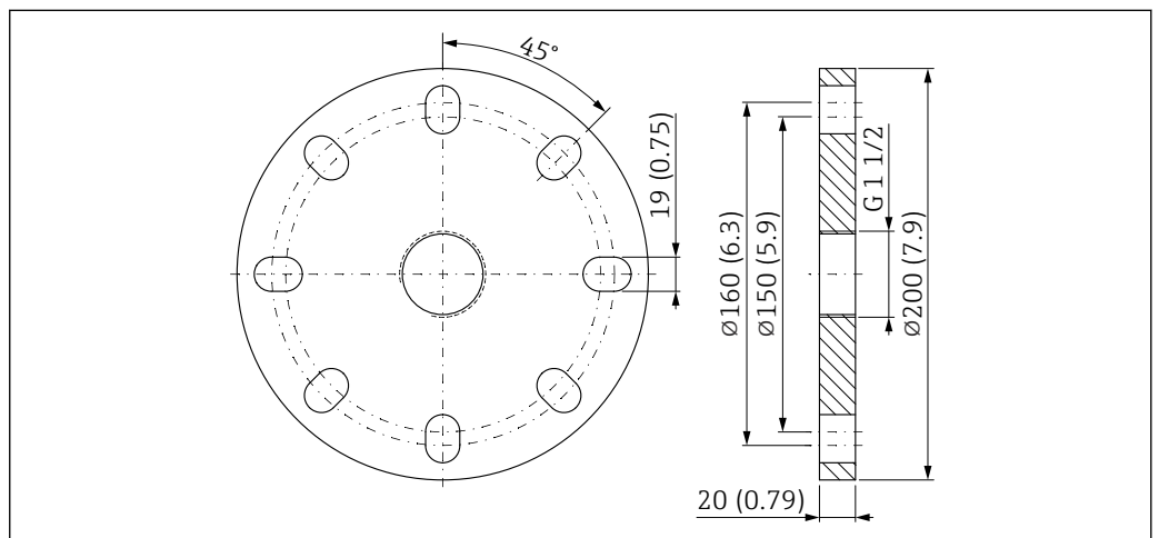
図 54 UNI フランジ 3"/DN80/80A の寸法。測定単位 mm (in)
