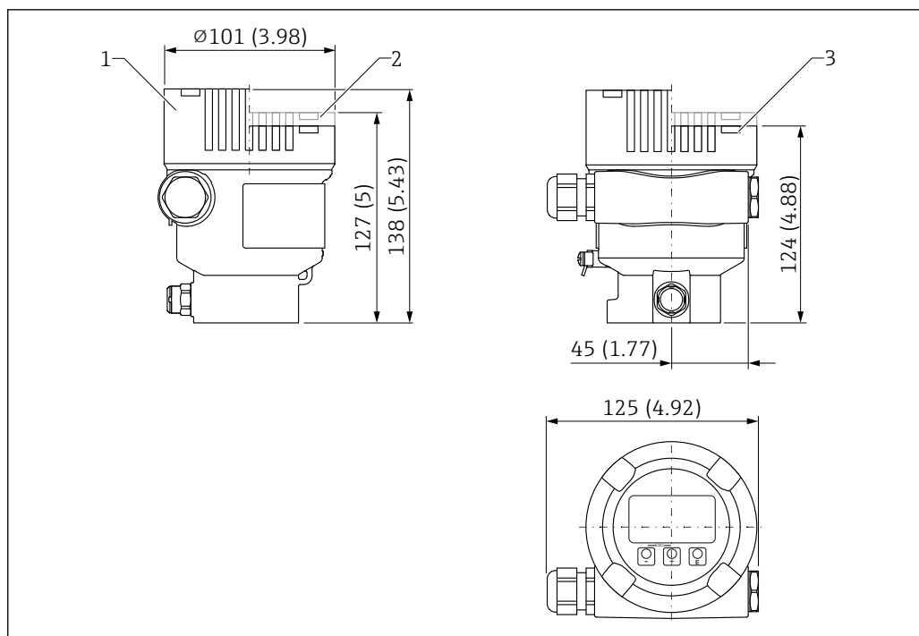
図 42 寸法 ; シングルコンパートメントハウジング (アルミニウム、コーティング) ; M20 カップリングおよびプラグ (プラスチック) 付き。測定単位 mm (in)
