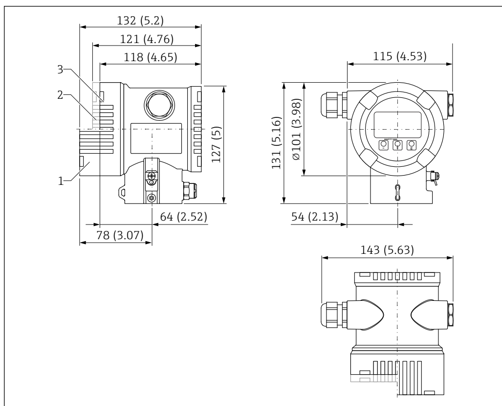
図 44 寸法；デュアルコンパートメントハウジング（アルミニウム、コーティング）；M20 カップリングおよびプラグ（プラスチック）付き。測定単位 mm (in)
