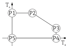
図 18 プラスチックハウジング ; プロセス温度 0~+130 °C (+32~+266 °F)、CSA C/US 認定取得
