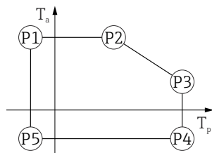
図 29 SUS 316L 相当製ハウジング ; プロセス温度 -20\sim+150\text{ }^{\circ}\text{C} ( -4\sim+302\text{ }^{\circ}\text{F} )
