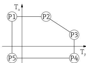
☑ 38 SUS 316L 相当製ハウジング、サニタリ仕様；プロセス温度 -40\sim+130\text{ }^{\circ}\text{C} ( -40\sim+266\text{ }^{\circ}\text{F} )
