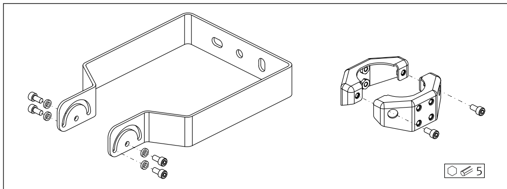
図 70 納入範囲；調整可能な取付ブラケット FMR6xB
