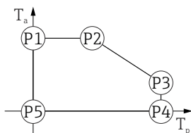
図 14 プラスチックハウジング ; プロセス温度 0\sim+200\text{ }^{\circ}\text{C} ( +32\sim+392\text{ }^{\circ}\text{F} )、CSA C/US 認定取得
