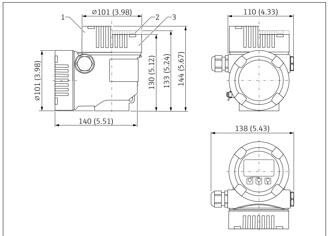
図 46 寸法；デュアルコンパートメントハウジングL字型 (SUS 316 L 相当)；M20 カップリングおよびプラグ (プラスチック) 付き。測定単位 mm (in)
