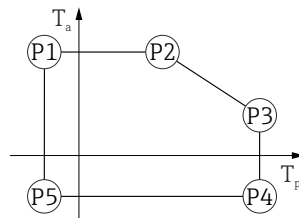
図 17 プラスチックハウジング ; プロセス温度 -40~+130 °C (-40~+266 °F)
