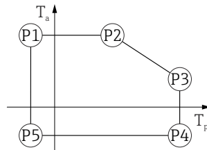
図 23 アルミニウムハウジング ; コーティング ; プロセス温度 -20~+150 °C (-4~+302 °F)
