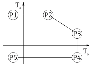
図 11 プラスチックハウジング ; プロセス温度 -20~+150 °C (-4~+302 °F)
