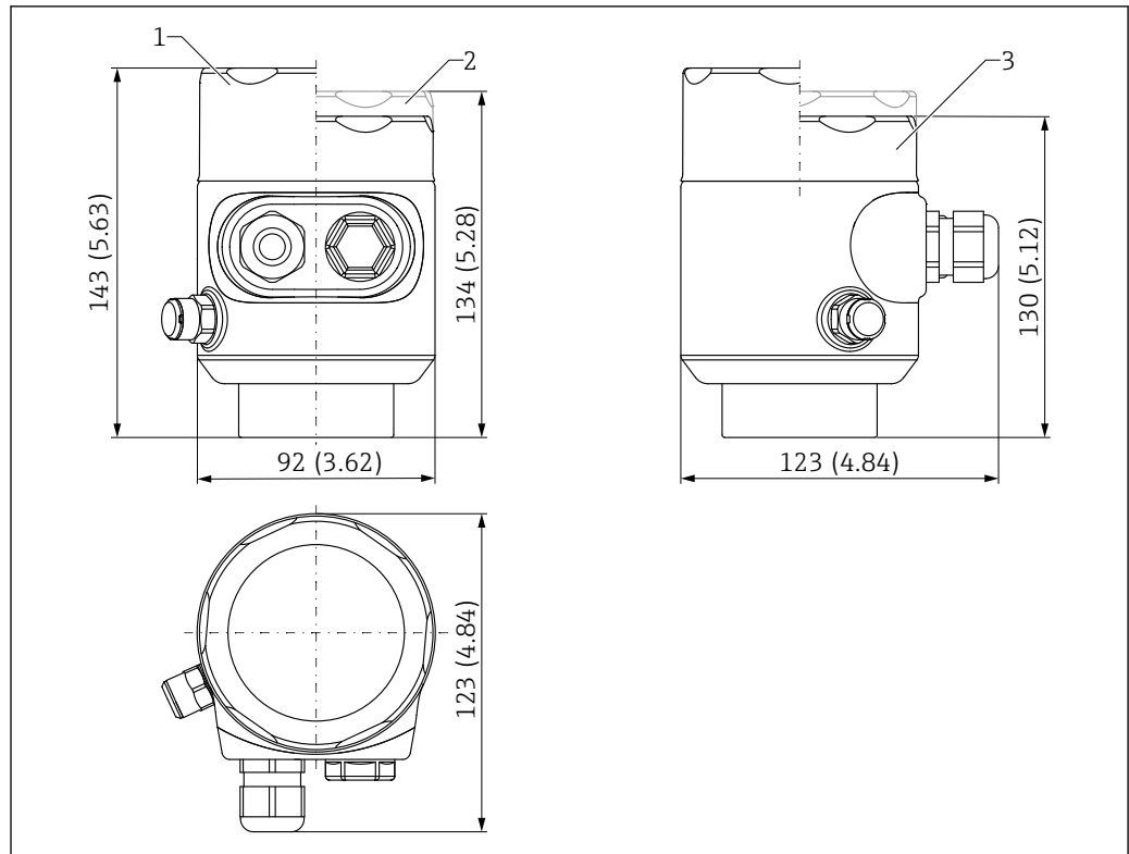
図 43 寸法 ; シングルコンパートメントハウジング (SUS 316L 相当、サニタリ仕様) ; M20 カップリング およびプラグ (プラスチック) 付き。測定単位 mm (in)
