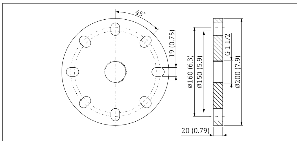
図 49 UNI フランジ 3"/DN80/80A の寸法。測定単位 mm (in)
