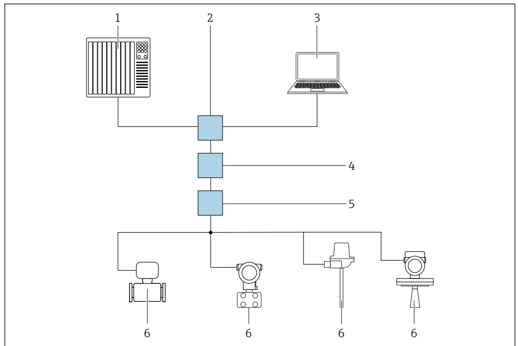
図 65 PROFINET (Ethernet-APL 対応) ネットワーク経由のリモート操作オプション：スター型トポロジ
