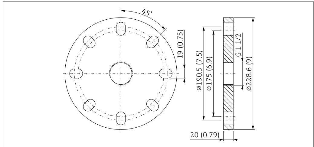
図 55 UNI フランジ 4"/DN100/100A の寸法。測定単位 mm (in)
