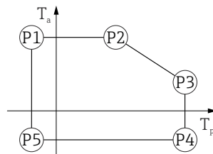
図 24 アルミニウムハウジング ; コーティング ; プロセス温度 -20~+200 °C (-4~+392 °F)
