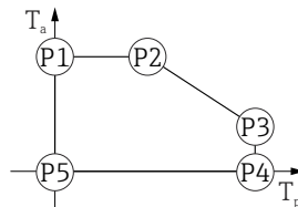
図 12 プラスチックハウジング ; プロセス温度 0~+150 °C (+32~+302 °F)、CSA C/US 認定取得
