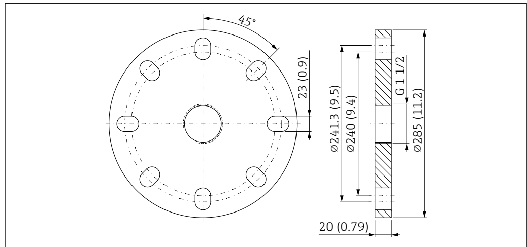
図 56 UNI フランジ 6"/DN150/150A の寸法。測定単位 mm (in)
