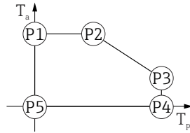
図 16 プラスチックハウジング ; プロセス温度 0~+80 °C (+32~+176 °F)、CSA C/US 認定取得
