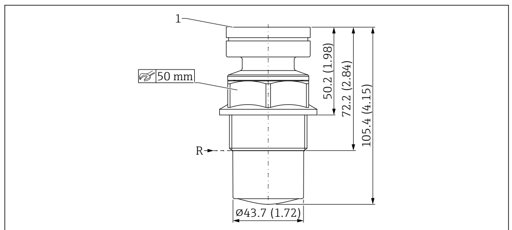
図 47 寸法；被覆アンテナ、PVDF、40 mm (1.5 in)。測定単位 mm (in)
