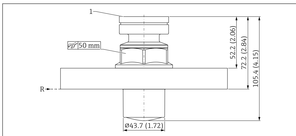
図 48 被覆アンテナ (PVDF、40 mm (1.5 in)、プロセス接続 UNI フランジ) の寸法。測定単位 mm (in)
