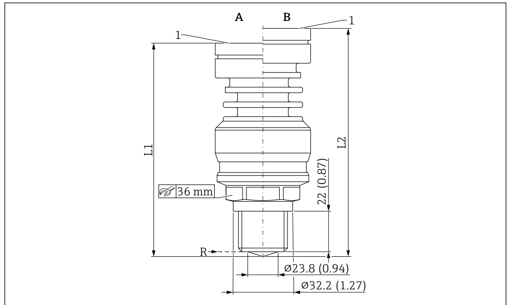
図 57 寸法；内蔵アンテナ、PEEK、20 mm (0.75 in)；プロセス接続、ネジ 3/4"。測定単位 mm (in)
