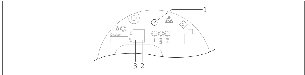
図 63 Ethernet-APL エレクトロニックインサート上の操作キーおよび DIP スイッチ
