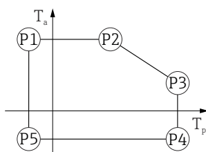
図 15 プラスチックハウジング ; プロセス温度 -40\sim+80\text{ }^{\circ}\text{C} ( -40\sim+176\text{ }^{\circ}\text{F} )
