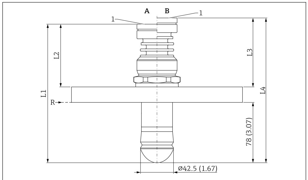
図 53 ドリップオフアンテナ 50 mm (2 in) (UNI フランジプロセス接続) の寸法。測定単位 mm (in)
