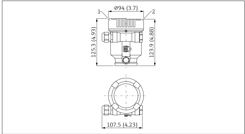
図 41 寸法 ; シングルコンパートメントハウジング (プラスチック) ; M20 カップリングおよびプラグ (プラスチック) 付き。測定単位 mm (in)
