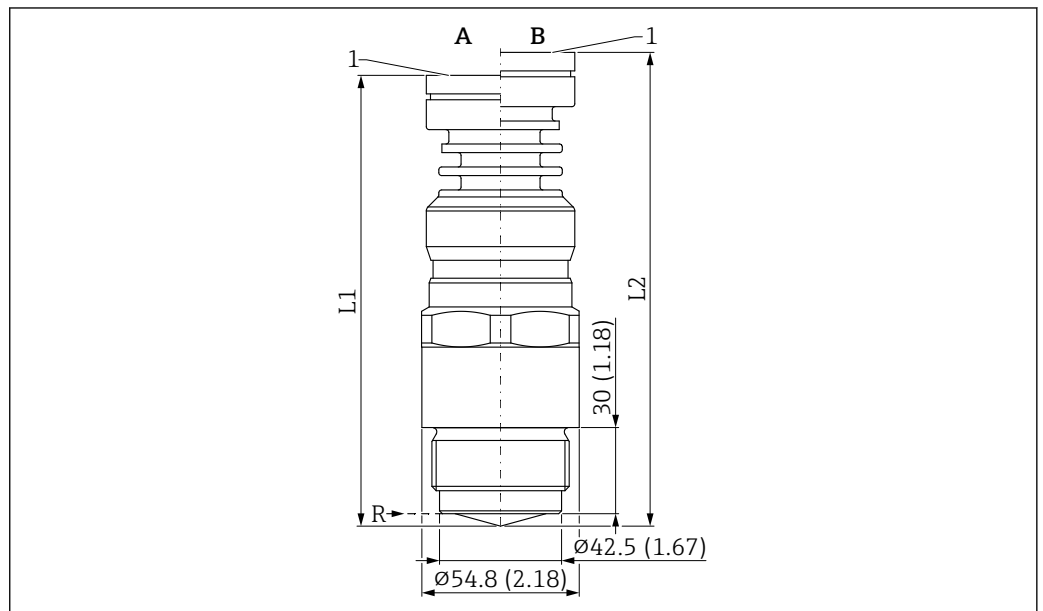
図 58 寸法；内蔵アンテナ、PEEK、40 mm (1.5 in)；プロセス接続、ネジ 1-1/2"。測定単位 mm (in)
