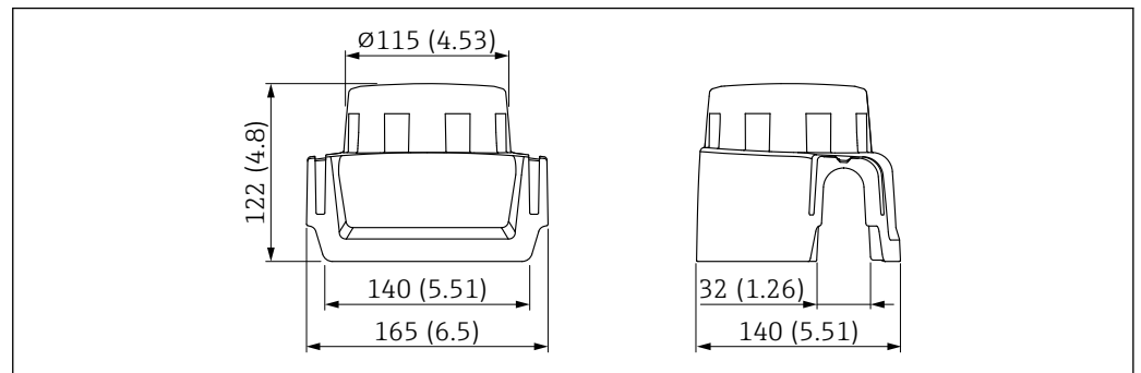
図 67 日除けカバー、プラスチック、XW111 の寸法。測定単位 mm (in)
