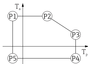
図 30 SUS 316L 相当製ハウジング ; プロセス温度 -20\sim+200\text{ }^{\circ}\text{C} ( -4\sim+392\text{ }^{\circ}\text{F} )
