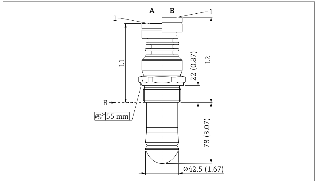
图 52 水滴型天线 (50 mm (2 in)口径) 的外形尺寸示意图, 螺纹过程连接
