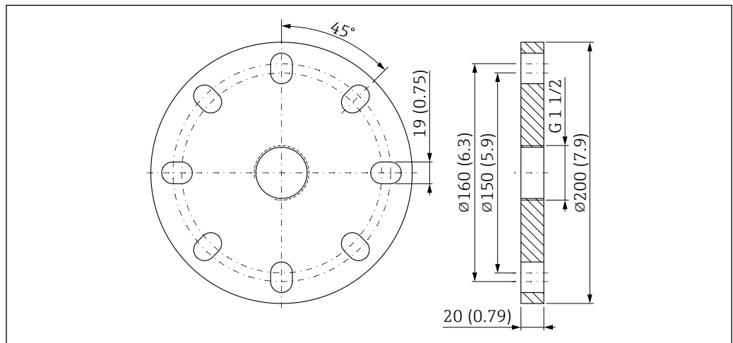
图 49 UNI 3"/DN80/80A 法兰的外形尺寸示意图。测量单位 mm (in)
