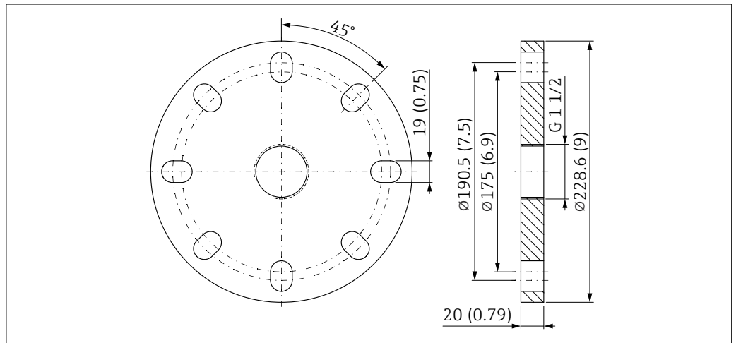
图 50 UNI 4"/DN100/100A 法兰的外形尺寸示意图。测量单位 mm (in)
