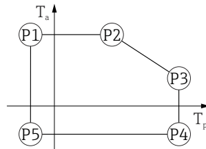
15 塑料外壳; 过程温度范围: -40 ... +80 °C (-40 ... +176 °F)
