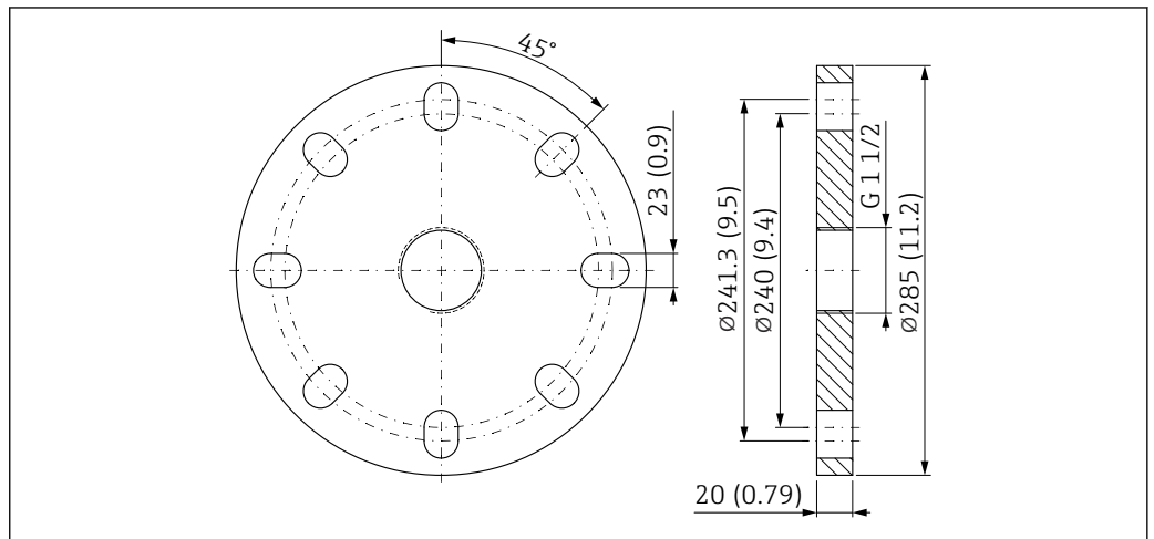
图 51 UNI 6"/DN150/150A 法兰的外形尺寸示意图。测量单位 mm (in)
