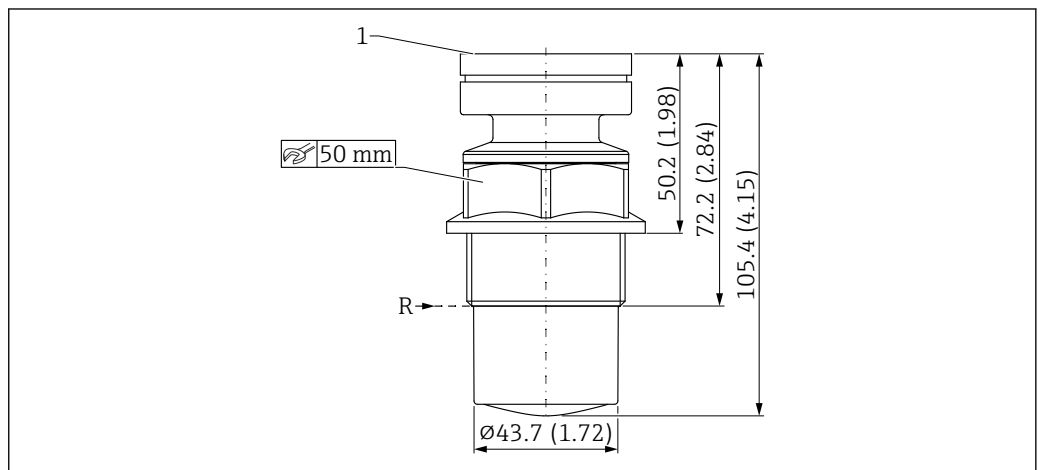
图 47 PVDF 全密封天线 (40 mm (1.5 in) 口径) 的外形尺寸示意图。测量单位 mm (in)
