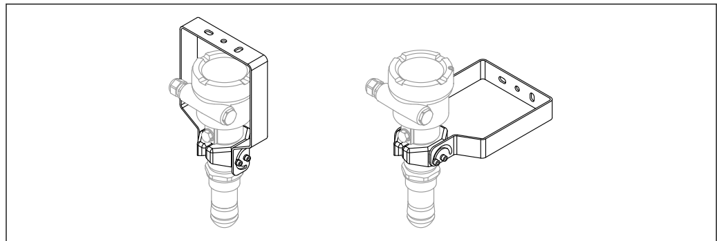
图 68 FMR6xB 的安装架 (可调节)；安装在罐顶或墙壁上
