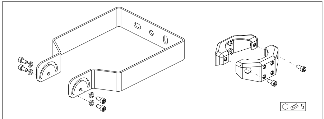
图 70 供货清单; FMR6xB 的安装架 (可调节)
