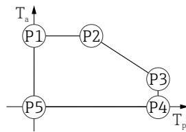
16 塑料外壳; 过程温度范围: 0 ... +80 °C (+32 ... +176 °F), 适用 CSA C/US 认证型仪表
