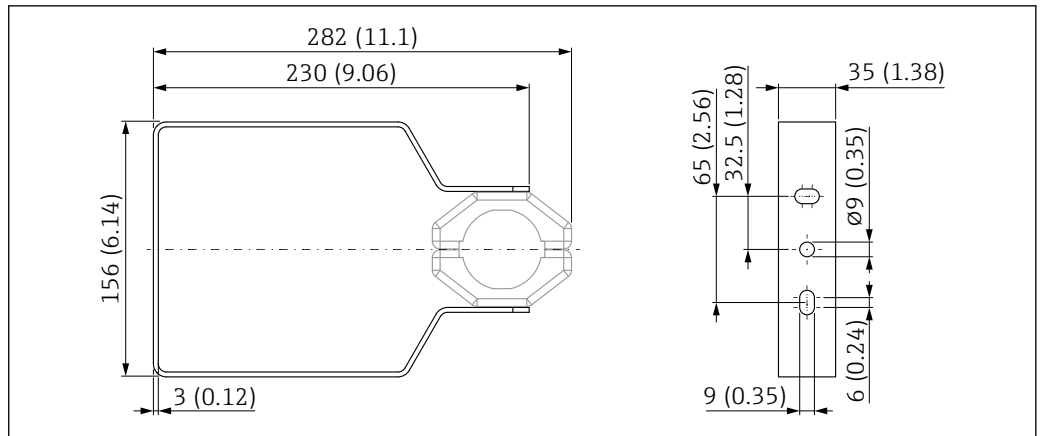
图 69 外形尺寸示意图; FMR6xB 的安装架 (可调节)。测量单位 mm (in)
