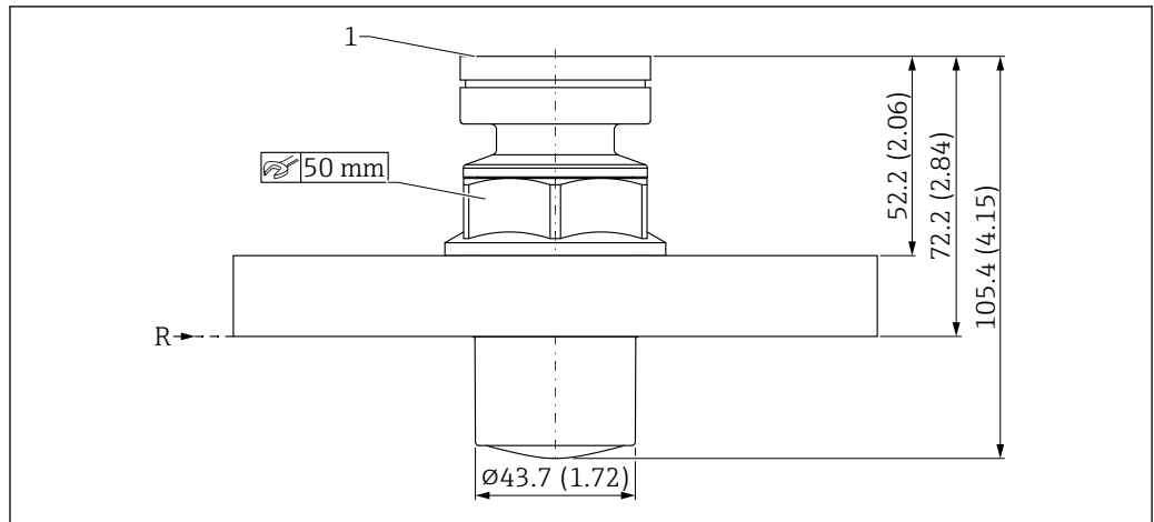
图 48 PVDF 全密封天线 (40 mm (1.5 in) 口径) 的外形尺寸示意图；UNI 法兰过程连接。测量单位 mm (in)
