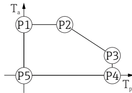
☑ 12 塑料外壳; 过程温度范围: 0 \dots +150 \text{ }^\circ\text{C} ( +32 \dots +302 \text{ }^\circ\text{F} ), 适用 CSA C/US 认证型仪表
