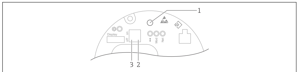
图 63 Ethernet-APL 电子插件上的操作按键和 DIP 开关
