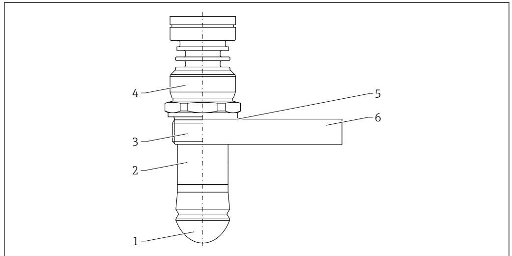
☑ 60 水滴型天线 (50 mm (2 in)口径) 的材质
