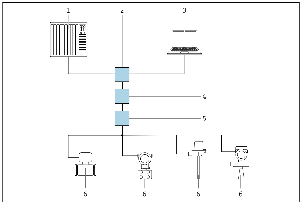
图 65 通过 PROFINET + Ethernet-APL 网络实现远程操作: 星形拓扑结构
