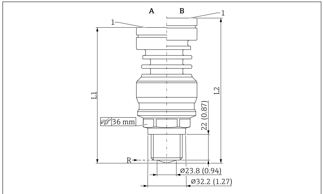
57 PEEK 一体式天线 (20 mm (0.75 in) 口径) 的外形尺寸示意图; 3/4"螺纹过程连接。测量单位 mm (in)
