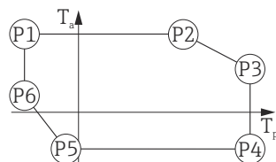
図 52 SUS 316L 相当製ハウジング、サニタリ仕様；プロセス温度 -196\sim+200\text{ }^{\circ}\text{C} ( -320\sim+392\text{ }^{\circ}\text{F} )
