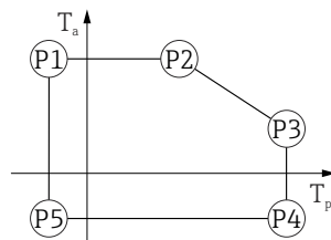
☐ 41 SUS 316L 相当製ハウジング ; プロセス温度範囲 : -40\sim+150\text{ }^{\circ}\text{C} ( -40\sim+302\text{ }^{\circ}\text{F} )
