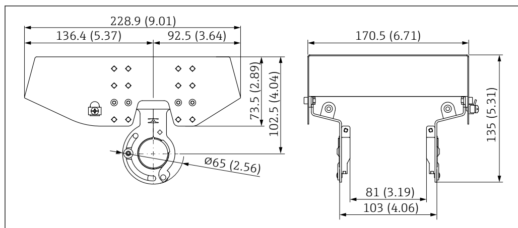
図 70 日除けカバー、SUS 316L 相当、XW112 の寸法。測定単位 mm (in)
