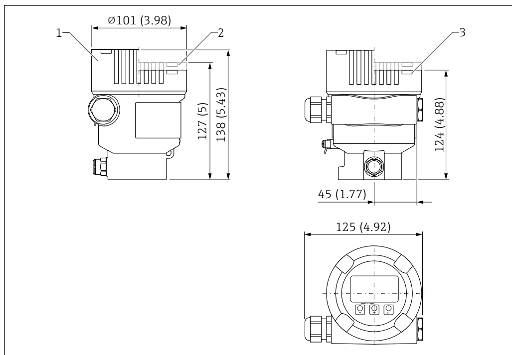
図 54 寸法 ; シングルコンパートメントハウジング (アルミニウム、コーティング) ; M20 カップリングおよびプラグ (プラスチック) 付き。測定単位 mm (in)
