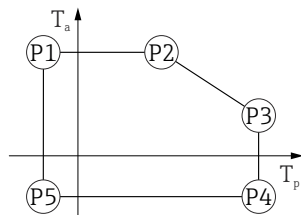
図 15 プラスチックハウジング ; プロセス温度 -20\sim+150\text{ }^{\circ}\text{C} ( -4\sim+302\text{ }^{\circ}\text{F} )
