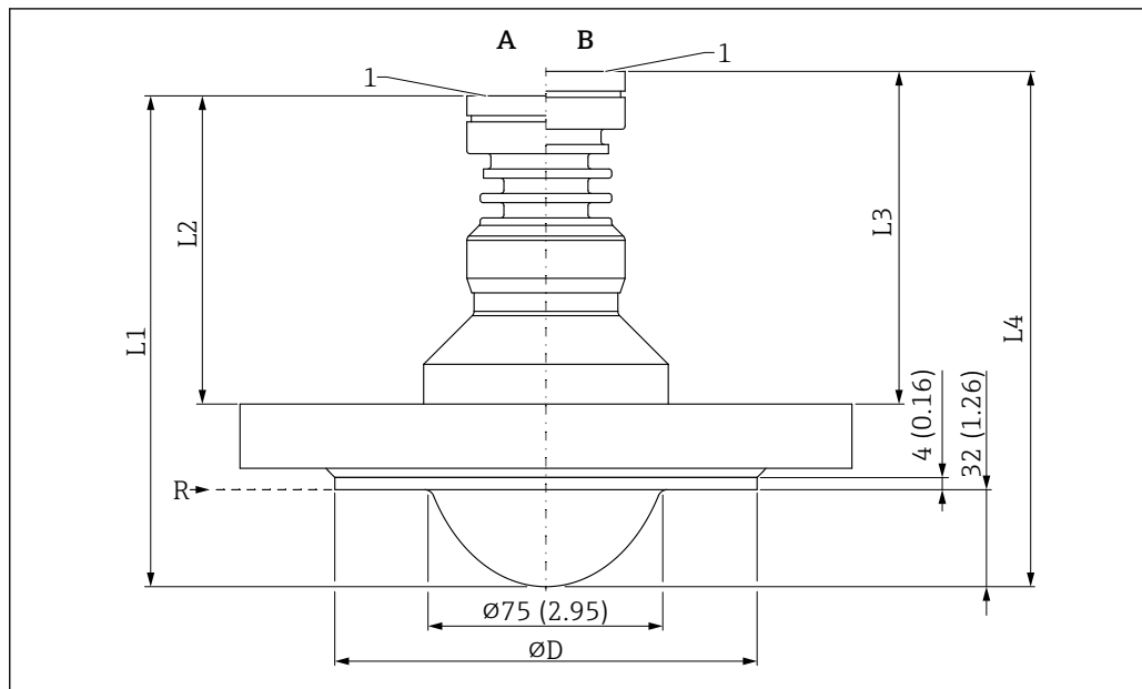
図 62 PTFE 外装付フラッシュマウントアンテナ (80 mm (3 in)、フランジ付き) の寸法。測定単位 mm (in)
