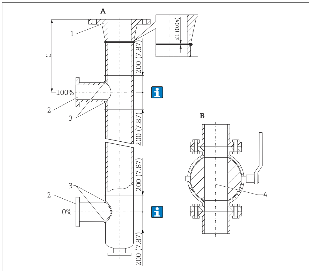
図 14 外筒管の構造例。測定単位 mm (in)
