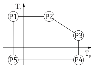
図 31 アルミニウムハウジング ; コーティング ; プロセス温度 -20~+150 °C (-4~+302 °F)
