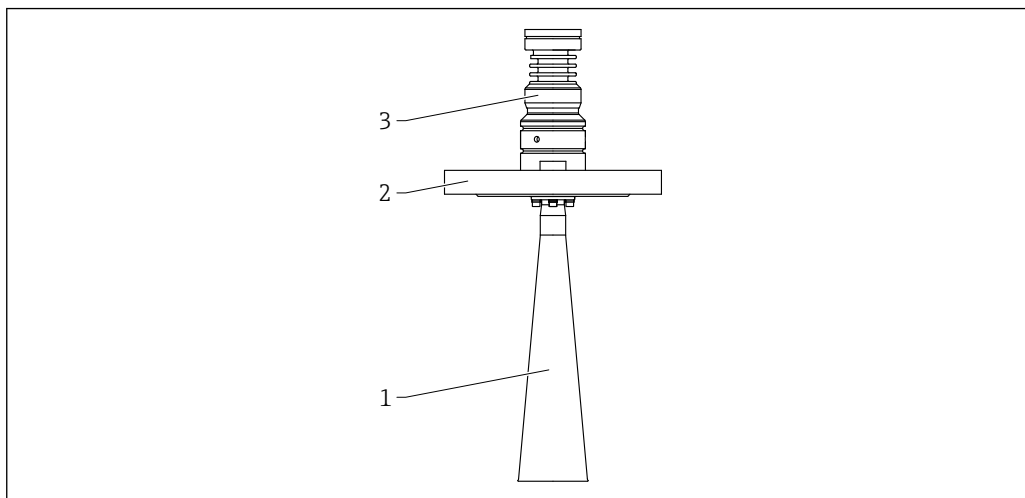
図 63 材質 ; DN65 ホーンアンテナ。測定単位 mm (in)
