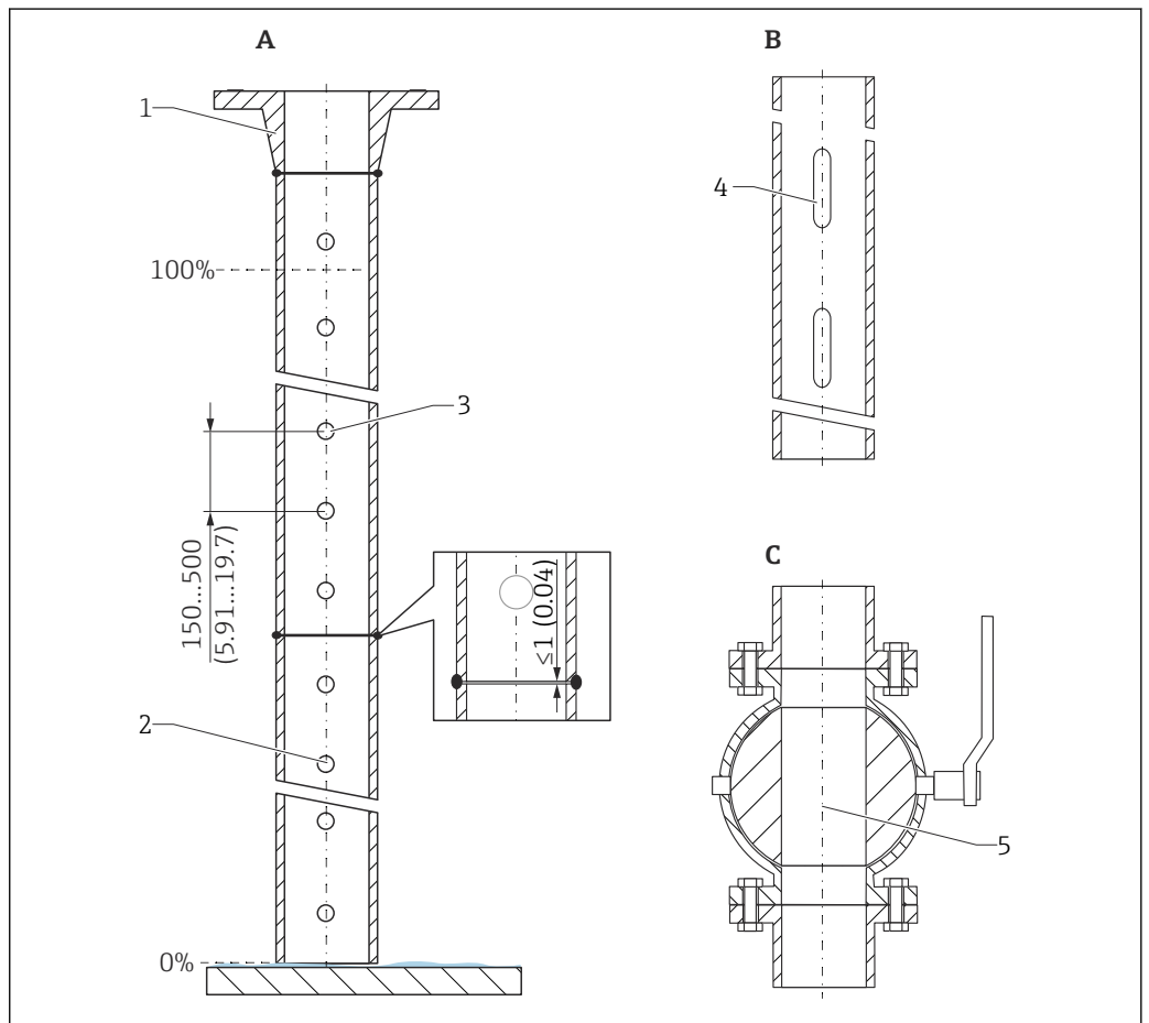
図 12 内筒管の構造例。測定単位 mm (in)
