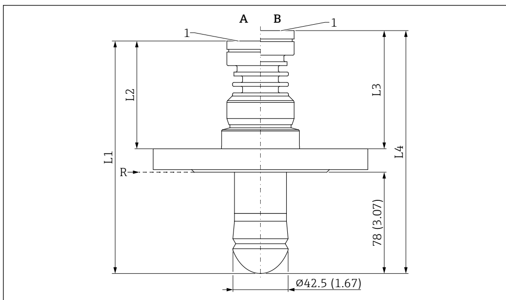
図 60 フランジプロセス接続の寸法。測定単位 mm (in)
