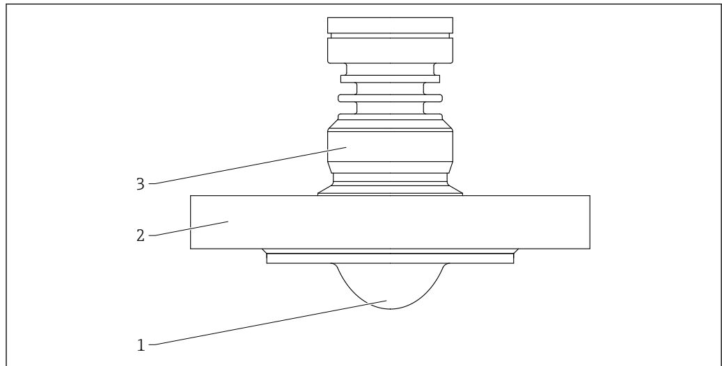
図 65 材質 ; PTFE 外装付フラッシュマウントアンテナ、50 mm (2 in)、フランジ付き
