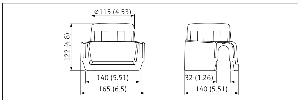
図 71 日除けカバー、プラスチック、XW111 の寸法。測定単位 mm (in)
