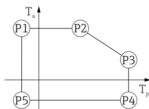
図 19 プラスチックハウジング ; プロセス温度 -40~+150 °C (-40~+302 °F)
