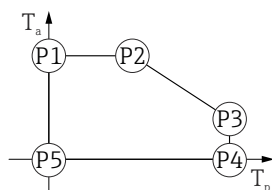
図 26 プラスチックハウジング ; プロセス温度 0~+450 °C (+32~+842 °F)、CSA C/US 認定取得
