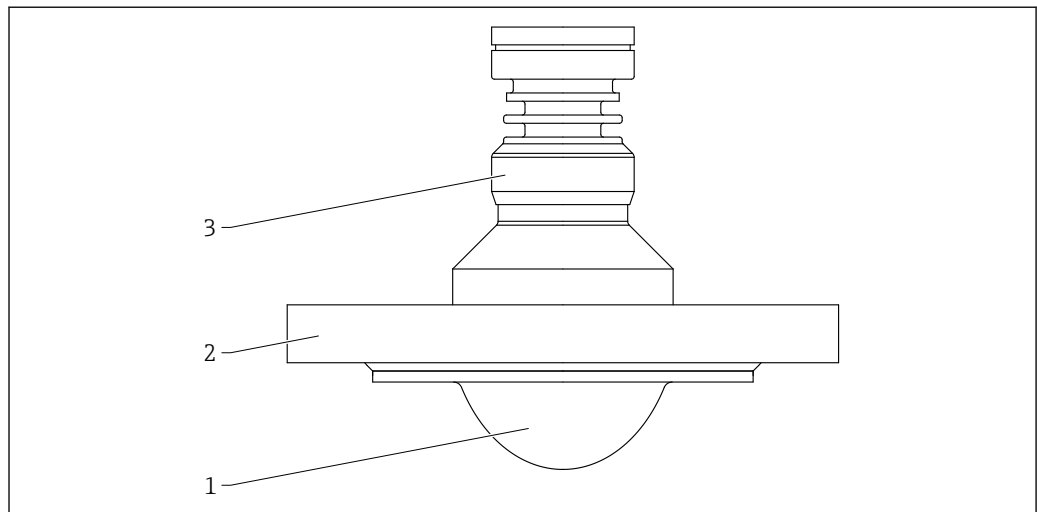
図 66 材質 ; PTFE 外装付フラッシュマウントアンテナ、80 mm (3 in)、フランジ付き
