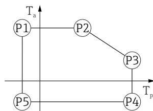
図 32 アルミニウムハウジング ; コーティング ; プロセス温度 -20~+200 °C (-4~+392 °F)
