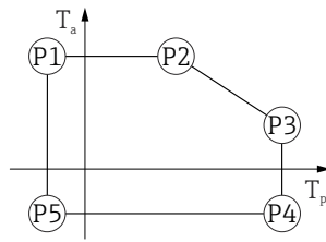
図 27 プラスチックハウジング ; プロセス温度 -60\sim+150\text{ }^{\circ}\text{C} ( -76\sim+302\text{ }^{\circ}\text{F} )
