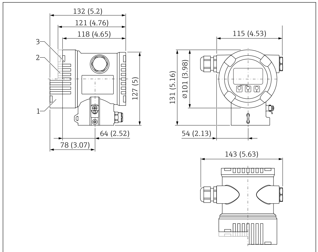
図 56 寸法；デュアルコンパートメントハウジング（アルミニウム、コーティング）；M20 カップリングおよびプラグ（プラスチック）付き。測定単位 mm (in)
