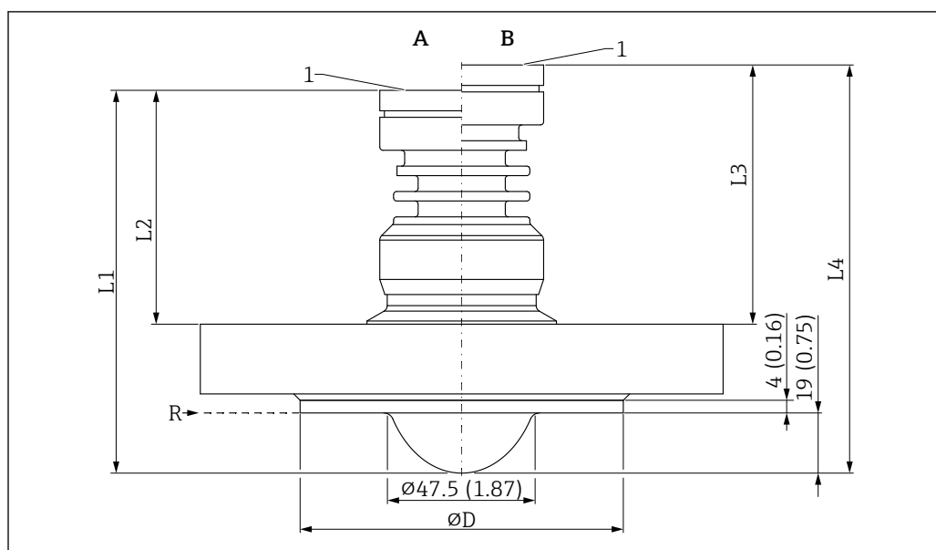
図 61 PTFE 外装付フラッシュマウントアンテナ (50 mm (2 in)、フランジ付き) の寸法。測定単位 mm (in)
