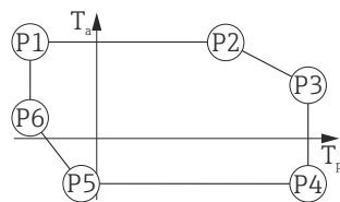
☐ 46 SUS 316L 相当製ハウジング ; プロセス温度 -196~+200 °C (-320~+392 °F)
