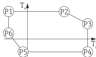
図 29 プラスチックハウジング ; プロセス温度 -196\sim+200\text{ }^{\circ}\text{C} ( -320\sim+392\text{ }^{\circ}\text{F} )
