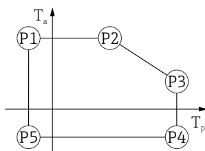
☑ 50 SUS 316L 相当製ハウジング、サニタリ仕様；プロセス温度 -40\sim+200\text{ }^{\circ}\text{C} ( -40\sim+392\text{ }^{\circ}\text{F} )
