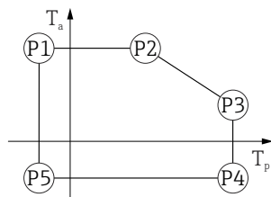
図 51 SUS 316L 相当製ハウジング、サニタリ仕様；プロセス温度 -60\sim+150\text{ }^{\circ}\text{C} ( -76\sim+302\text{ }^{\circ}\text{F} )
