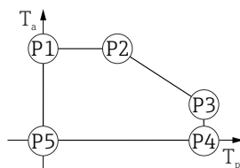
図 16 プラスチックハウジング ; プロセス温度 0\sim+150\text{ }^{\circ}\text{C} ( +32\sim+302\text{ }^{\circ}\text{F} )、CSA C/US 認定取得
