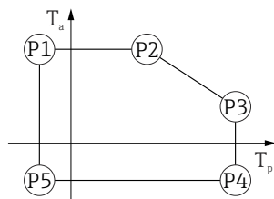
☐ 47 SUS 316L 相当製ハウジング、サニタリ仕様 ; プロセス温度 -20~+150 °C (-4~+302 °F)
