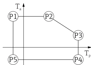
図 17 プラスチックハウジング ; プロセス温度 -20\sim+200\text{ }^{\circ}\text{C} ( -4\sim+392\text{ }^{\circ}\text{F} )
