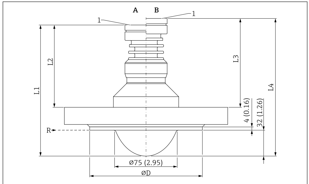
图 62 PTFE 涂层天线（齐平安装，80 mm (3 in)口径）的外形尺寸示意图；带法兰。测量单位 mm (in)
