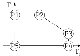
28 塑料外壳; 过程温度: 0 \dots +150 \text{ }^\circ\text{C} ( +32 \dots +302 \text{ }^\circ\text{F} ), 针对 CSA C/US 认证型仪表
