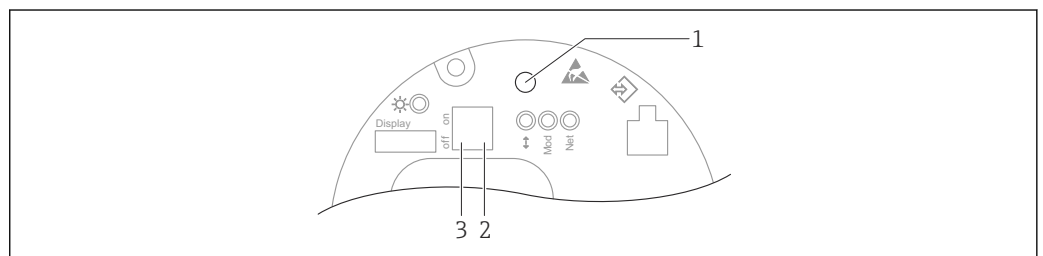
图 67 Ethernet-APL 电子插件上的操作按键和 DIP 开关
