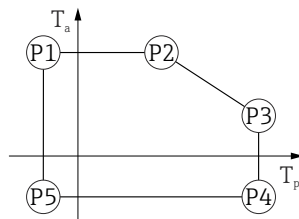
图 35 铝外壳, 带涂层; 过程温度: -40 \dots +280 \text{ }^\circ\text{C} ( -40 \dots +536 \text{ }^\circ\text{F} )
