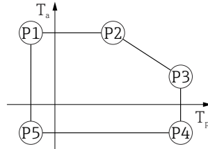
15 塑料外壳; 过程温度范围: -20 \dots +150 \text{ }^\circ\text{C} ( -4 \dots +302 \text{ }^\circ\text{F} )
