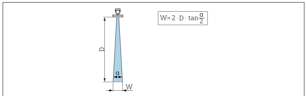
9 波束角 \alpha 、距离 D 和波束宽度 W 的相互关系
