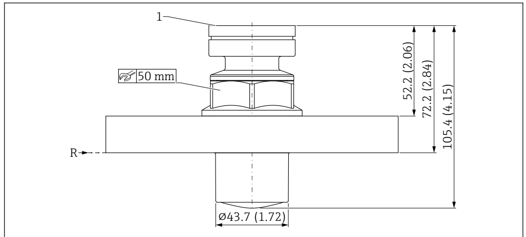
图 27 PVDF 全密封天线 (40 mm (1.5 in)口径) 的外形尺寸示意图; UNI 法兰过程连接。测量单位 mm (in)
