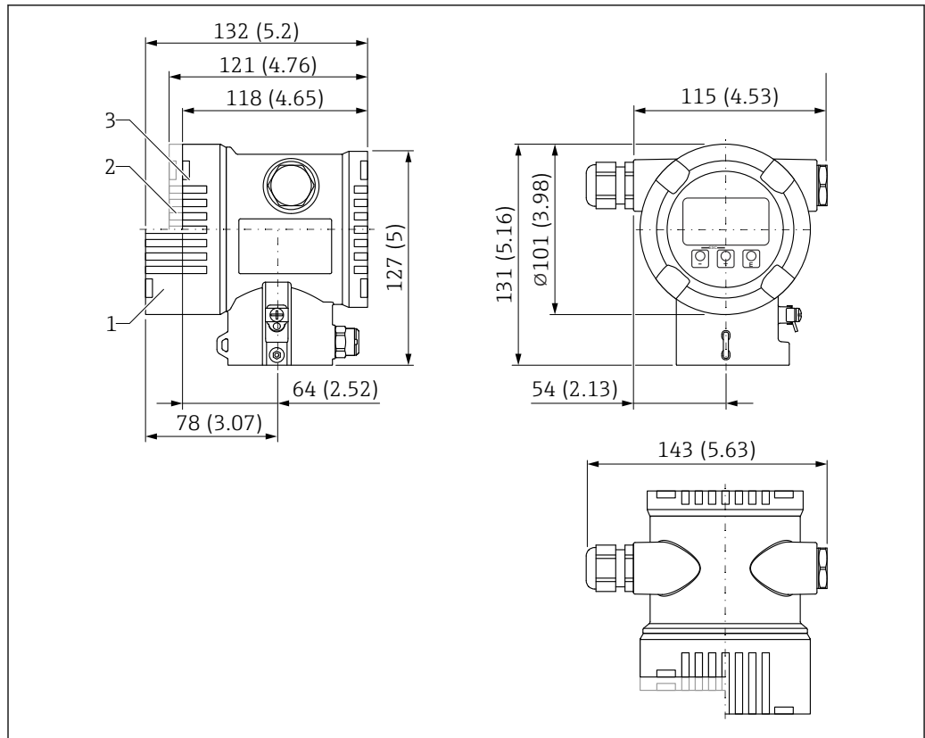
图 23 双腔室铝外壳 (带涂层) 的外形尺寸示意图; 包括 M20 接头和塑料插头。测量单位 mm (in)
