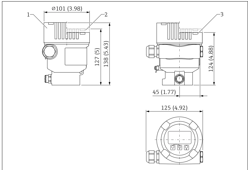
图 21 单腔室铝外壳 (带涂层) 的外形尺寸示意图; 包括 M20 接头和塑料插头。测量单位 mm (in)
