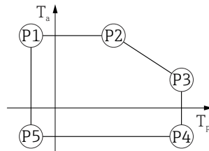
图 14 铝外壳, 带涂层; 过程温度范围: -40 ... +80 °C (-40 ... +176 °F)
