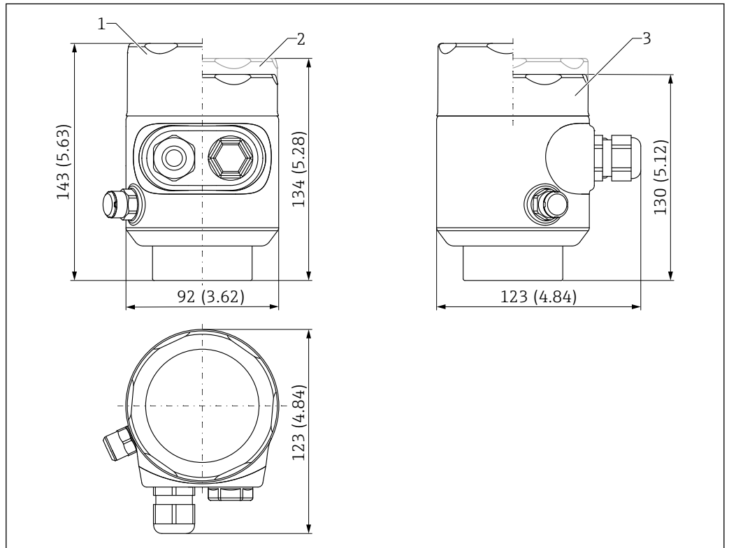
图 22 316L 单腔室外壳 (卫生型) 的外形尺寸示意图; 包括 M20 接头和塑料插头。测量单位 mm (in)
