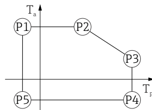
图 15 铝外壳, 带涂层; 过程温度范围: -40 ... +130 °C (-40 ... +266 °F)
