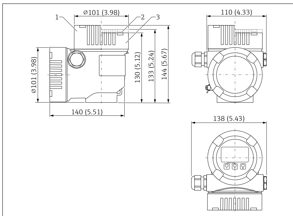
図 25 寸法；デュアルコンパートメントハウジング L 字型 (SUS 316 L 相当)；M20 カップリングおよびプラグ (プラスチック) 付き。測定単位 mm (in)
