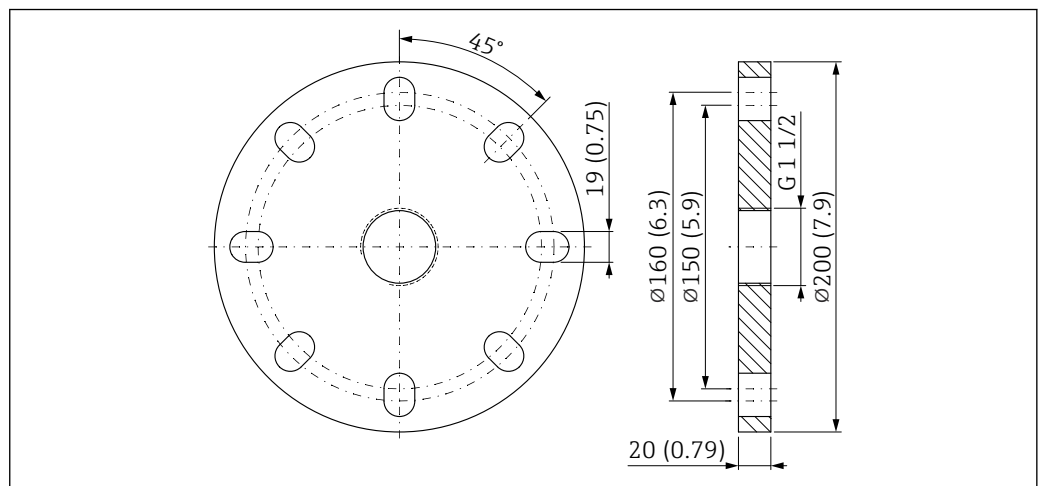
図 28 UNI フランジ 3"/DN80/80A の寸法。測定単位 mm (in)
