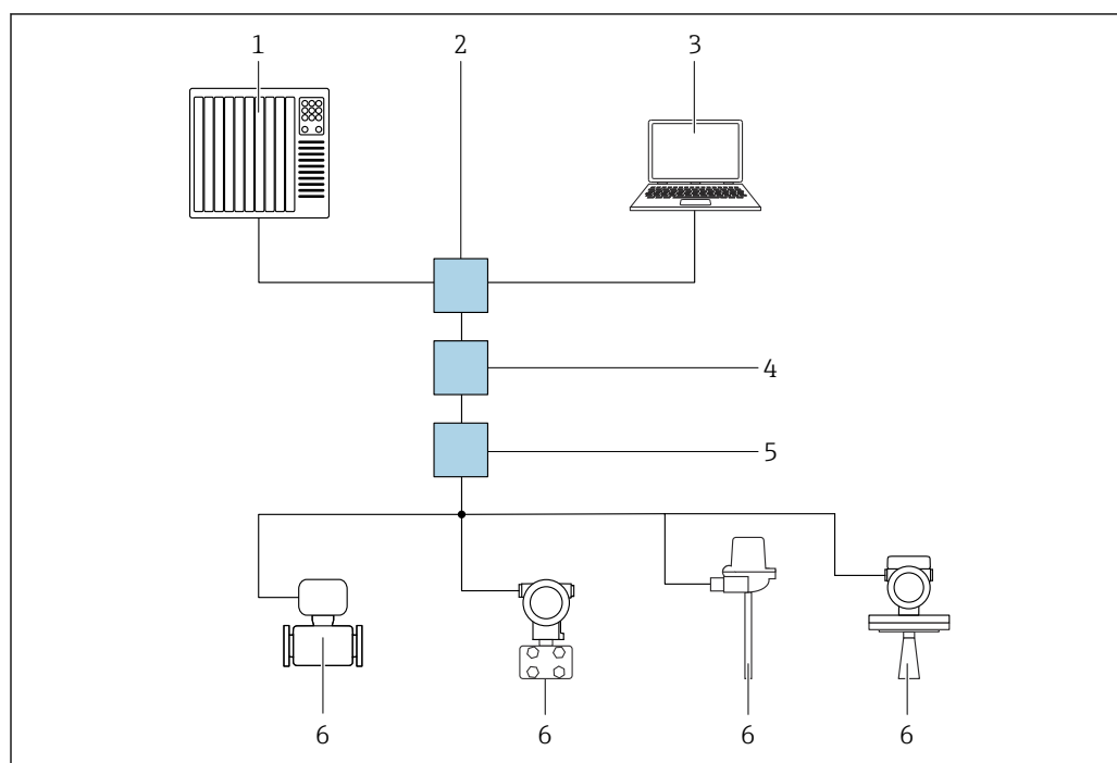
図 40 PROFINET (Ethernet-APL 対応) ネットワーク経由のリモート操作オプション：スター型トポロジ
