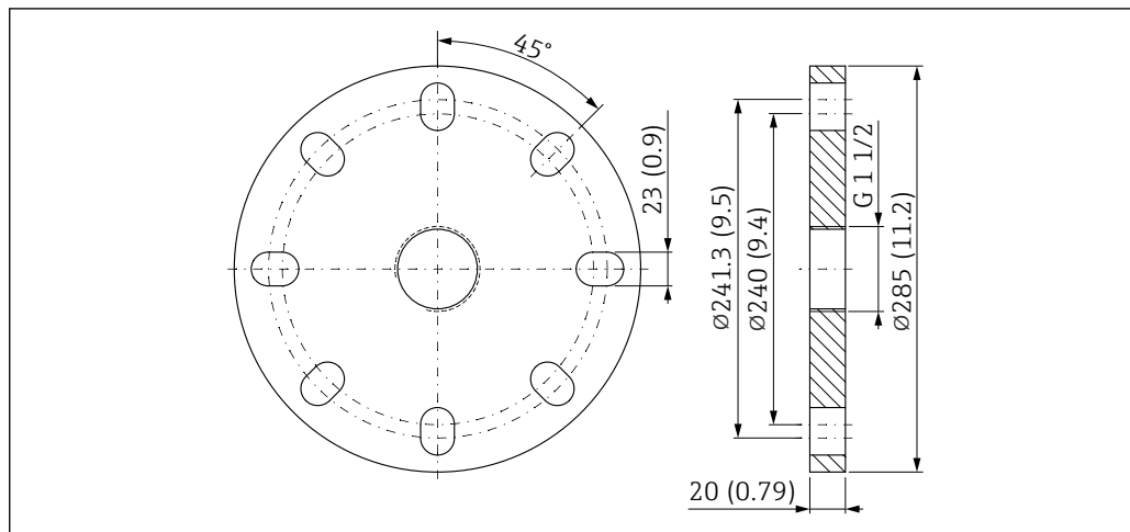
図 35 UNI フランジ 6"/DN150/150A の寸法。測定単位 mm (in)
