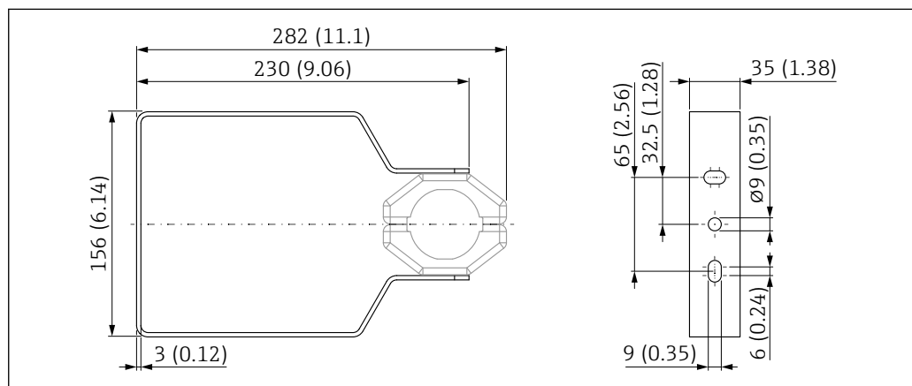
図 44 寸法 ; 調整可能な取付ブラケット FMR6xB。測定単位 mm (in)
