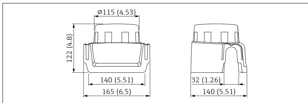
図 42 日除けカバー、プラスチック、XW111 の寸法。測定単位 mm (in)
