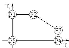
図 11 プラスチックハウジング ; プロセス温度 0\sim+80\text{ }^{\circ}\text{C} ( +32\sim+176\text{ }^{\circ}\text{F} )、CSA C/US 認定取得
