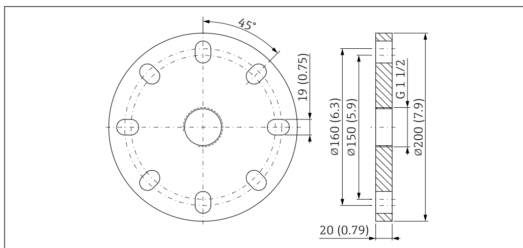
図 33 UNI フランジ 3"/DN80/80A の寸法。測定単位 mm (in)
