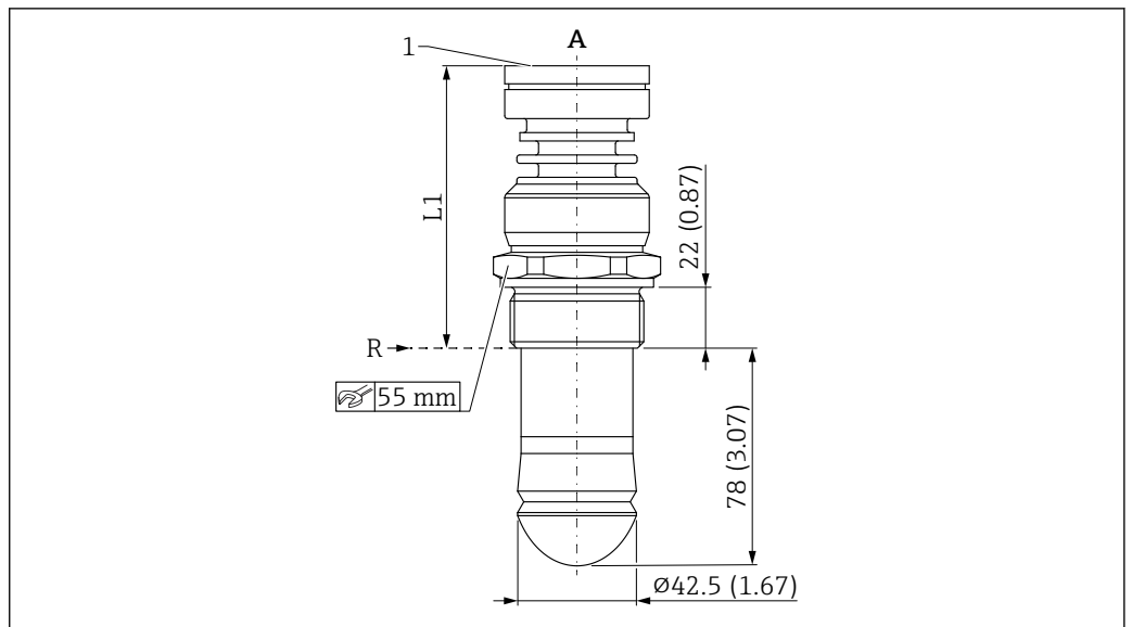
図 31 ドリップオフアンテナ 50 mm (2 in)、ネジ込みプロセス接続の寸法
