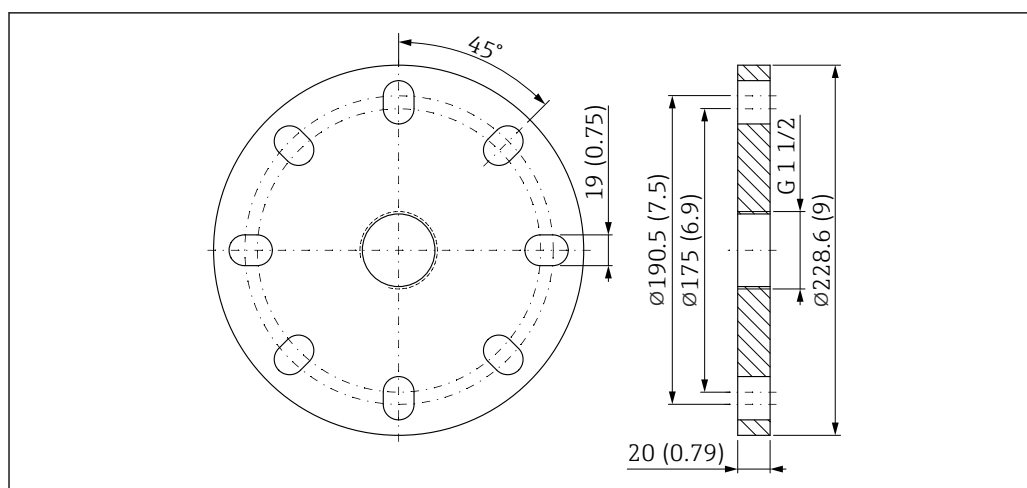
図 29 UNI フランジ 4"/DN100/100A の寸法。測定単位 mm (in)
