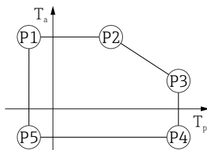
図 17 SUS 316L 相当製ハウジング ; プロセス温度 -40\sim+130\text{ }^{\circ}\text{C} ( -40\sim+266\text{ }^{\circ}\text{F} )
