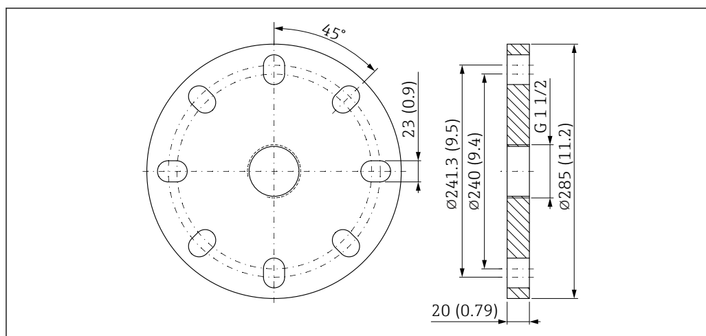
図 30 UNI フランジ 6"/DN150/150A の寸法。測定単位 mm (in)
