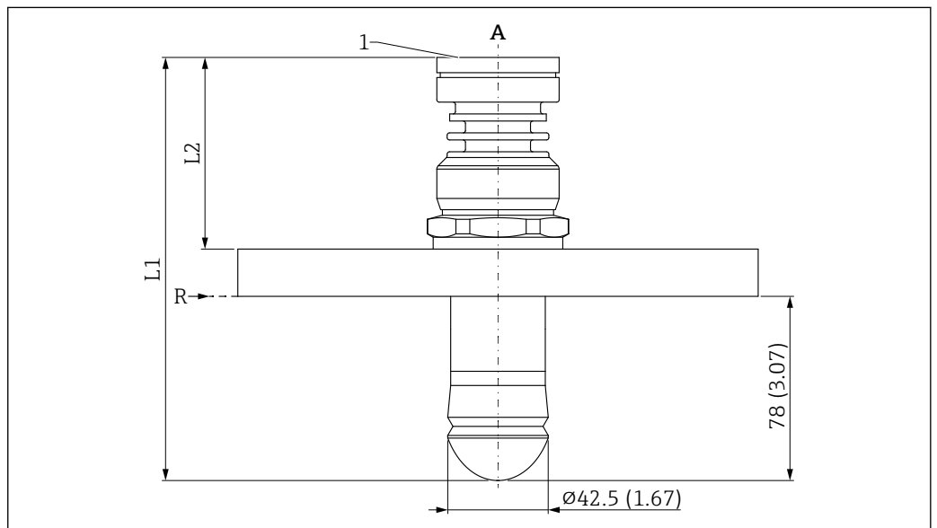
図 32 ドリップオフアンテナ 50 mm (2 in) (UNI フランジプロセス接続) の寸法。測定単位 mm (in)
