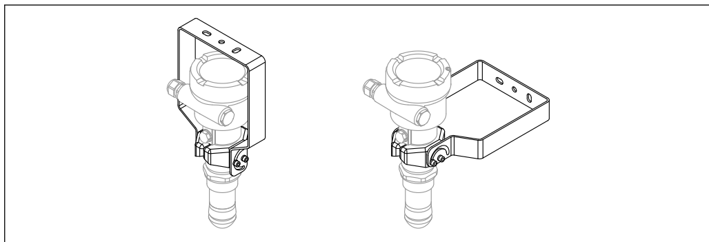
図 43 調整可能な取付ブラケット FMR6xB ; 天井または壁面取付け
