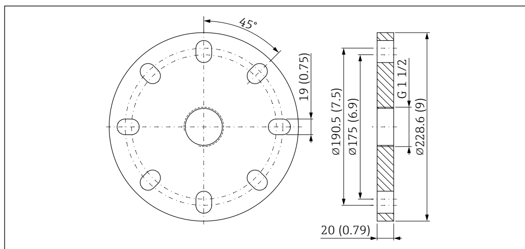
図 34 UNI フランジ 4"/DN100/100A の寸法。測定単位 mm (in)
