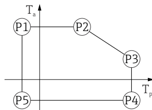
図 14 アルミニウムハウジング ; コーティング ; プロセス温度 -40~+80 °C (-40~+176 °F)
