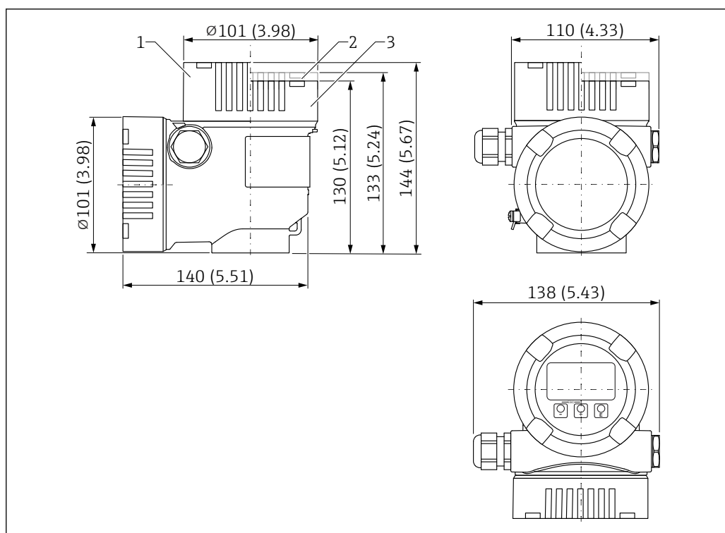
■ 24 寸法；デュアルコンパートメントハウジングL字型（アルミニウム、コーティング）；M20 カップリングおよびプラグ（プラスチック）付き。測定単位 mm (in)
