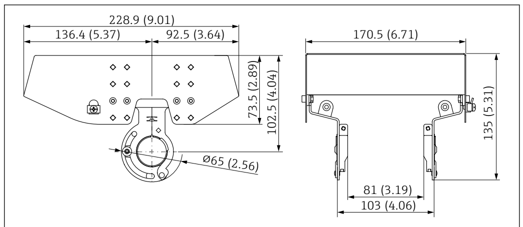
41 日除けカバー、SUS 316L 相当、XW112 の寸法。測定単位 mm (in)
