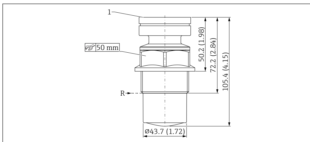
図 26 寸法；被覆アンテナ、PVDF、40 mm (1.5 in)。測定単位 mm (in)
