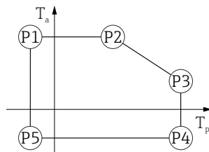
図 15 アルミニウムハウジング ; コーティング ; プロセス温度 -40~+130 °C (-40~+266 °F)
