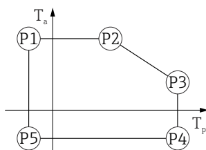
図 18 SUS 316L 相当製ハウジング、サニタリ仕様 ; プロセス温度 -40\sim+80\text{ }^{\circ}\text{C} ( -40\sim+176\text{ }^{\circ}\text{F} )
