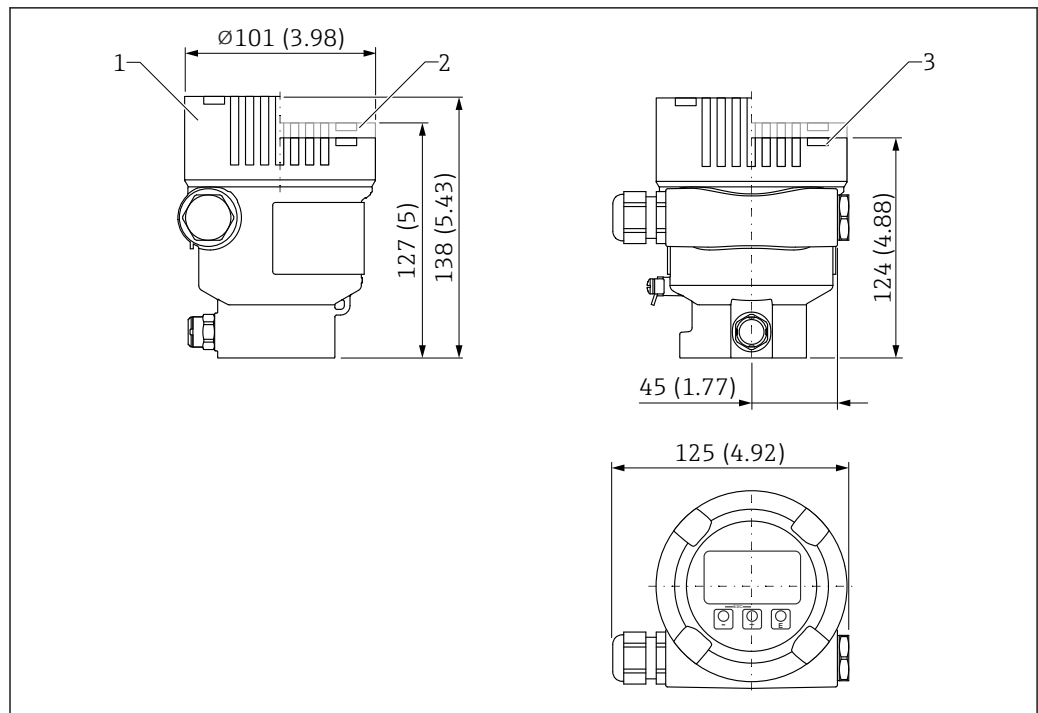
図 21 寸法 ; シングルコンパートメントハウジング (アルミニウム、コーティング) ; M20 カップリングおよびプラグ (プラスチック) 付き。測定単位 mm (in)
