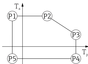
図 16 SUS 316L 相当製ハウジング ; プロセス温度 -40\sim+80\text{ }^{\circ}\text{C} ( -40\sim+176\text{ }^{\circ}\text{F} )
