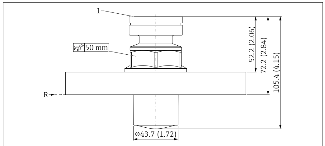
図 27 被覆アンテナ (PVDF、40 mm (1.5 in)、プロセス接続 UNI フランジ) の寸法。測定単位 mm (in)
