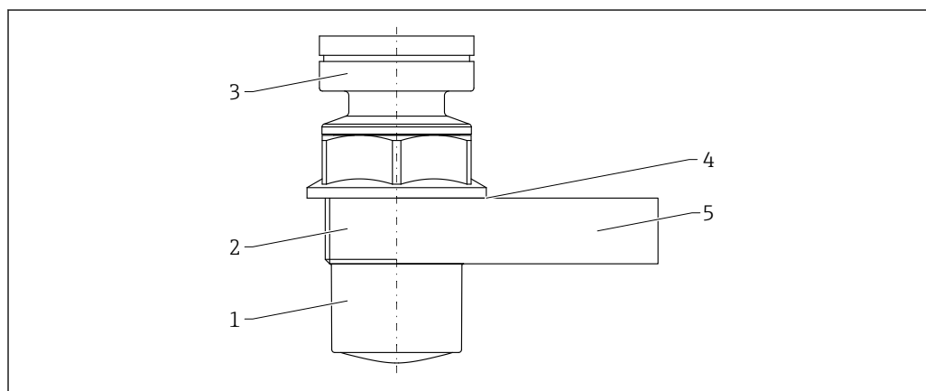
図 36 材質 ; 被覆アンテナ PVDF、40 mm (1.5 in)
