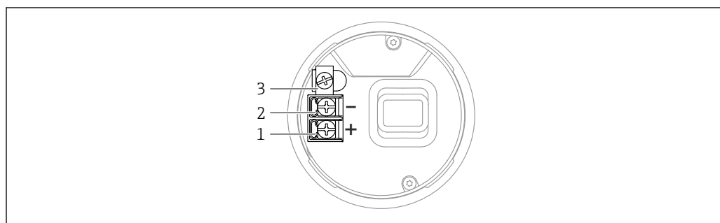
図 3 端子部の接続端子と接地端子（シングルコンパートメントハウジング）
