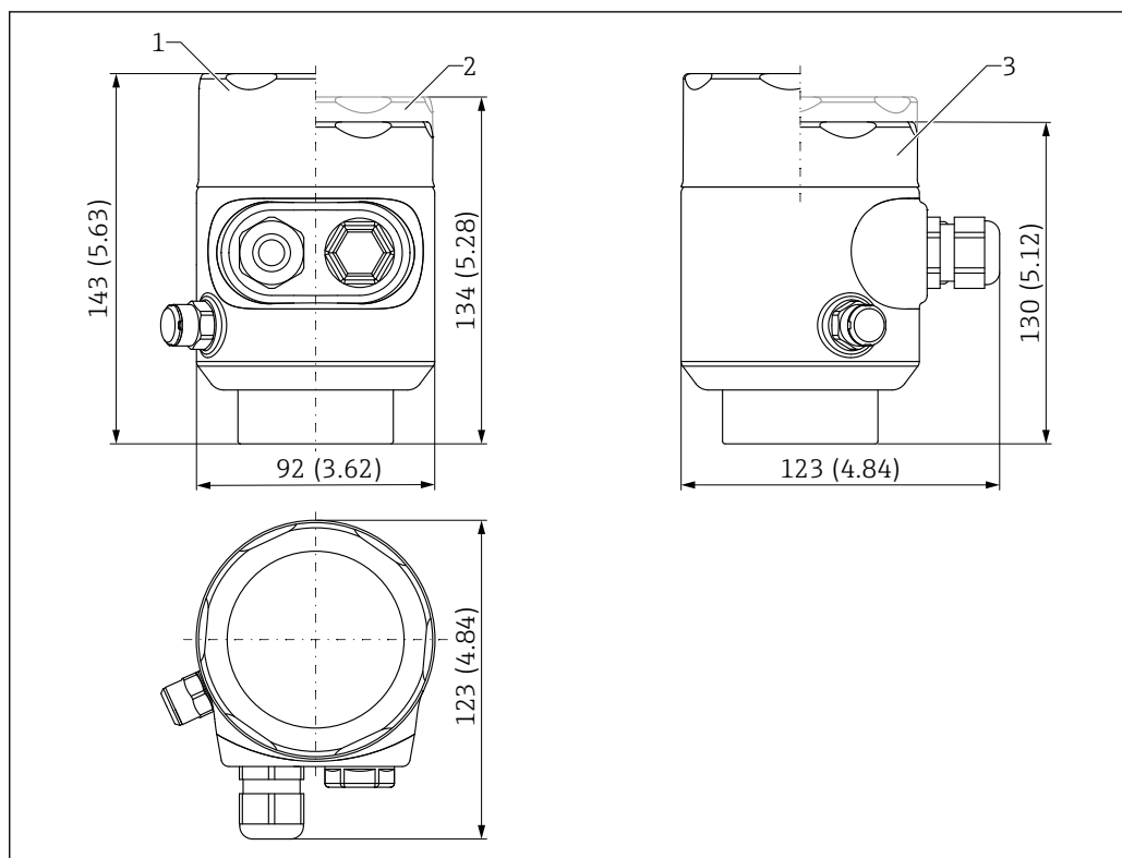
■ 21 寸法；シングルコンパートメントハウジング（SUS 316L 相当、サニタリ仕様）；M20 カップリングおよびプラグ（プラスチック）付き。測定単位 mm (in)
