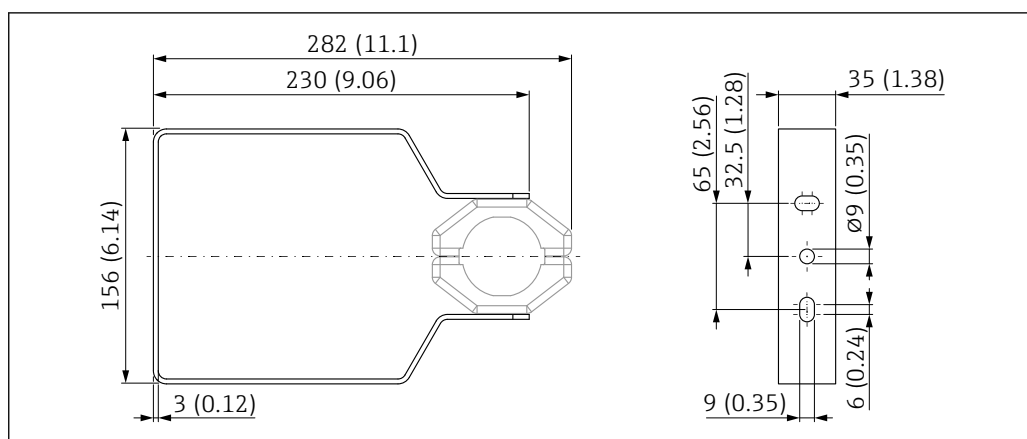
図 42 寸法；調整可能な取付ブラケット FMR6xB。測定単位 mm (in)
