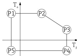
■ 17 SUS 316L 相当製ハウジング、サニタリ仕様 ; プロセス温度 -40\sim+80\text{ }^{\circ}\text{C} ( -40\sim+176\text{ }^{\circ}\text{F} )
