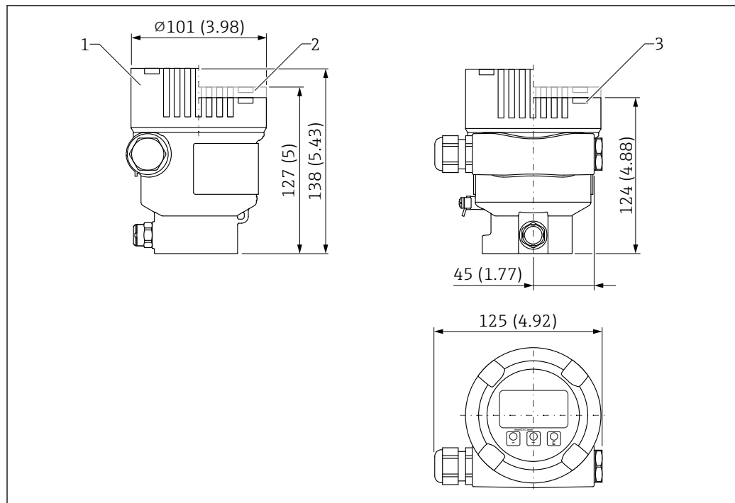
図 20 寸法 ; シングルコンパートメントハウジング (アルミニウム、コーティング) ; M20 カップリングおよびプラグ (プラスチック) 付き。測定単位 mm (in)
