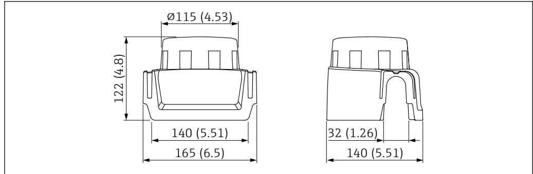
图 69 塑料防护罩 XW111 的外形尺寸示意图。测量单位 mm (in)
