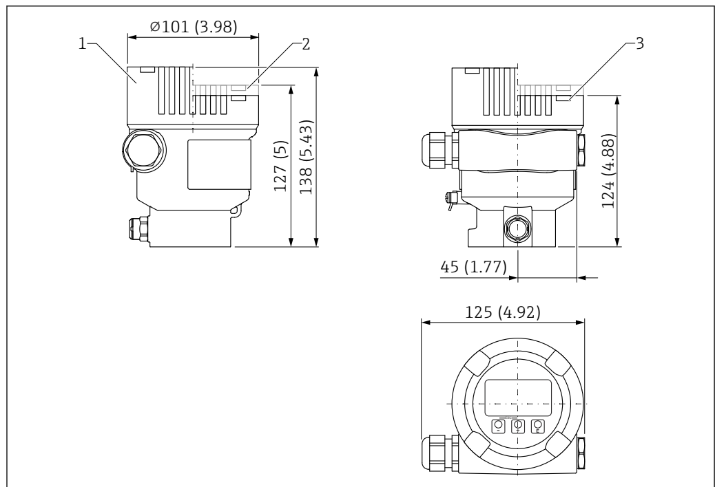
图 53 单腔室铝外壳（带涂层）的外形尺寸示意图；包括 M20 接头和塑料插头。测量单位 mm (in)
