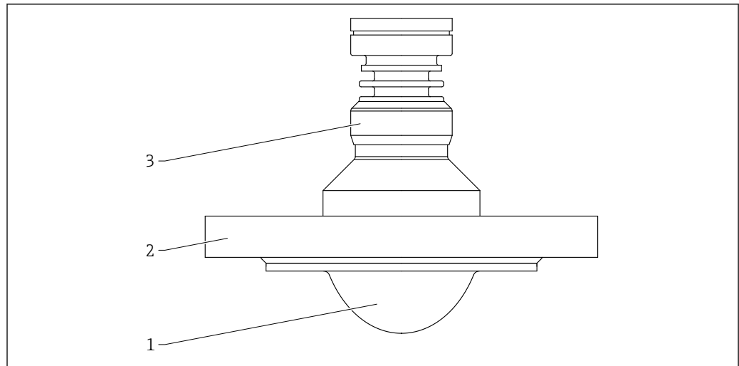
图 65 PTFE 涂层天线（齐平安装，80 mm (3 in)口径）的材质；带法兰
