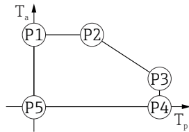
■ 15 プラスチックハウジング ; プロセス温度 0\sim+150\text{ }^{\circ}\text{C} ( +32\sim+302\text{ }^{\circ}\text{F} )、CSA C/US 認定取得
