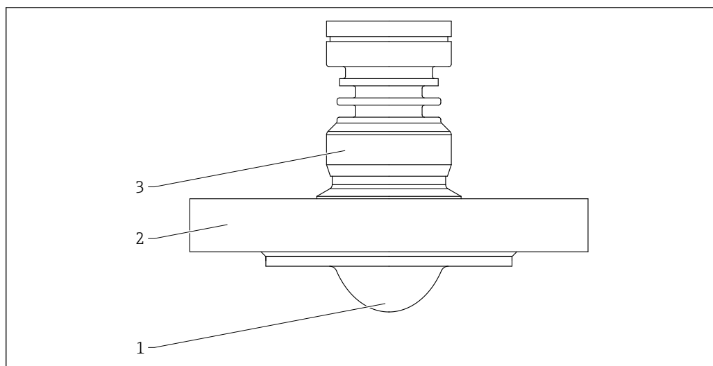
☑ 64 材質 ; PTFE 外装付フラッシュマウントアンテナ、50 mm (2 in)、フランジ付き
