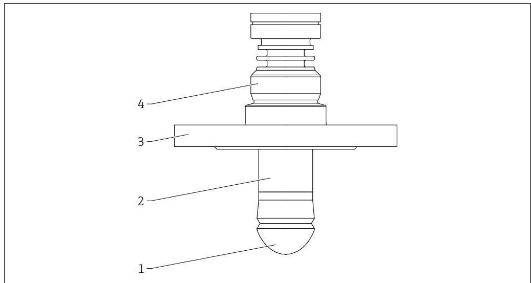
図 63 材質 ; ドリップオフアンテナ
