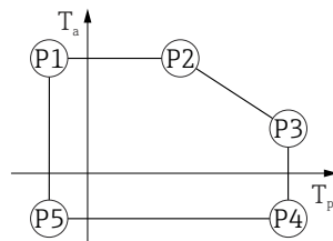
☐ 49 SUS 316L 相当製ハウジング、サニタリ仕様；プロセス温度 -40~+200 °C (-40~+392 °F)
