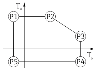
■ 16 プラスチックハウジング ; プロセス温度 -20\sim+200\text{ }^{\circ}\text{C} ( -4\sim+392\text{ }^{\circ}\text{F} )
