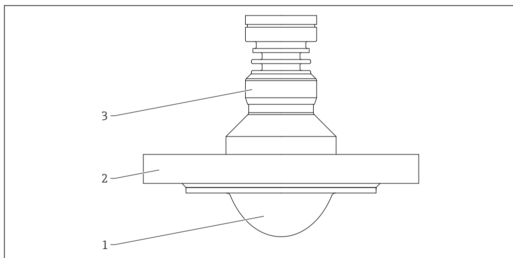
☑ 65 材質 ; PTFE 外装付フラッシュマウントアンテナ、80 mm (3 in)、フランジ付き
