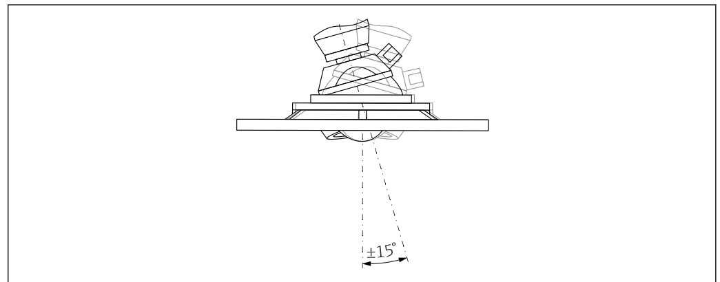
图 10 天线 (齐平安装)，带天线角度调节装置
