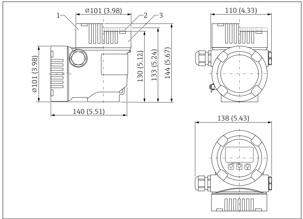
图 40 L型双腔室铝外壳（带涂层）的外形尺寸示意图；包括 M20 接头和塑料插头。测量单位 mm (in)
