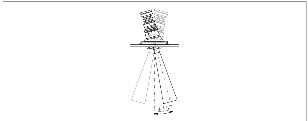
图 9 喇叭天线，带天线角度调节装置
