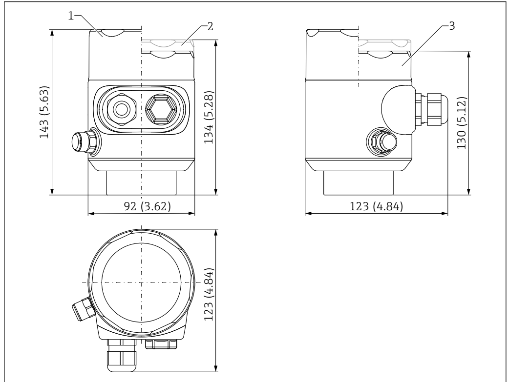
图 38 316L 单腔室外壳（卫生型）的外形尺寸示意图；包括 M20 接头和塑料插头。测量单位 mm (in)
