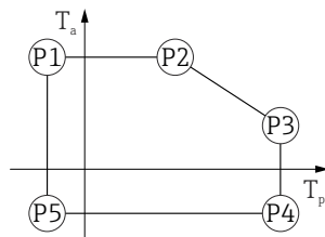
☑ 23 铝外壳, 带涂层; 过程温度范围: -40 ... +80 °C (-40 ... +176 °F)
