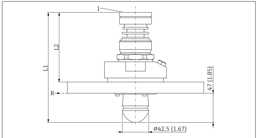
48 PTFE 水滴型天线 (50 mm (2 in)口径) 的外形尺寸示意图; 带 UNI 法兰和空气吹扫接口。测量单位 mm (in)
