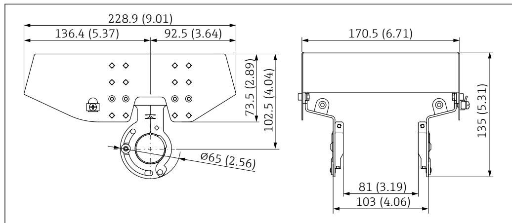
图 70 316L 防护罩 XW112 的外形尺寸示意图。测量单位 mm (in)
