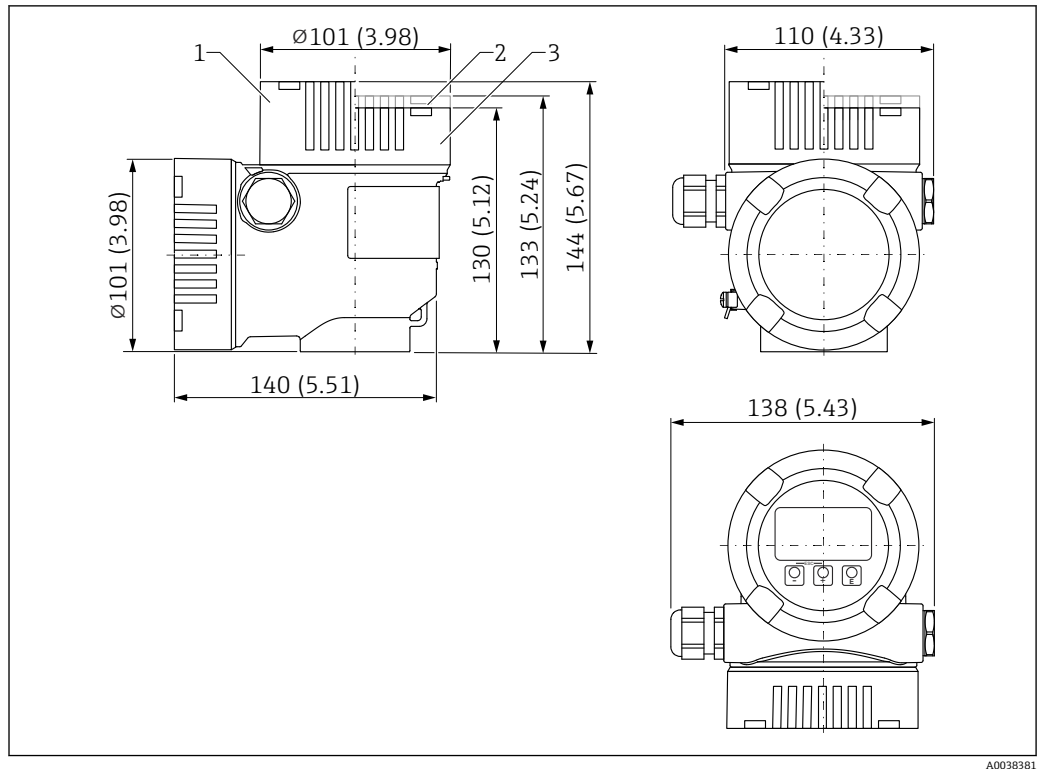
图 41 L 型双腔室 316L 外壳的外形尺寸示意图；包括 M20 接头和塑料插头。测量单位 mm (in)
