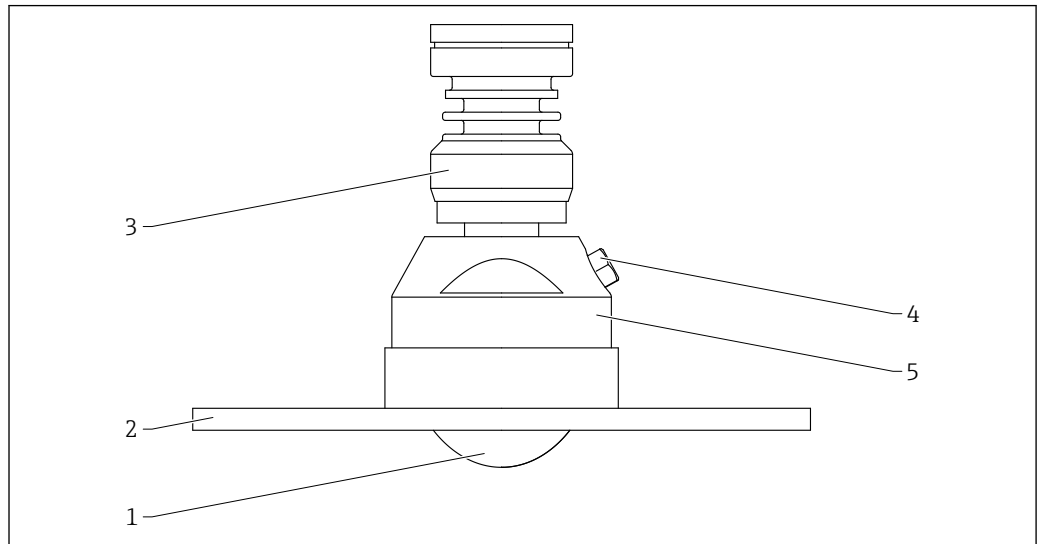
图 65 天线（齐平安装，80 mm (3 in)口径）的材质，带 UNI 法兰和空气吹扫接口。测量单位 mm (in)
