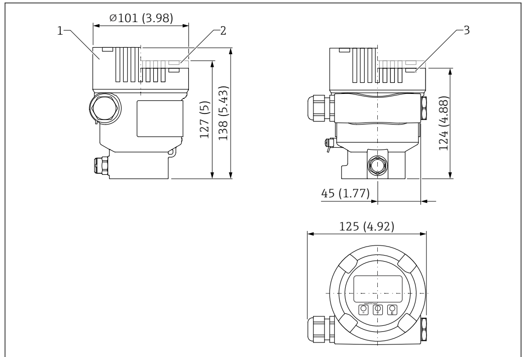
图 37 单腔室铝外壳 (带涂层) 的外形尺寸示意图; 包括 M20 接头和塑料插头。测量单位 mm (in)
