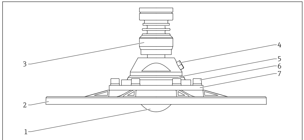
图 66 天线（齐平安装，80 mm (3 in)口径）的材质，带 UNI 法兰、天线角度调节装置和空气吹扫接口
