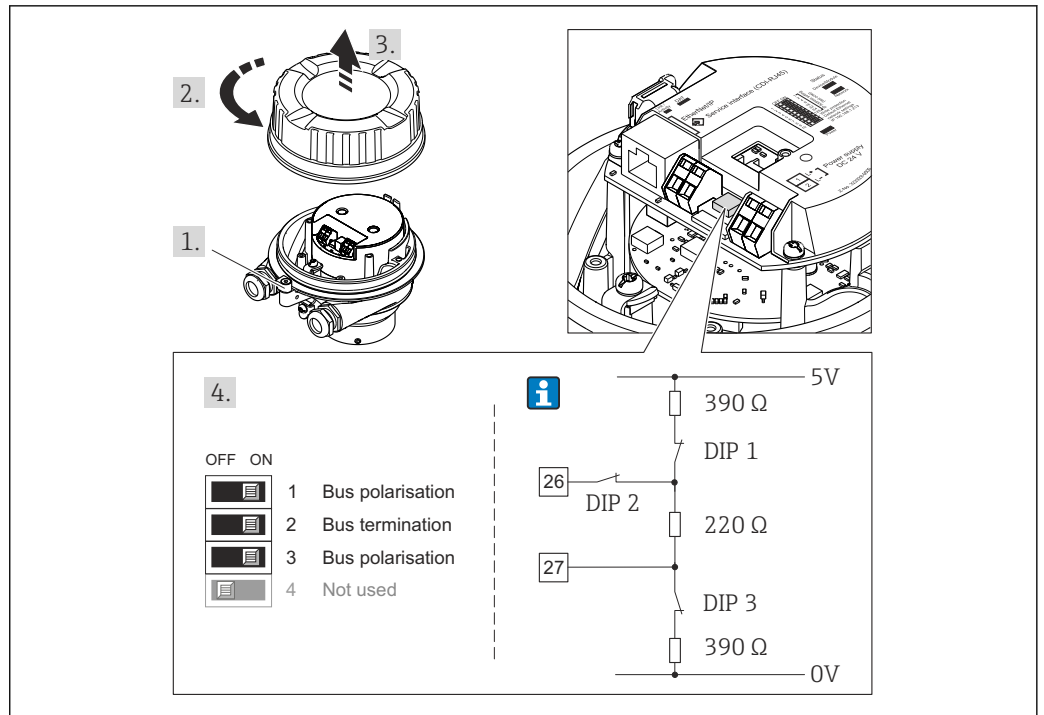
12 Finalização usando minisseletoras no módulo para componentes eletrônicos de E/S (para taxas de transferência < 1.5 Mbaud)
