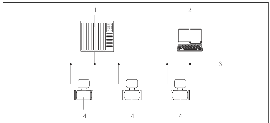
18 Opções para operação remota através da rede PROFIBUS DP
