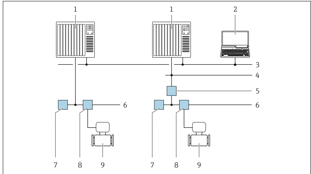
图 13 通过 FOUNDATION Fieldbus 网络进行远程操作
