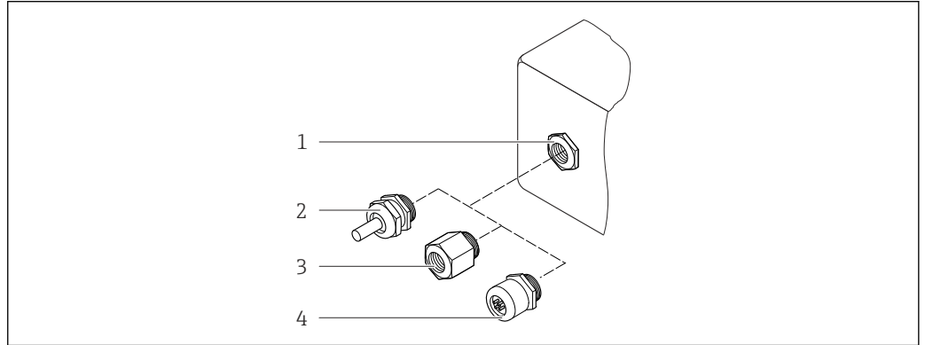
图 24 允许的电缆入口/缆塞
