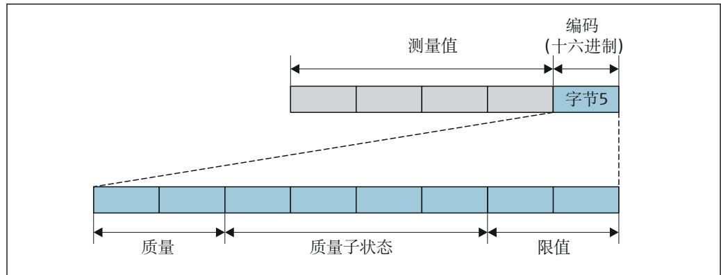
图 20 编码字节结构
