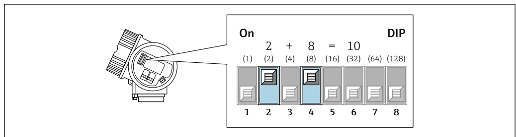
图 11 接线腔中的地址开关示意图; 将设备地址设置为 10
