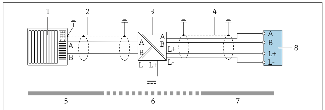
图 14 接线实例: 本安 Modbus RS485
