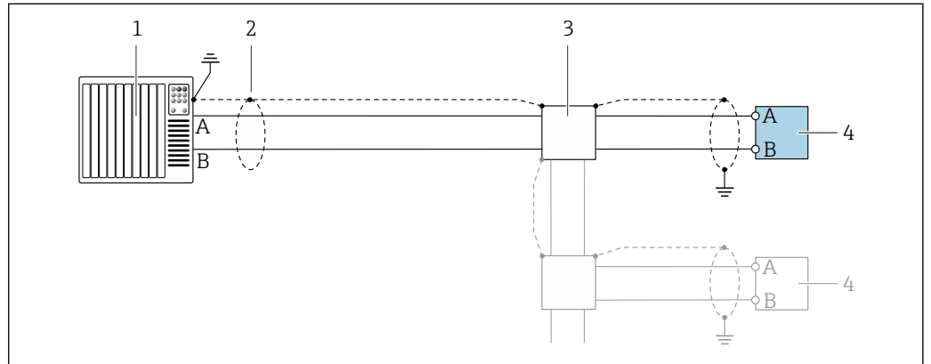
图 13 接线实例, Modbus RS485, 非防爆危险区和 Zone 2 / Div. 2 防爆危险区
