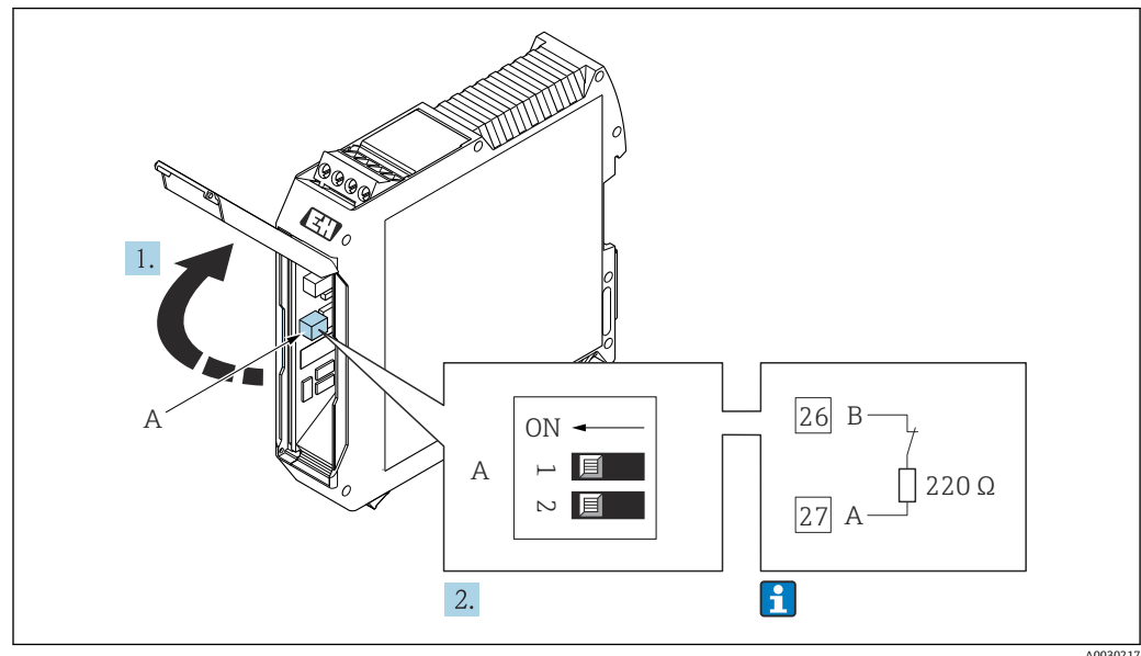
图 16 通过 Promass 100 安全栅上的 DIP 开关开启终端电阻
