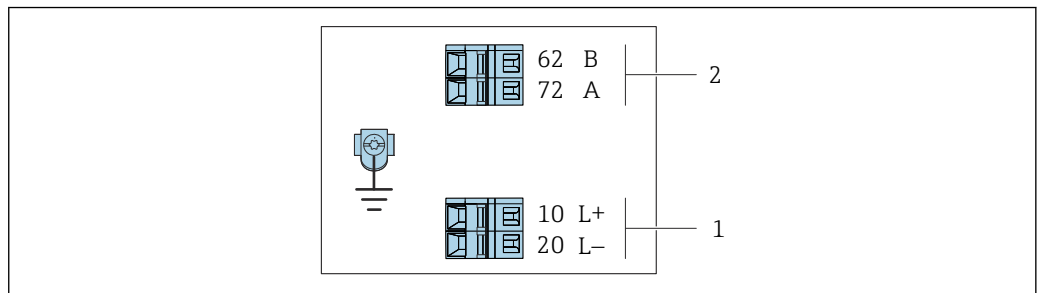
图 8 接线端子分配: Modbus RS485, 在本安防爆区中使用 (通过 Promass 100 安全栅连接)
