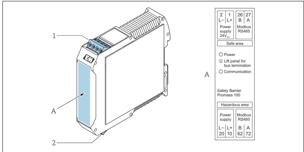
图 9 Promass 100 安全栅, 带接线端子
