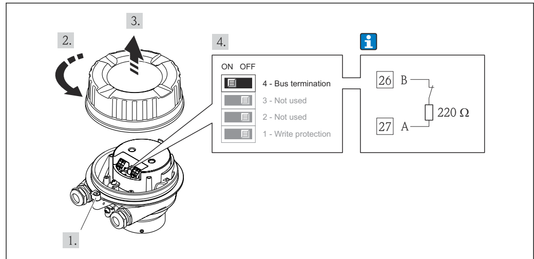
图 15 通过电子模块上的 DIP 开关开启终端电阻
