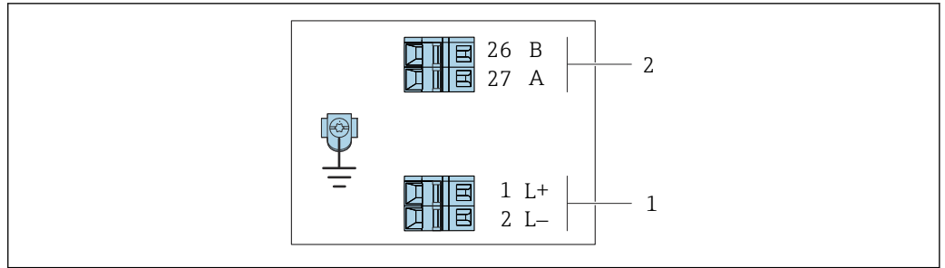
图 7 Modbus RS485 接线端子分配，连接类型适用非危险区和 Zone 2/ Div. 2 防爆场合
