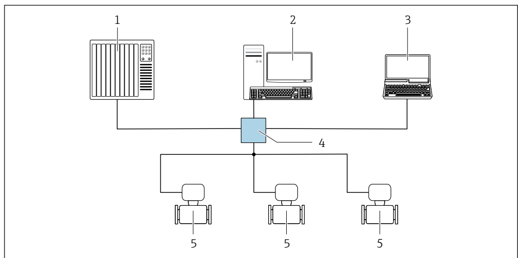
11 Options pour la configuration à distance via le réseau EtherNet/IP : topologie en étoile
