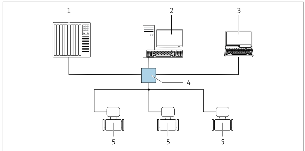
14 Options pour la configuration à distance via le réseau EtherNet/IP : topologie en étoile
