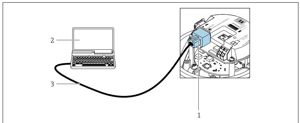
15 Raccordement pour caractéristique de commande "Sortie", option N : EtherNet/IP
