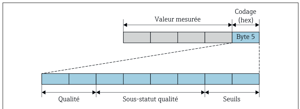
15 Structure de l'octet de codage
