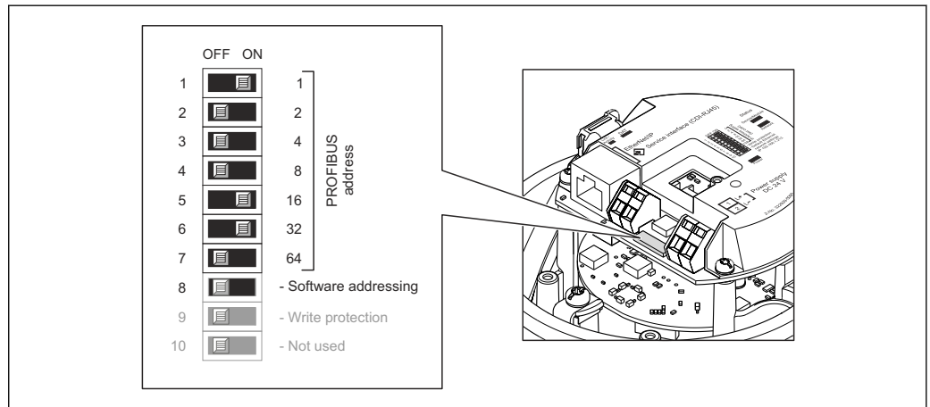
10 Adressage à l'aide des commutateurs DIP sur le module électronique E/S
