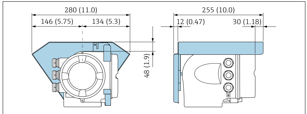
6 Unité de mesure mm (in)
