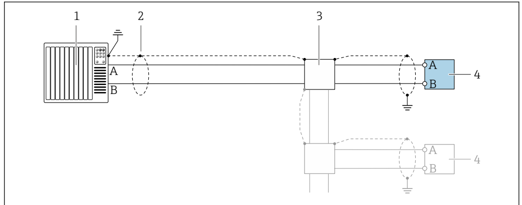
10 Exemple de raccordement pour Modbus RS485, zone non explosible et Zone 2 ; Class I, Division 2
