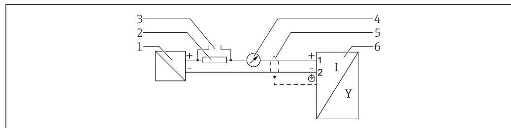
図 11 機能図 4~20 mA HART
