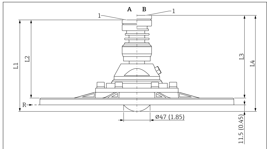
図 64 フラッシュマウントアンテナ (80 mm (3 in)、UNI フランジ/角度調節器/エアージャコネクション付き) の寸法。測定単位 mm (in)
