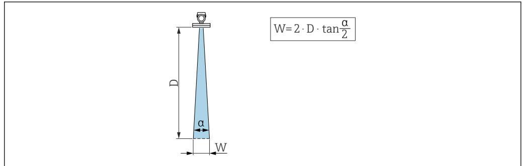
20 ビーム放射角 \alpha 、距離 D 、ビーム幅 W の関係
