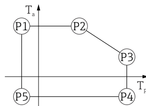
図 21 プラスチックハウジング ; プロセス温度 -40~+80 °C (-40~+176 °F)
