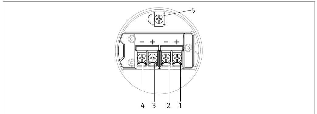
図 5 端子部の端子の割当て ; 4~20 mA HART + 4~20 mA アナログ ; デュアルコンパートメントハウジング
