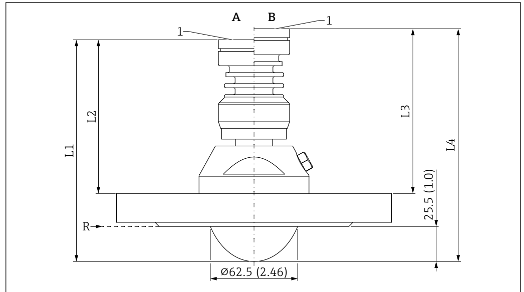
図 60 フラッシュマウントアンテナ (PTFE、80 mm (3 in)、標準フランジおよびエアージャコネクション付き) の寸法。測定単位 mm (in)
