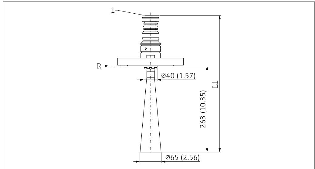
図 50 DN65 ホーンアンテナ - フランジプロセス接続の寸法。測定単位 mm (in)
