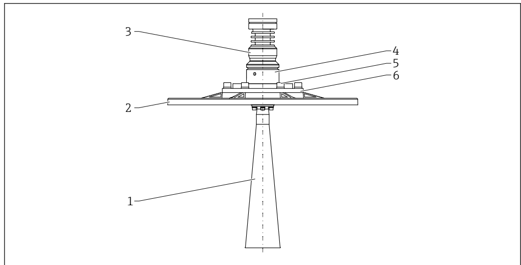
図 70 材質 ; 65 mm (2.6 in) ホーンアンテナ、UNI フランジおよび角度調節器付き。測定単位 mm (in)
