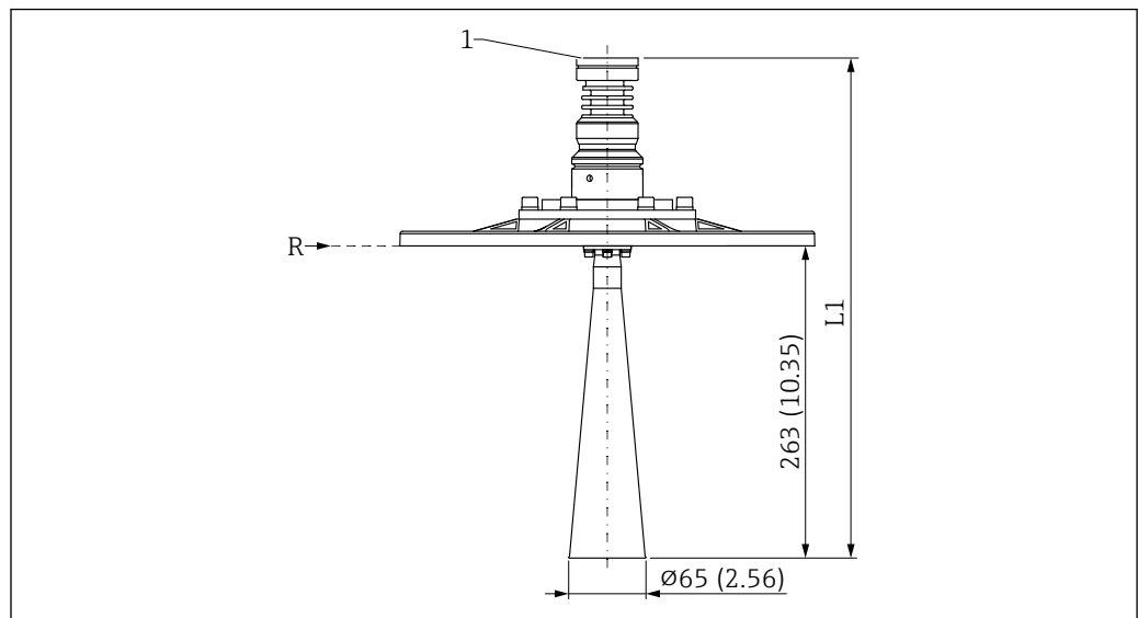
図 51 DN65 ホーンアンテナ（UNI フランジおよび角度調節器付き）の寸法。測定単位 mm (in)
