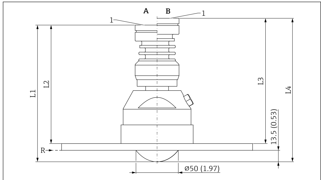
図 61 フラッシュマウントアンテナ (PTFE、80 mm (3 in)、UNI フランジおよびエアージャコネクション付き) の寸法。測定単位 mm (in)
