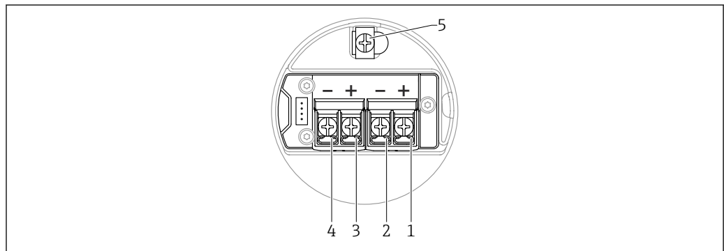
図 8 端子部の端子の割当て ; 4~20 mA HART + 4~20 mA アナログ ; デュアルコンパートメントハウジング L 字型
