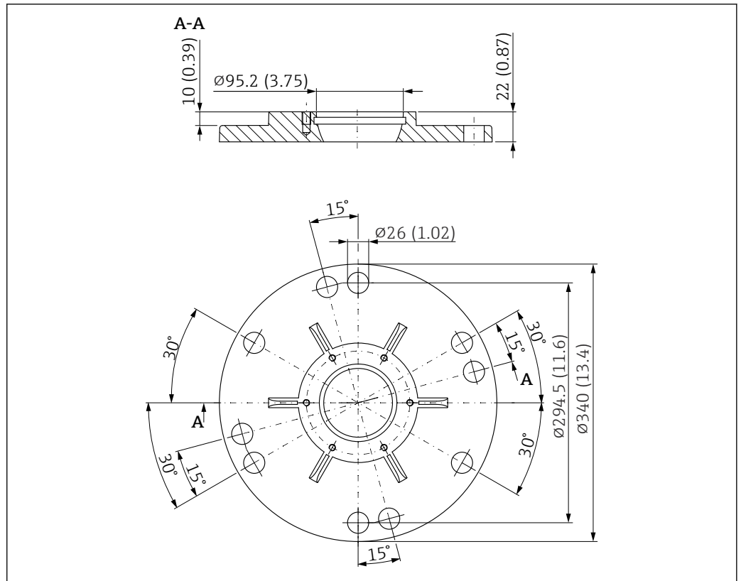
図 67 UNI フランジ 8"/DN200/200A (角度調節器付きアンテナ用) の寸法。測定単位 mm (in)
