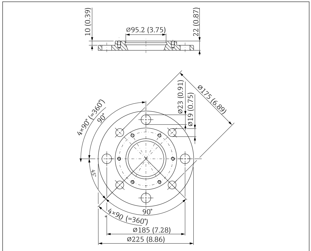
図 52 UNI フランジ UNI 4"/DN100/100A (角度調節器付きアンテナ用) の寸法。測定単位 mm (in)
