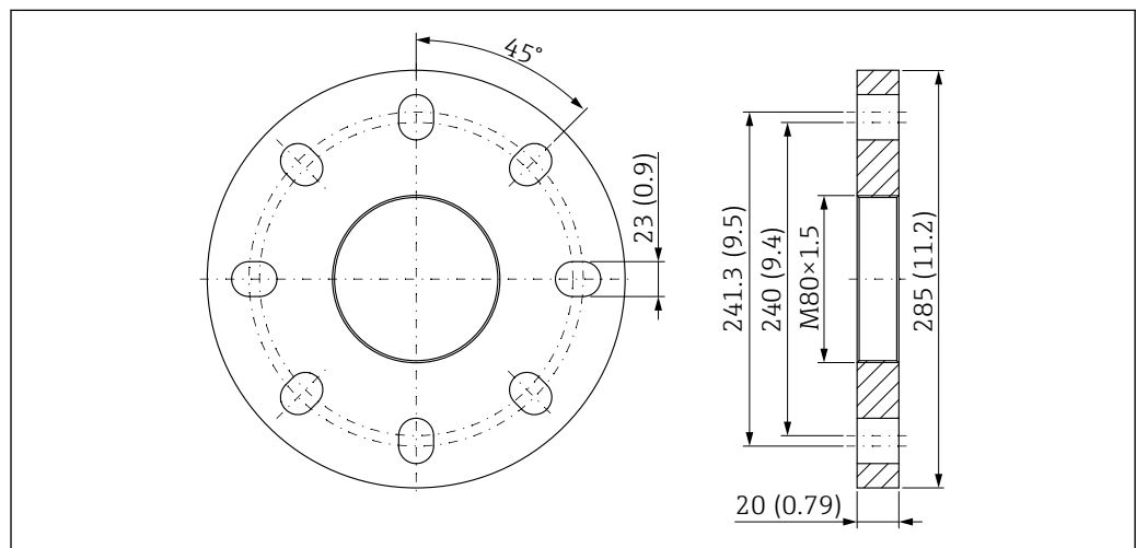
図 59 UNI フランジ 6"/DN150/150A (ドリップオフアンテナ (PTFE、50 mm (2 in)、エアージャコネクション付き) 用)。測定単位 mm (in)
