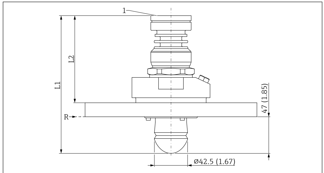
■ 56 ドリッポフアンテナ (PTFE、50 mm (2 in)、UNI フランジおよびエアパージコネクション付き) の寸法。測定単位 mm (in)
