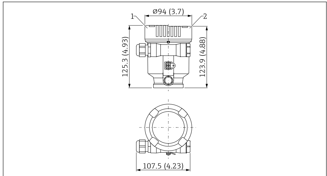
図 44 寸法；シングルコンパートメントハウジング（プラスチック）；M20 カップリングおよびプラグ（プラスチック）付き。測定単位 mm (in)
