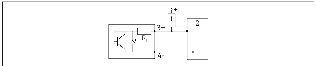
図 14 デジタル入力の接続例
