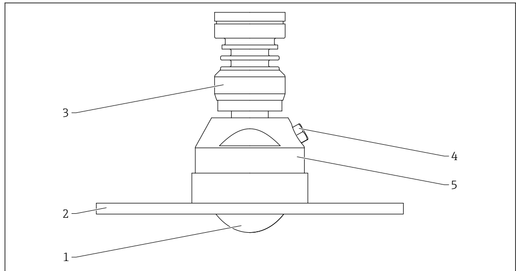
図 73 材質 ; アンテナ、フラッシュマウント、80 mm (3 in)、UNI フランジおよびパージエア接続付き。測定単位 mm (in)
