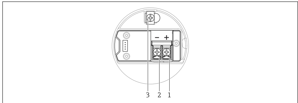
図 7 端子部の端子の割当て ; 4~20 mA HART ; デュアルコンパートメントハウジング L 字型
