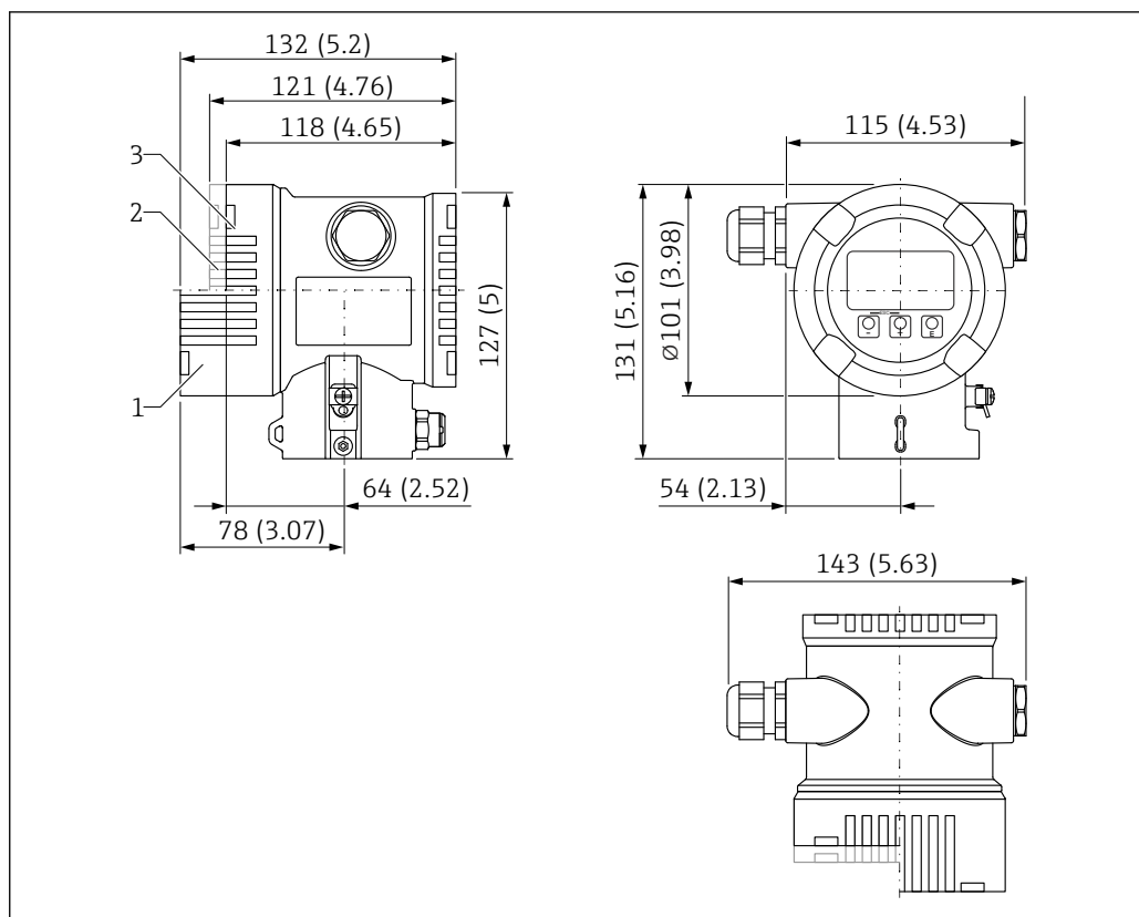
図 47 寸法；デュアルコンパートメントハウジング（アルミニウム、コーティング）；M20 カップリングおよびプラグ（プラスチック）付き。測定単位 mm (in)
