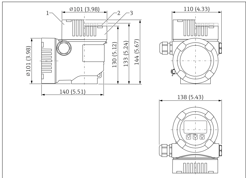
図 48 寸法 ; デュアルコンパートメントハウジング L 字型 (アルミニウム、コーティング) ; M20 カップリングおよびプラグ (プラスチック) 付き。測定単位 mm (in)
