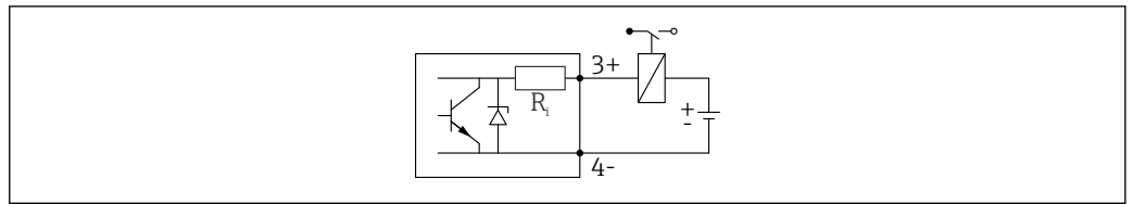
図 13 リレーの接続例
