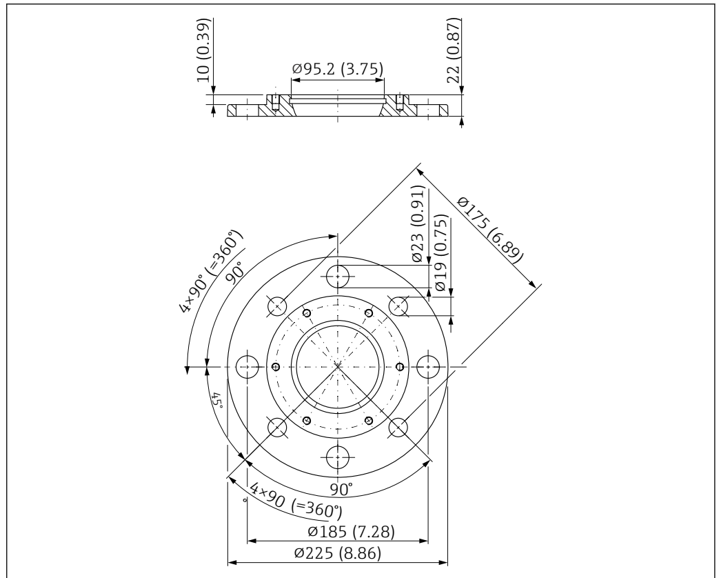
図 65 UNI フランジ UNI 4"/DN100/100A (角度調節器付きアンテナ用) の寸法。測定単位 mm (in)
