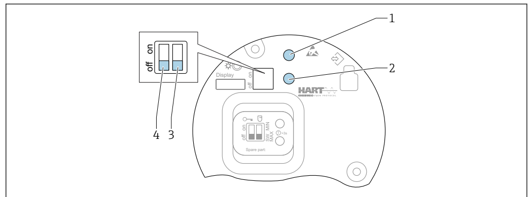
図 75 HART エレクトロニクインサート上の操作キーおよび DIP スイッチ
