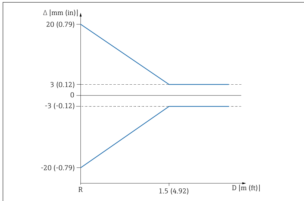
図 16 近範囲アプリケーションにおける最大測定誤差
