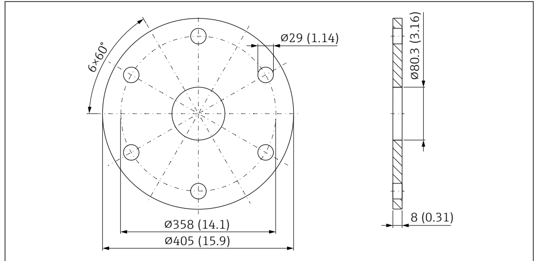
図 63 UNI フランジ 10"/DN250/250A (エアーパージコネクション付き DN80 アンテナ用) の寸法。測定単位 mm (in)
