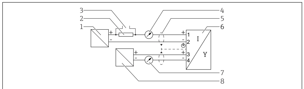
図 15 4~20 mA HART + 4~20 mA アナログの機能図
