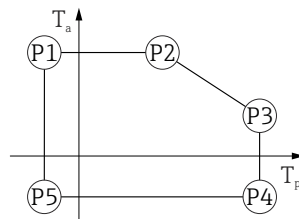
☐ 39 SUS 316L 相当製ハウジング ; プロセス温度 -40 \sim +280 \text{ }^{\circ}\text{C} ( -40 \sim +536 \text{ }^{\circ}\text{F} )
