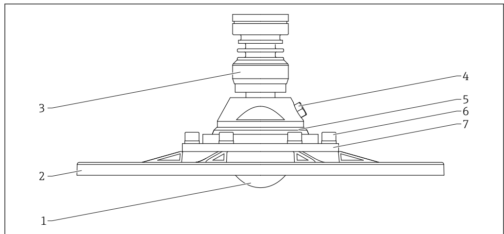
図 74 材質 ; アンテナ、フラッシュマウント、80 mm (3 in)、UNI フランジ/角度調節器/パージエア接続付き
