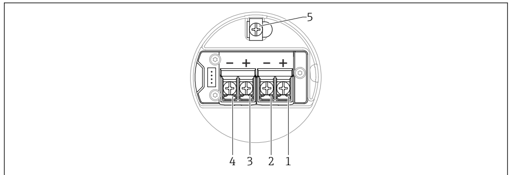
図 9 端子部の端子の割当て ; 4~20 mA HART、スイッチ出力 ; デュアルコンパートメントハウジング L 字型
