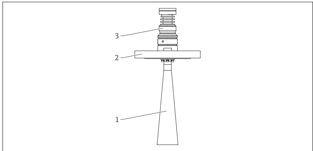
図 69 材質 ; 65 mm (2.6 in) ホーンアンテナ。測定単位 mm (in)
