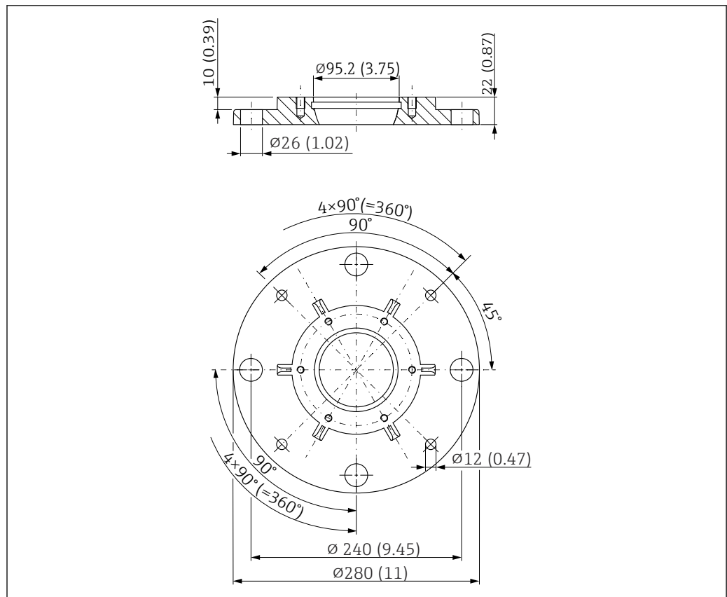
図 53 UNI フランジ 6"/DN150/150A (角度調節器付きアンテナ用) の寸法。測定単位 mm (in)
