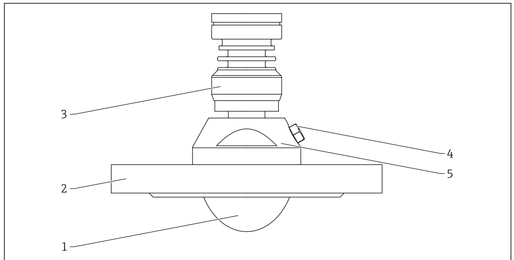
☐ 72 材質；アンテナ、フラッシュマウント、80 mm (3 in)、フランジおよびパージエア接続付き。測定単位 mm (in)
