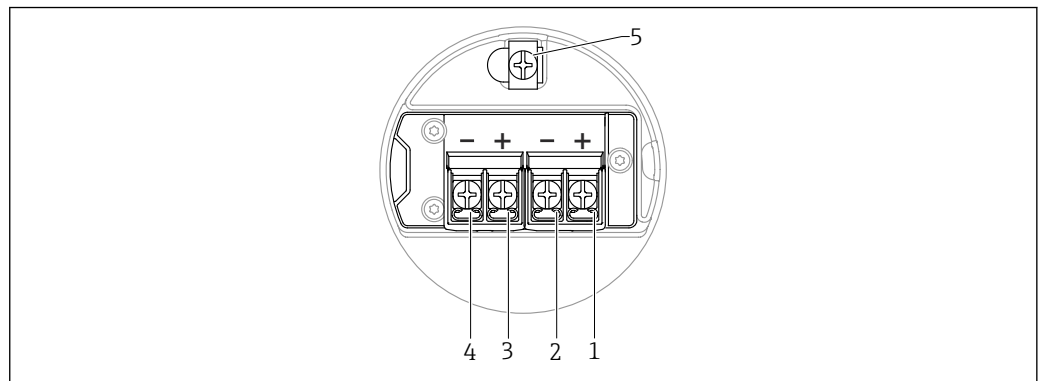
図 6 端子部の端子の割当て ; 4~20 mA HART、スイッチ出力 ; デュアルコンパートメントハウジング
