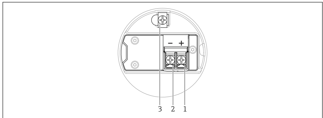
図 4 端子部の端子の割当て；4～20 mA HART；デュアルコンパートメントハウジング
