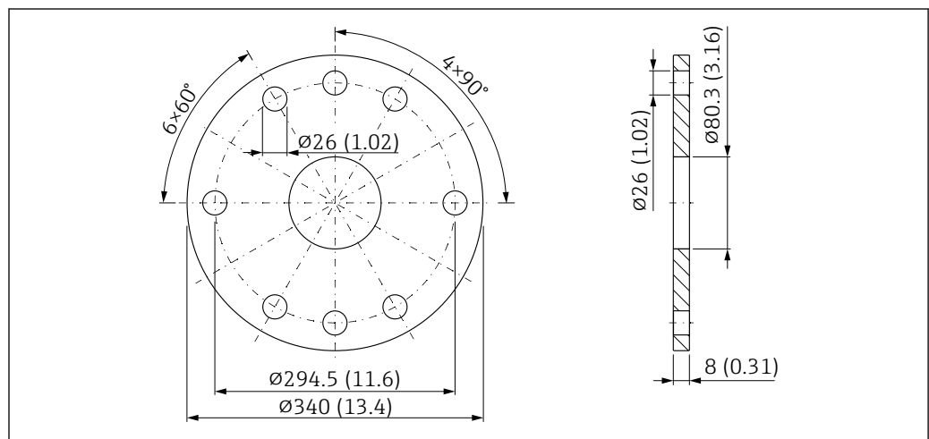
図 62 UNI フランジ 8"/DN200/200A (エアージャコネクション付き DN80 アンテナ用) の寸法。測定単位 mm (in)
