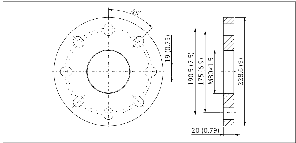
図 58 UNI フランジ 4"/DN100/100A (ドリップオフアンテナ (PTFE、50 mm (2 in)、エアージャコネクション付き) 用)。測定単位 mm (in)
