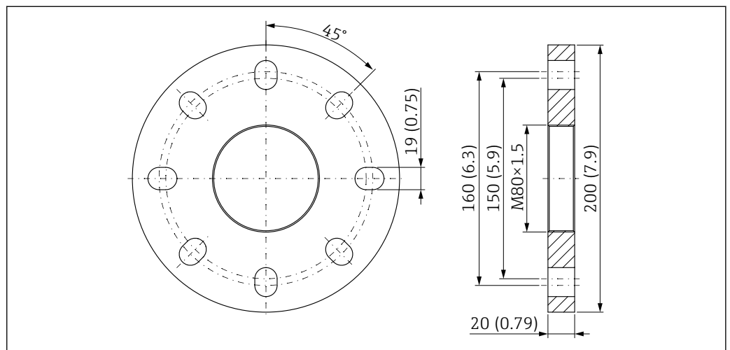
■ 57 UNI フランジ 3"/DN80/80A (ドリッポフアンテナ (PTFE、50 mm (2 in)、エアパージコネクション付き) 用)。測定単位 mm (in)
