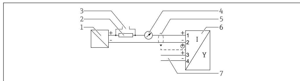
図 12 4~20 mA HART、スイッチ出力の機能図
