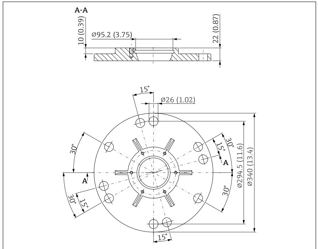
図 54 UNI フランジ 8"/DN200/200A (角度調節器付きアンテナ用) の寸法。測定単位 mm (in)
